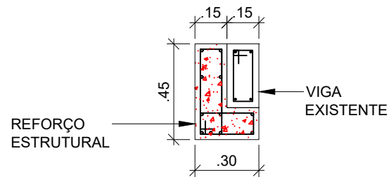
3- REFORÇO DO MURO VIGA INFERIOR ESC. 1/25
