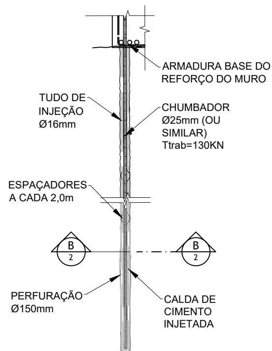
4 - DET. EXECUÇÃO DOS CHUMBADORES ESTACAS COM MONOBARRA SEM ESCALA
