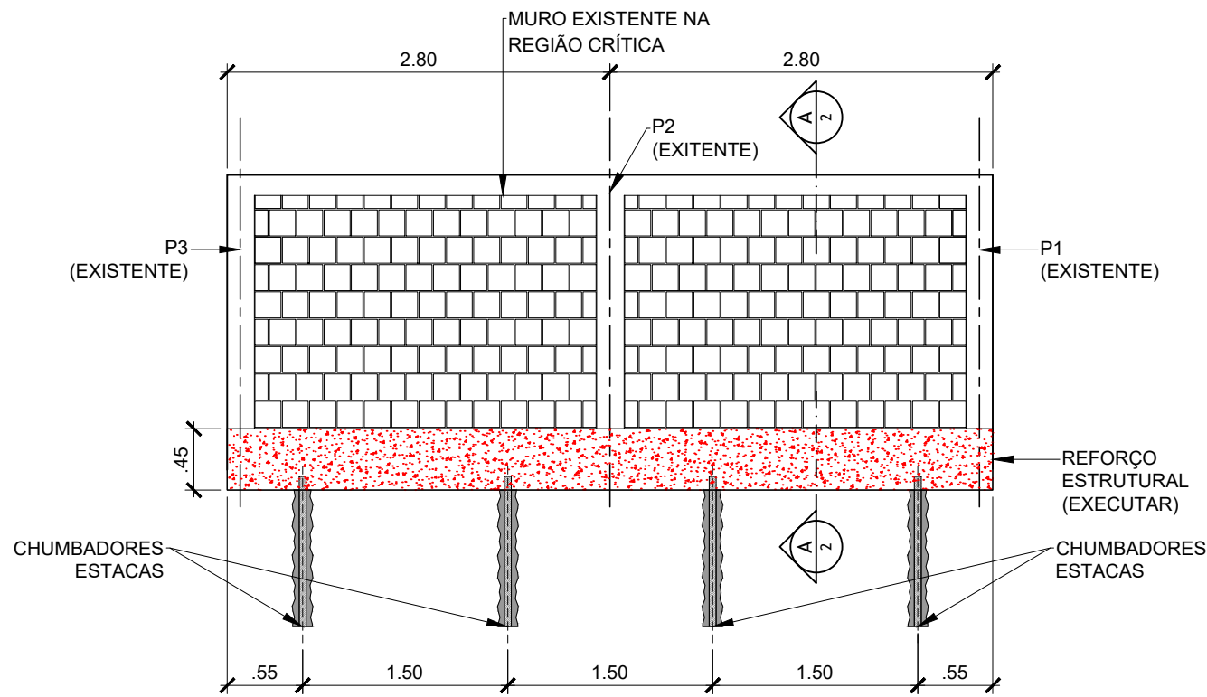
2 - PLANIFICAÇÃO ESC. 1:50
