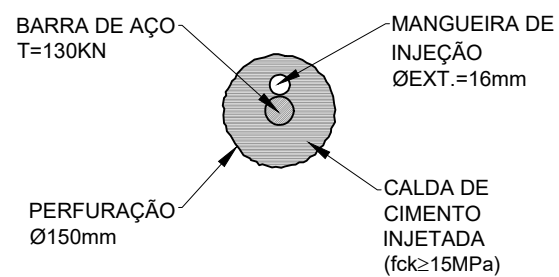
5 - CORTE B-B SEM ESCALA
