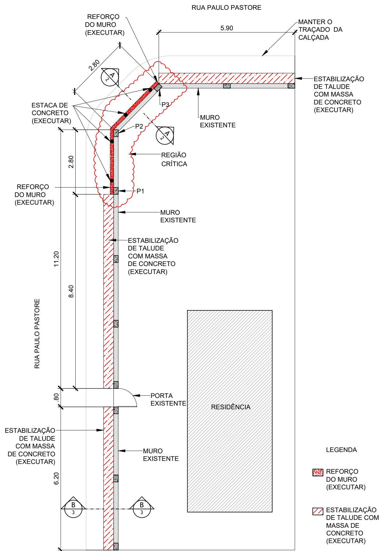
1 - PLANTA DE LOCALIZAÇÃO ESC. 1:100
