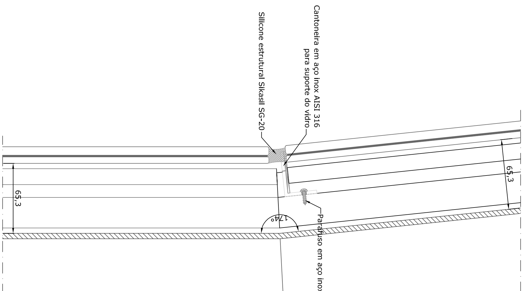
SEV-P10 ESCALA 1:2
