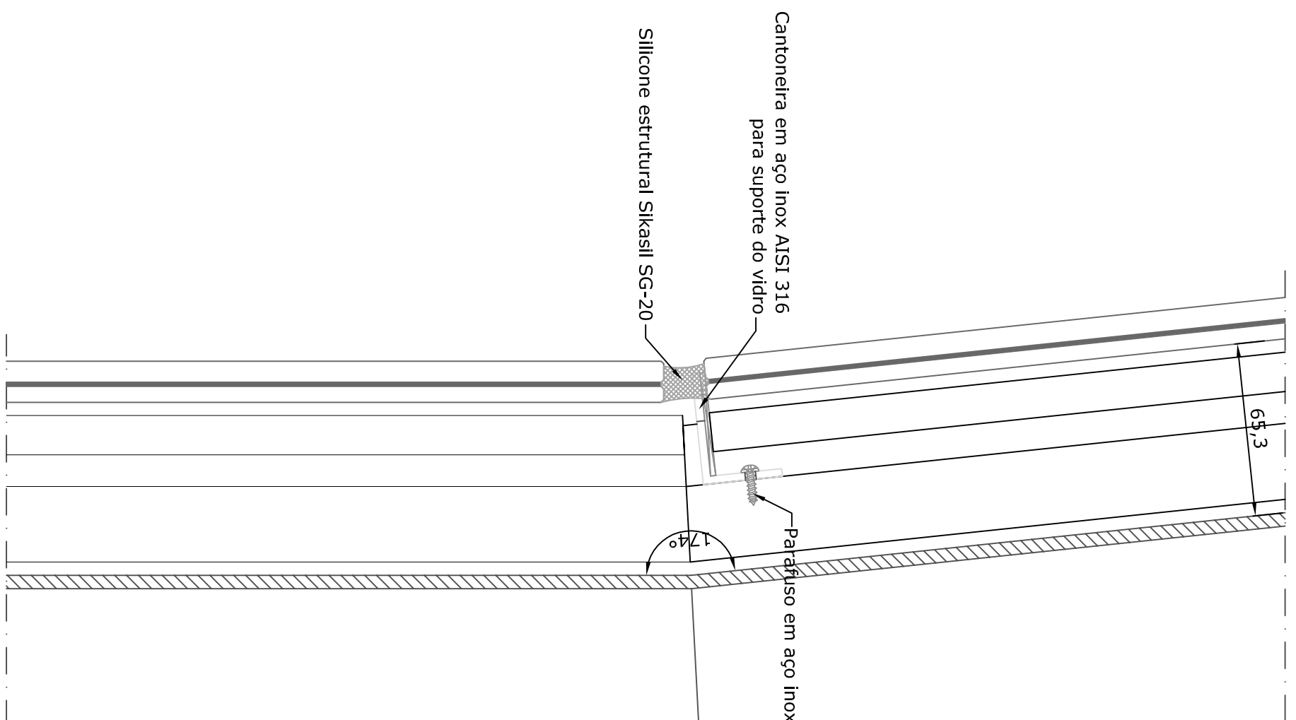
SEV-P13 ESCALA 1:2
