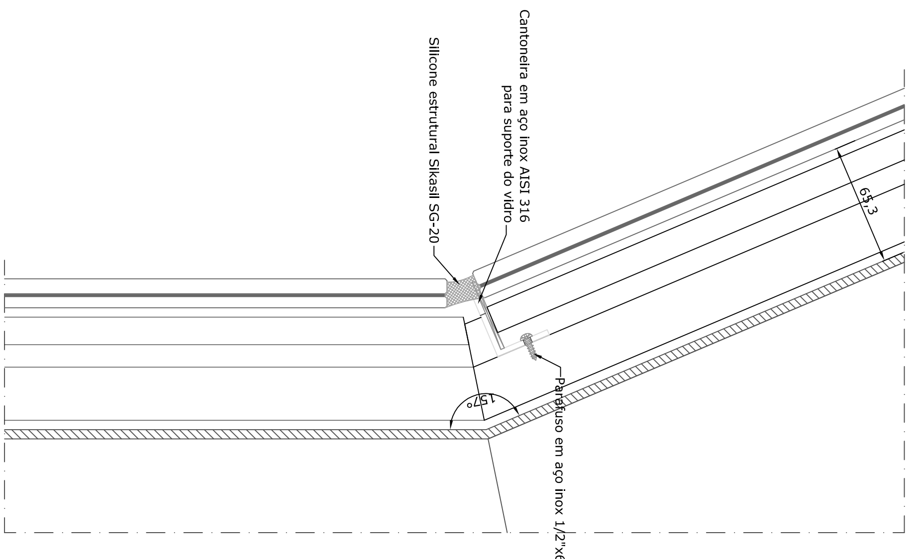
SEV-P11 ESCALA 1:2
