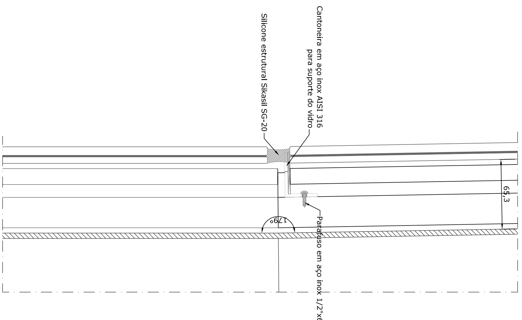
SEV-P12 ESCALA 1:2
