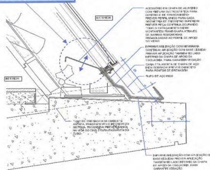
5 DETALHE INFERIOR - EGS 1,2 NA BORDA DE LAJE (10. PAVIMENTO)
