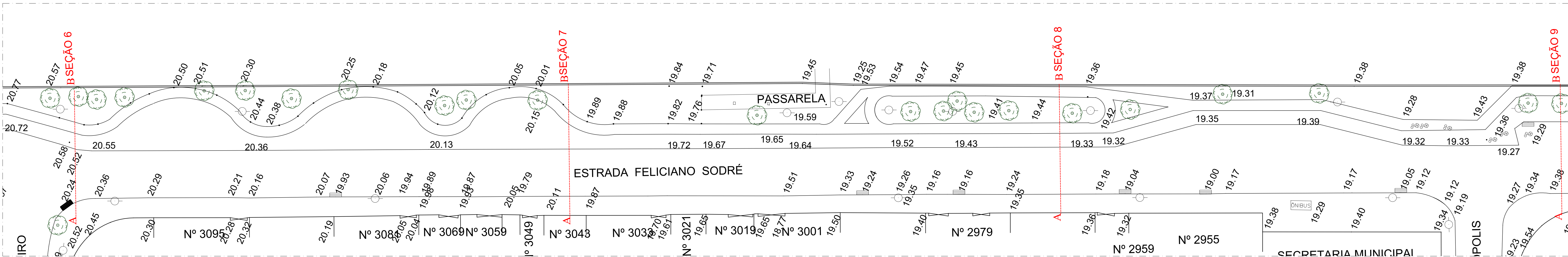
3 TOPOGRAFIA - TRECHO B ESCALA 1:250
