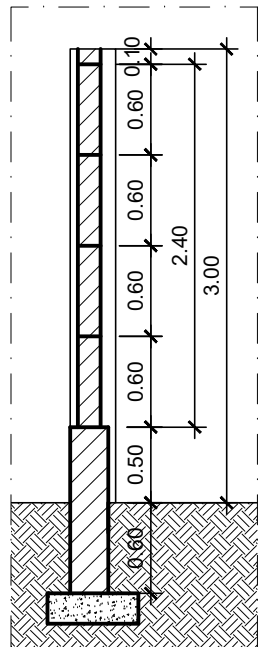
3 CORTE ESCALA 1/50
