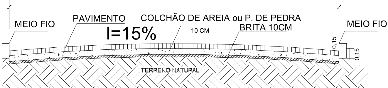
PERFIL TRANSVERSAL - SEM ESCALA
