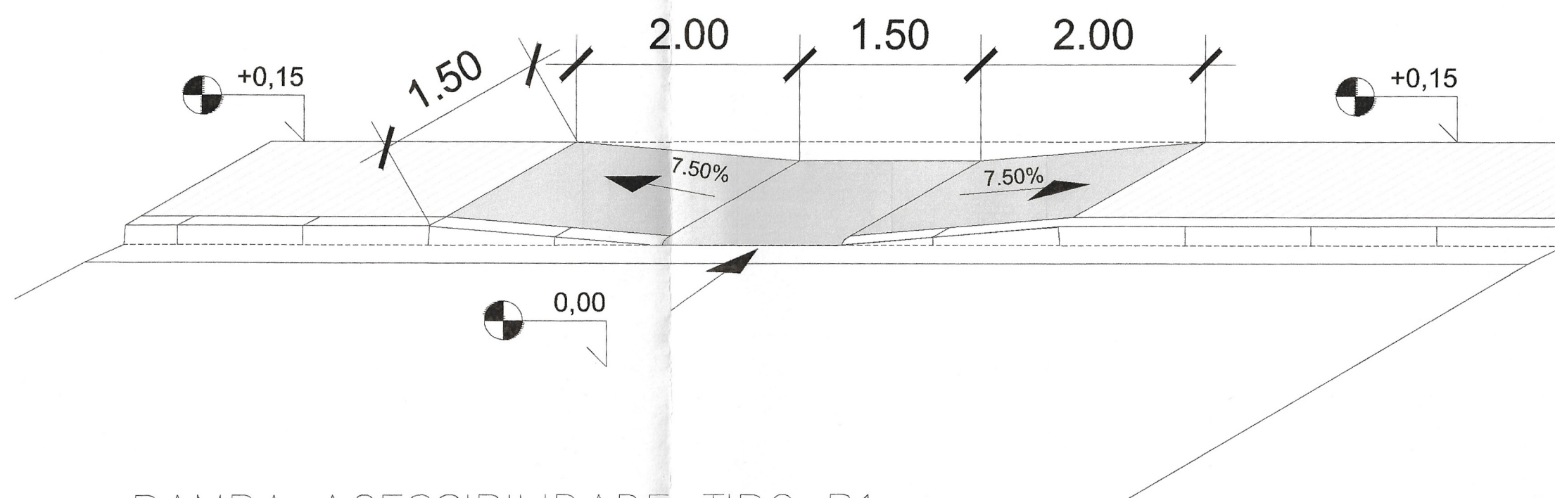
RAMPA ACESSIBILIDADE TIPO R1 VISTA ISOMÉTRICA SEM ESCALA
