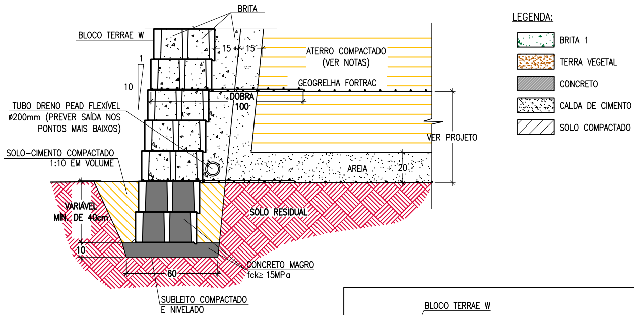
DETALHE DA BASE DO MURO EM SOLO SEM ESC.
