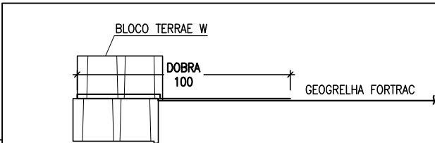
DETALHE DO TRANSPASSE SEM ESC.
