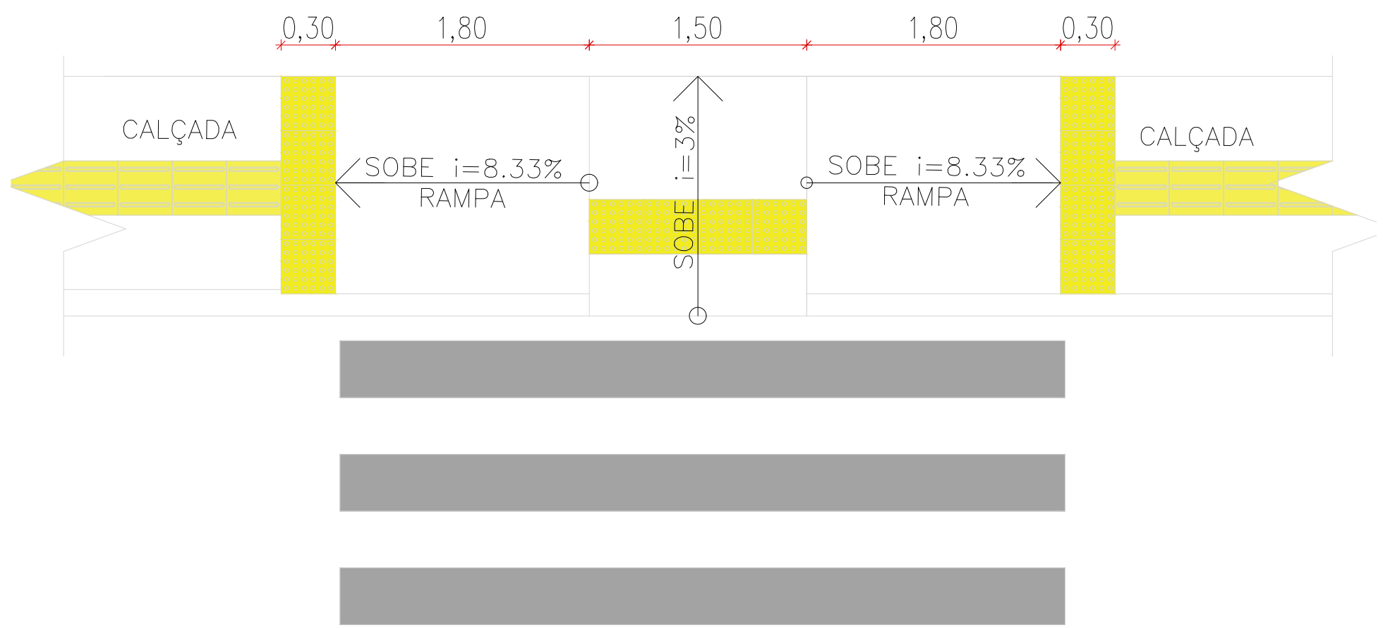
02 DETALHE DAS RAMPAS PARALELAS ÀS VIAS SEM ESCALA
