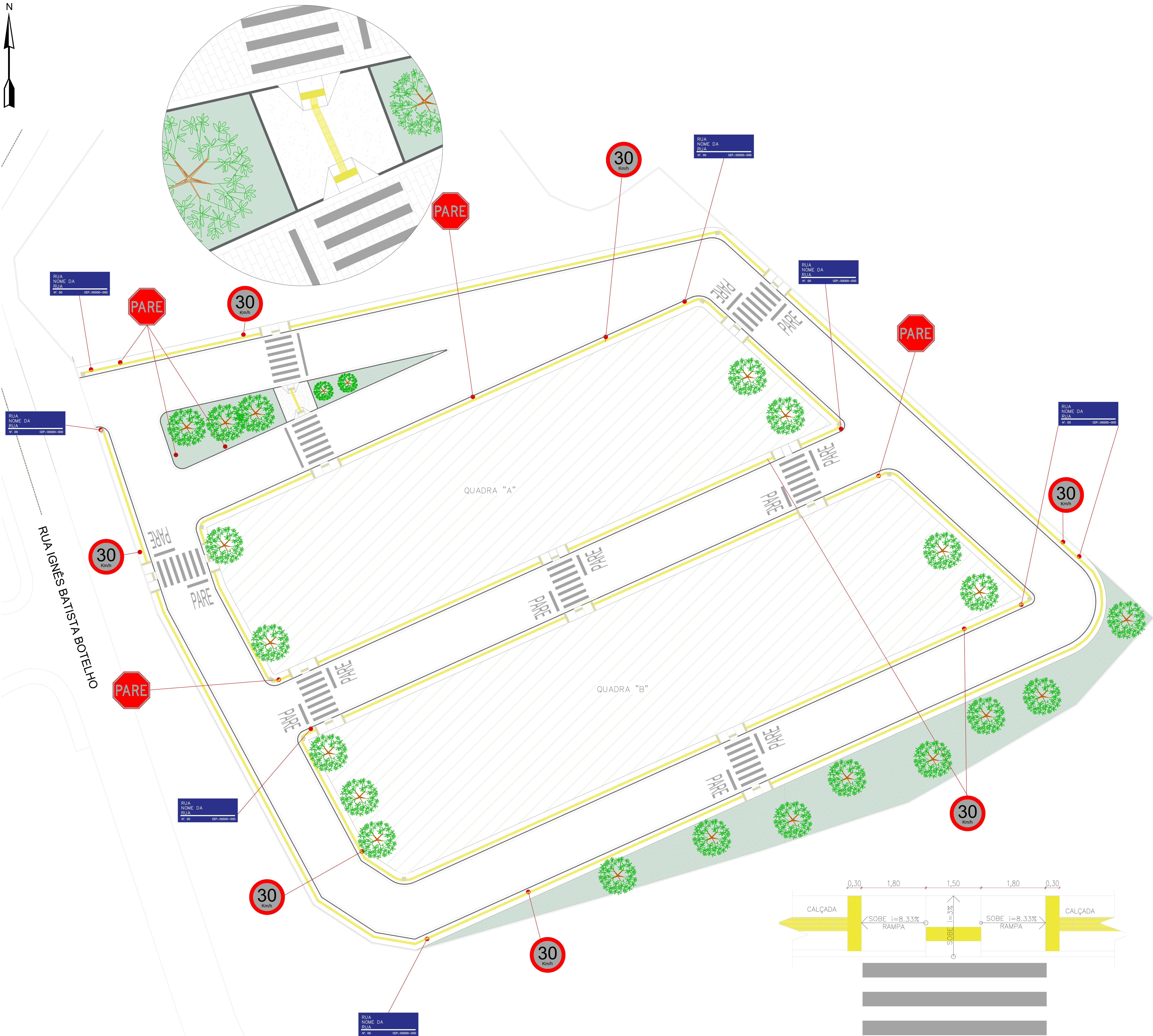
01 PLANTA BAIXA- SINALIZAÇÃO E ACESSIBILIDADE ESC. 1:200
