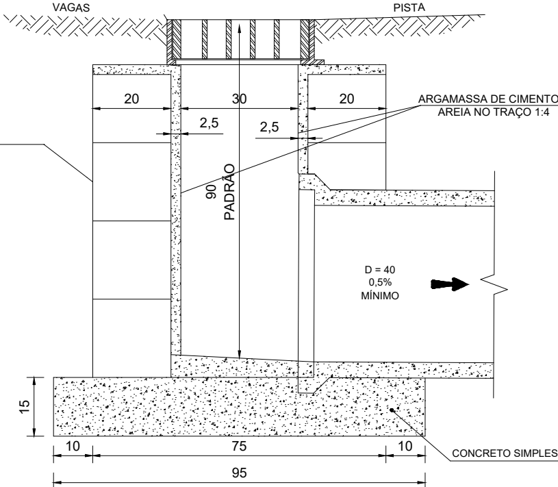
CORTE AA ESCALA - S/ESC
