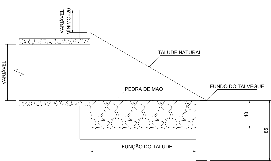
CORTE BB
