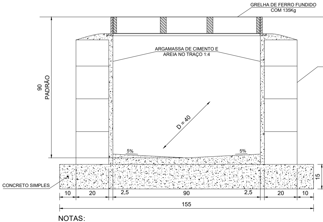
CORTE BB ESCALA - S/ESC
