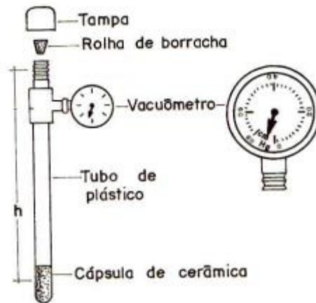
Figura 5. Tensiômetro. Fonte: Silveira e Stone (1994).
