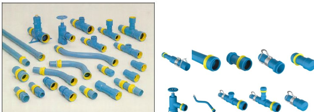
Figura 2. Acessórios para tubulações de PVC com engates rápidos rosqueáveis, alça e bolsa.
