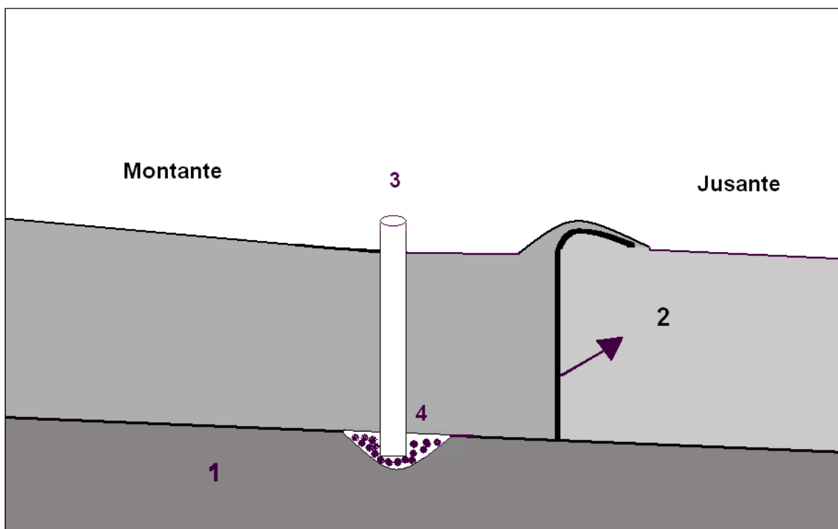
Figura 8: Corte transversal (1 = Camada impermeável; 2 = lona (manta) de polietileno; 3 = poço de manilhas ou tijolos; 4 = fundo do poço envolvido por cascalhos, pedras ou entulho limpo de obra).
