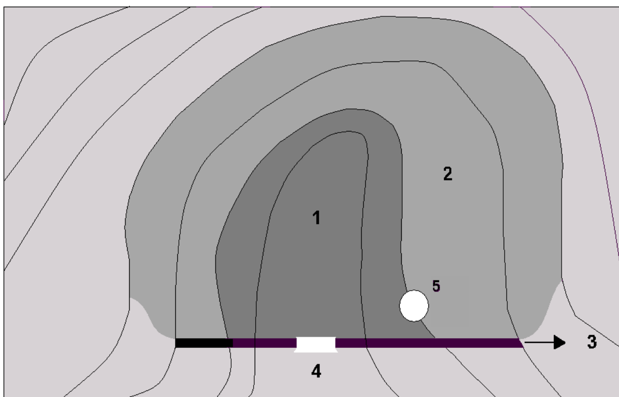
Figura 7: Planta baixa (1 = Área mais baixa, saturada e/ou com água aparente; 2 = Área com água disponível abaixo da superfície; 3 = Barragem subterrânea; 4 = Vertedouro; 5 = Poço).
