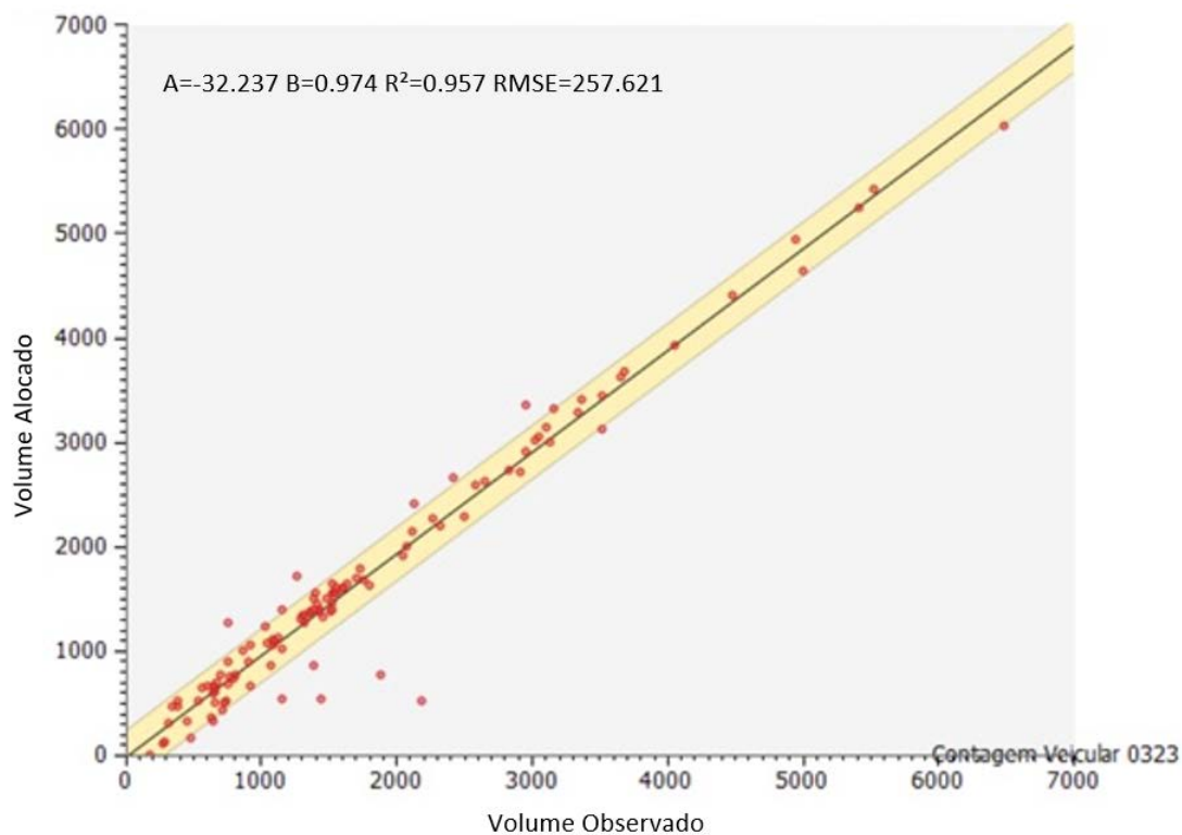
Figura 90: Gráfico do volume alocado x observado para transporte privado
