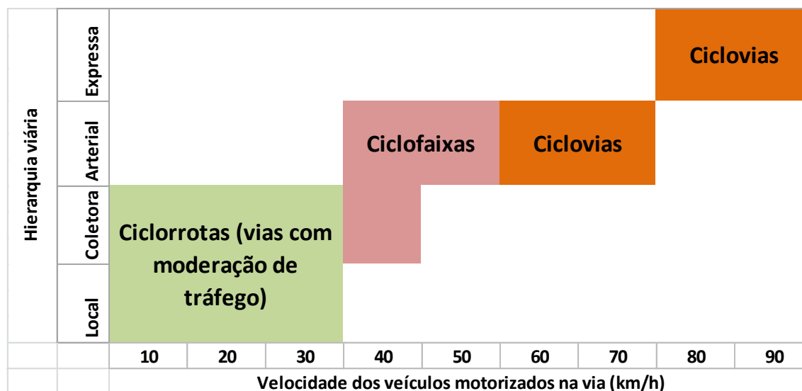
Figura 161: Tipologia de tratamento ciclovitário de acordo com hierarquia viária e velocidade da via
