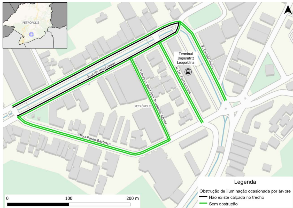
Figura 62: Obstrução de iluminação ocasionada por árvore nas calçadas da rede inventariada de Petrópolis
