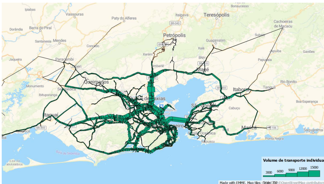
Figura 129: Carregamento de transporte individual nos principais eixos metropolitanos, no cenário de prognóstico
