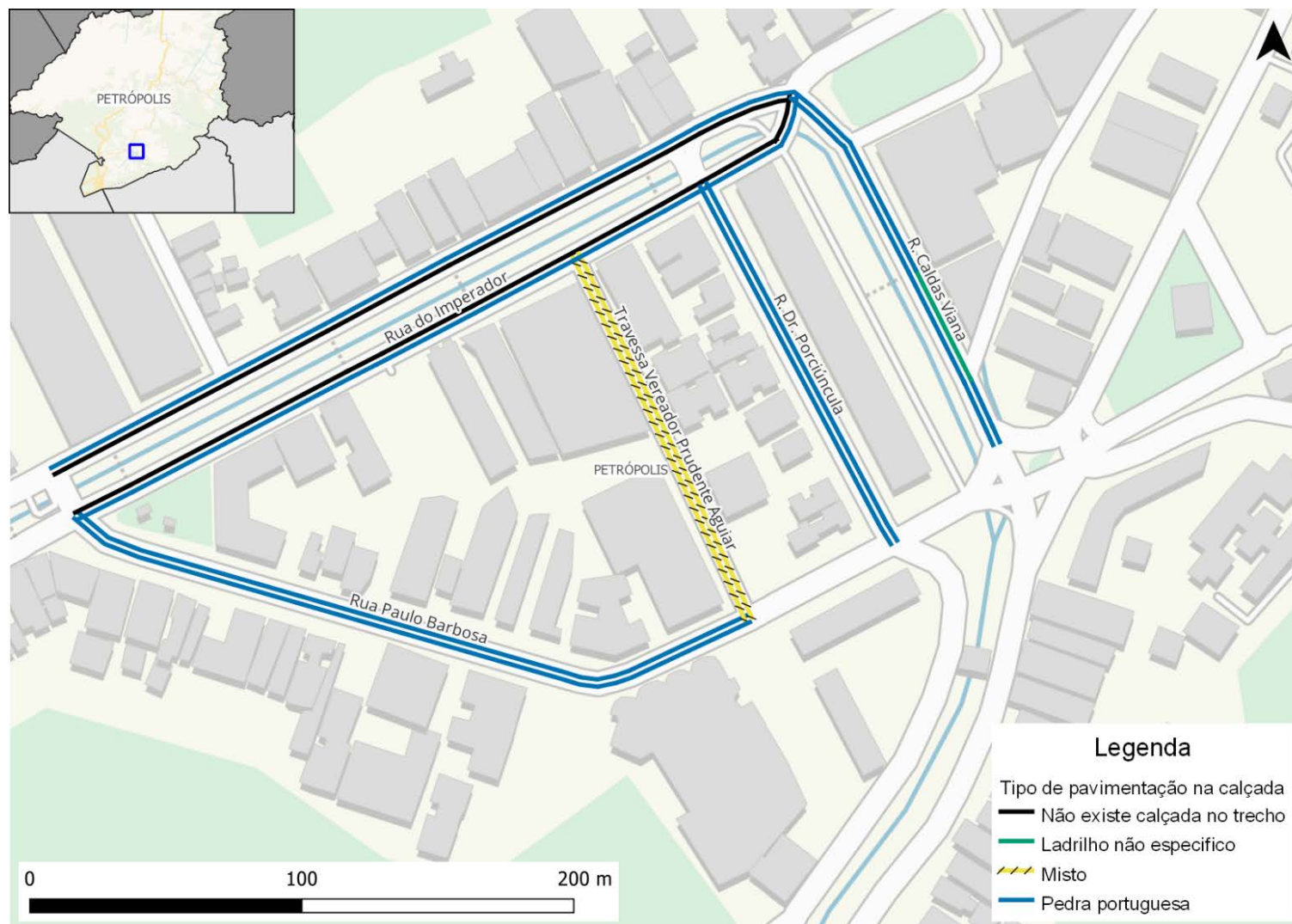
Figura 220: Tipo de pavimentação nas calçadas da rede inventariada de Petrópolis
