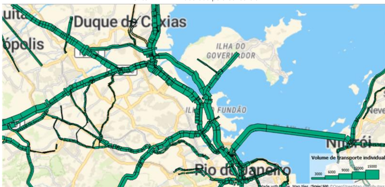
Figura 92: Carregamento de transporte individual nos principais eixos metropolitanos, Av. Brasil e Linha Vermelha
