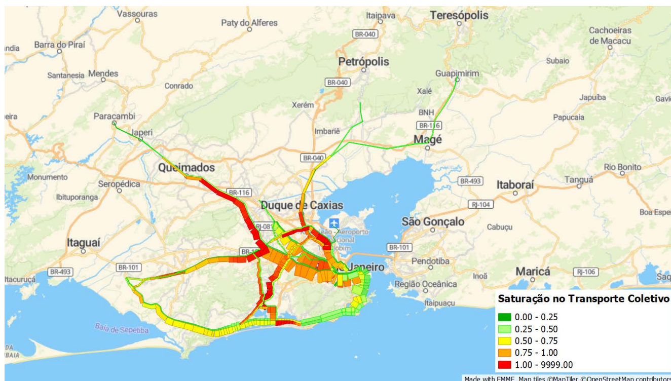
Figura 133: Saturação dos sistemas estruturantes de transporte coletivo no cenário de prognóstico
