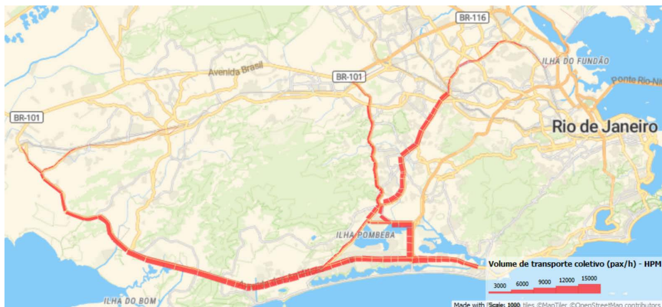
Figura 97: Carregamento dos BRTs TransOeste, TransOlímpica e TransCarioca na HPM
