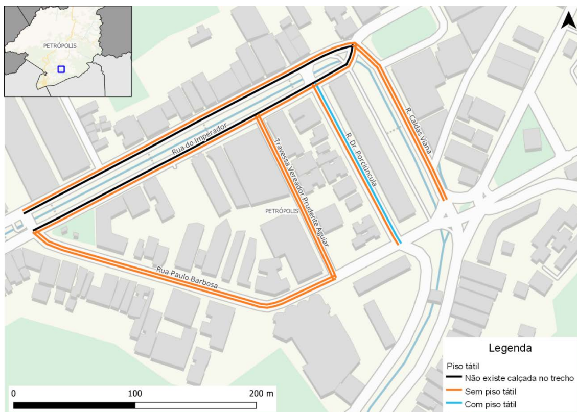
Figura 63: Existência de piso tátil nas calçadas da rede inventariada de Petrópolis
