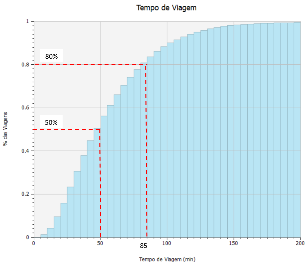
Figura 101: Histograma do tempo de viagem do transporte coletivo na RMRJ
