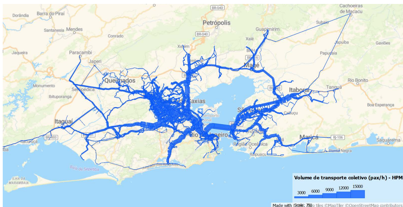
Figura 98: Carregamento de transporte coletivo – Linhas Metropolitanas
