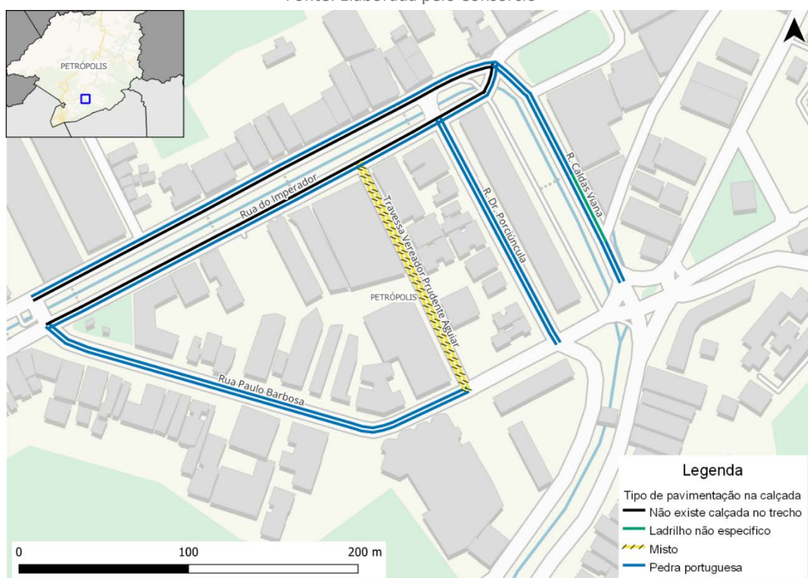
Figura 57: Tipo de pavimentação nas calçadas da rede inventariada de Petrópolis
