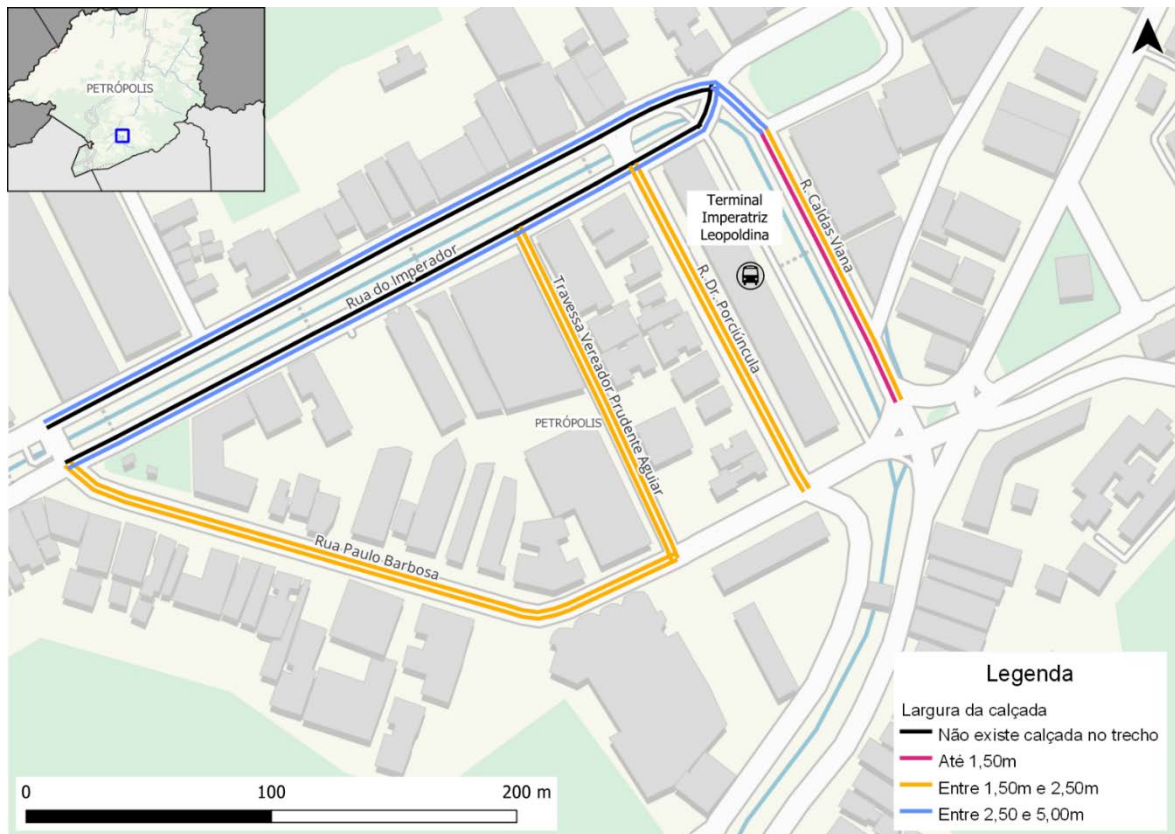
Figura 58: Largura das calçadas da rede inventariada de Petrópolis
