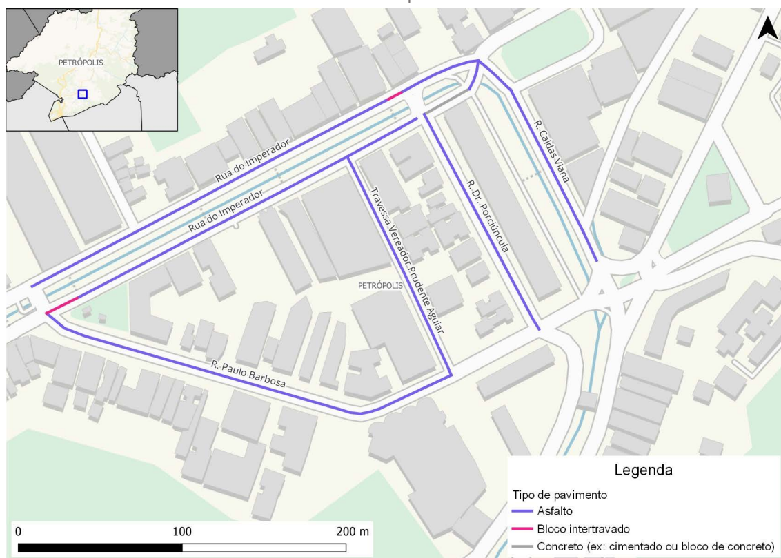
Figura 45: Tipo de pavimento na rede inventariada de Petrópolis
