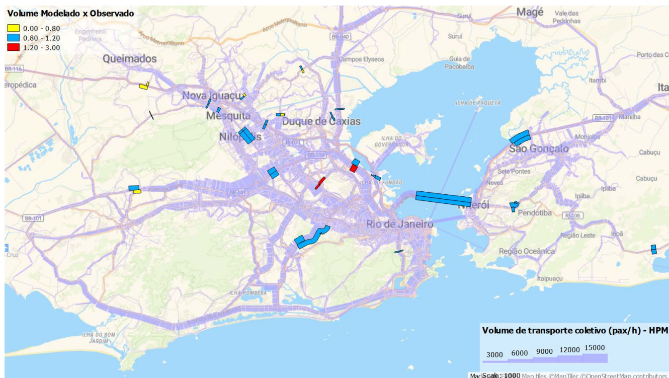
Figura 88: Volume de passageiros no Transporte Público – HPM
