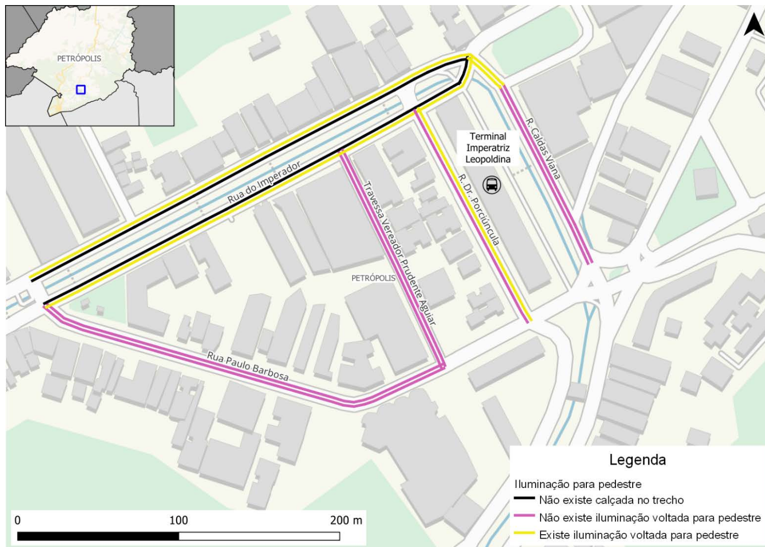
Figura 229: Iluminação para pedestre nas calçadas da rede inventariada de Petrópolis
