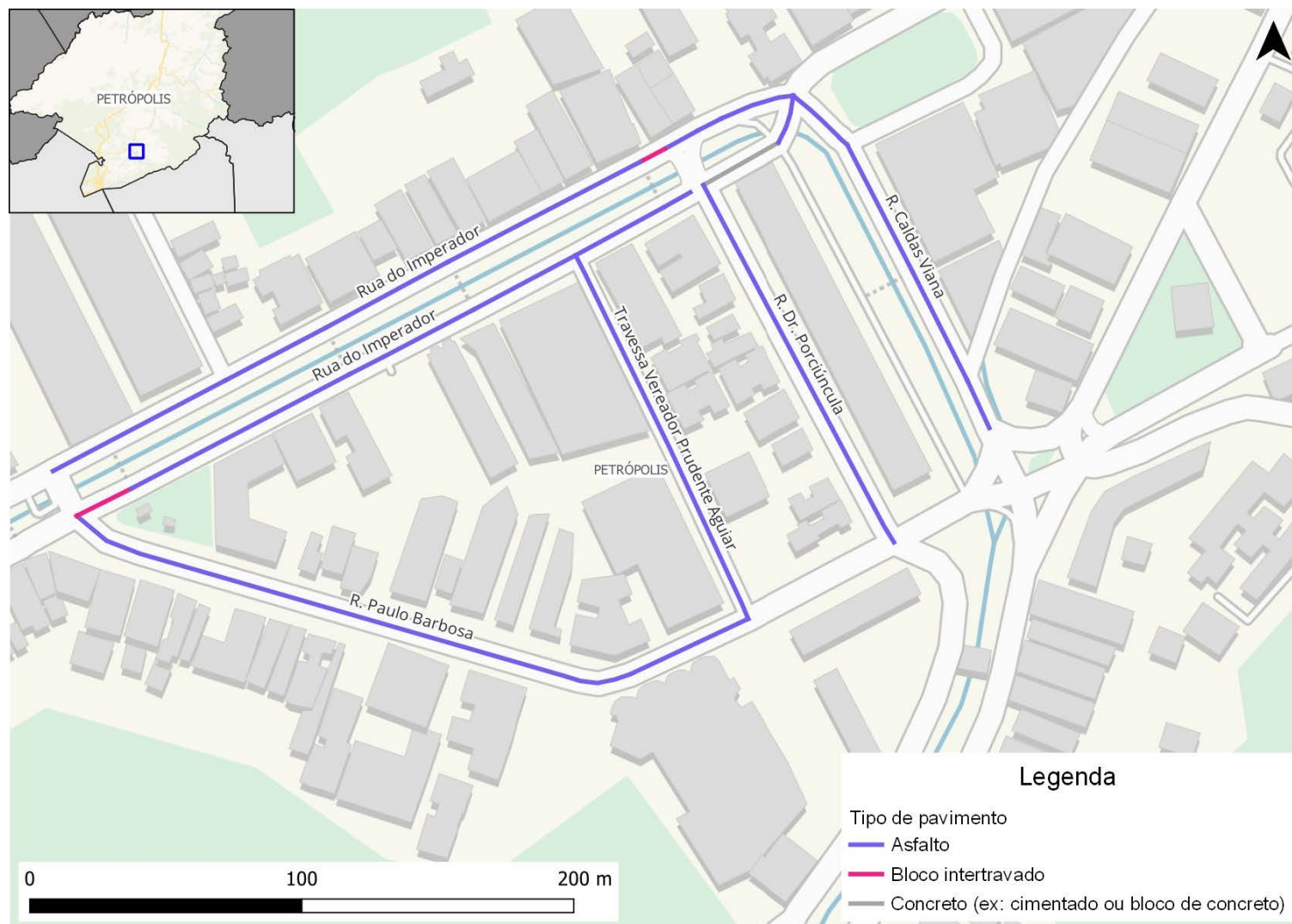
Figura 204: Tipo de pavimento na rede inventariada de Petrópolis
