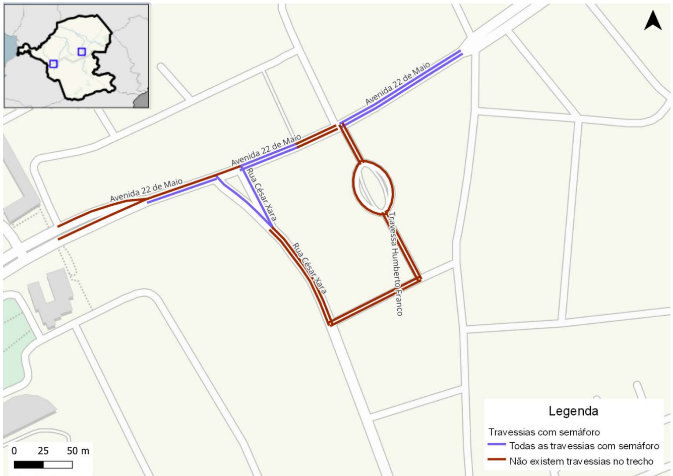
Figura 162: Travessias semaforizadas no entorno do terminal de Venda das Pedras
