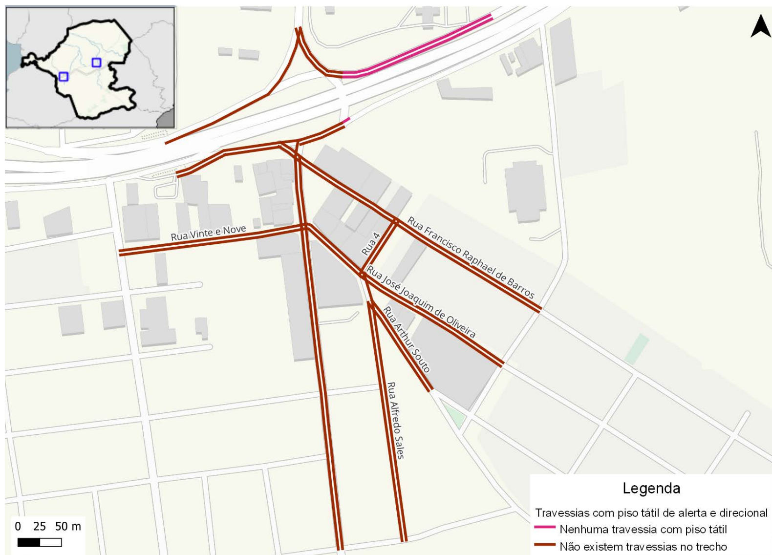
Figura 284: Travessias com piso tátil na rede inventariada de Itaboraí (Manilha)
