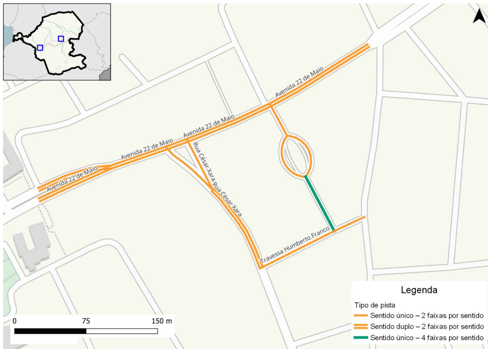
Figura 252: Tipo de pista e número de faixas por sentido na rede inventariada de Itaboraí (Venda das Pedras)
