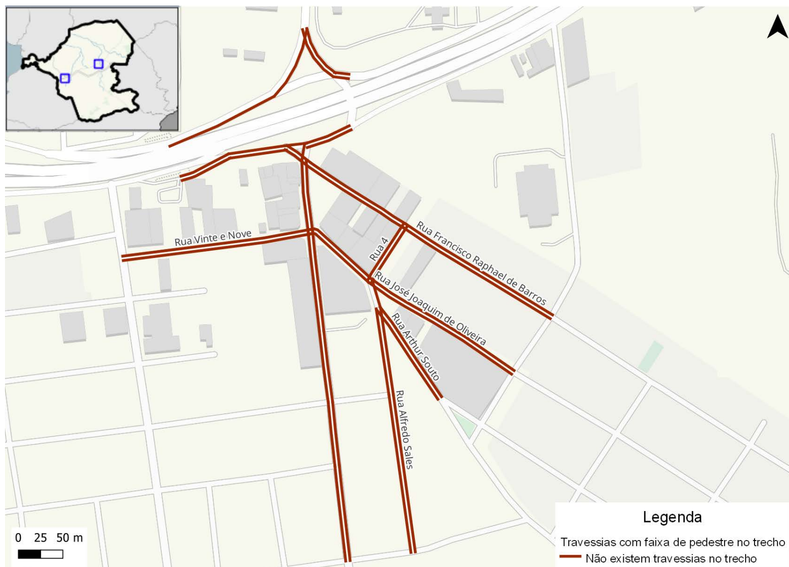
Figura 283: Travessias com faixas de pedestres na rede inventariada de Itaboraí (Manilha)
