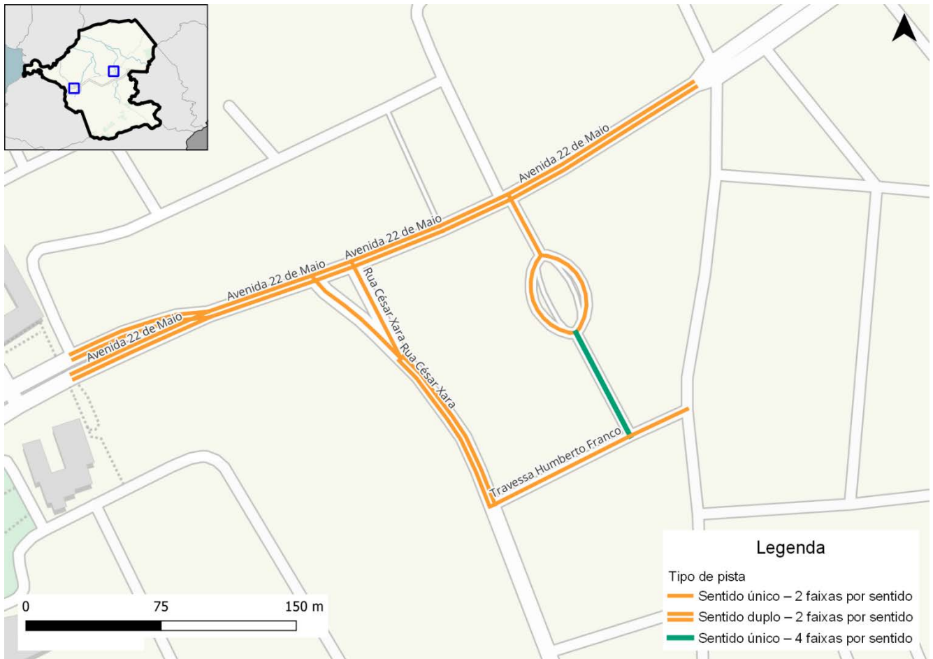
Figura 118: Tipo de pista na região do entorno do terminal de Venda das Pedras
