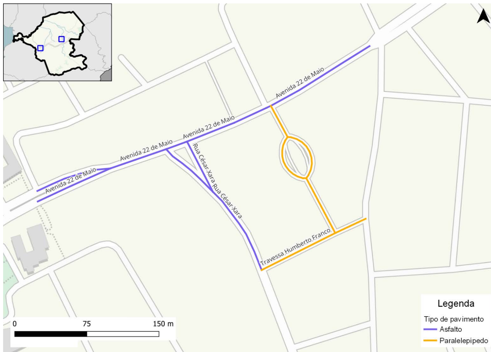
Figura 253: Tipo de pavimento na rede inventariada de Itaboraí (Venda das Pedras)
