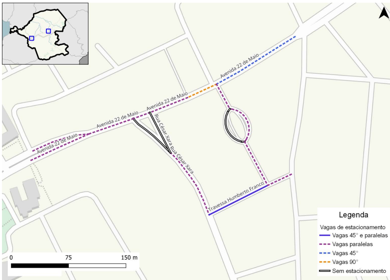
Figura 263: Tipo de vaga de estacionamento na rede inventariada de Itaboraí (Venda das Pedras)
