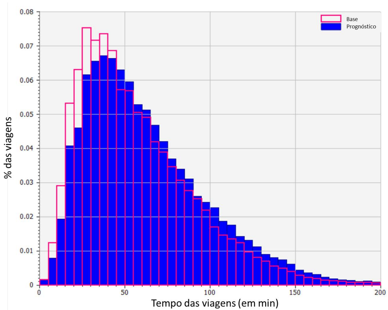
Figura 176: Histograma de comparação do tempo de viagem entre cenários base e prognóstico
