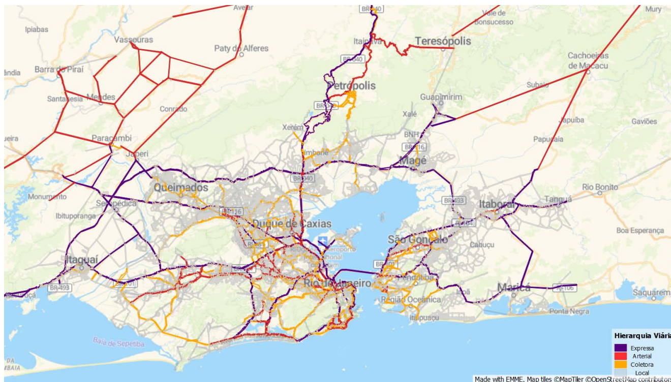
Figura 53: Hierarquia viária utilizada na rede de simulação
