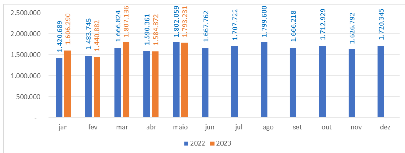
Figura 9: Demanda dos ônibus intermunicipais que passam em Itaboraí, para os anos de 2022 e 2023
