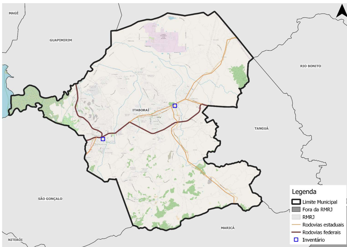
Figura 46: Localização da rede inventariada no município de Itaboraí
