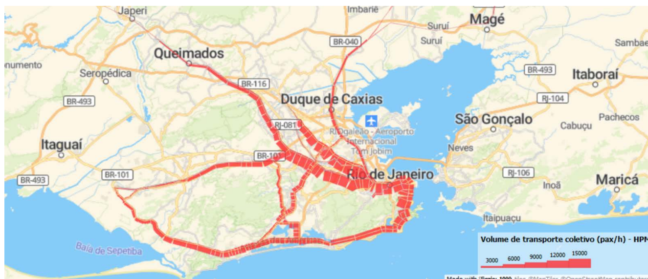
Figura 76: Carregamento do transporte coletivo – Metrô, SuperVia e BRTs
