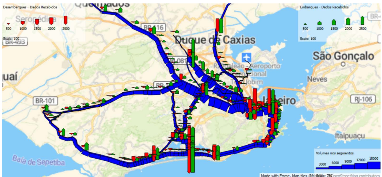
Figura 61: Volume de passageiros no sistema estruturante SuperVia, Metro e BRTs – HPM
