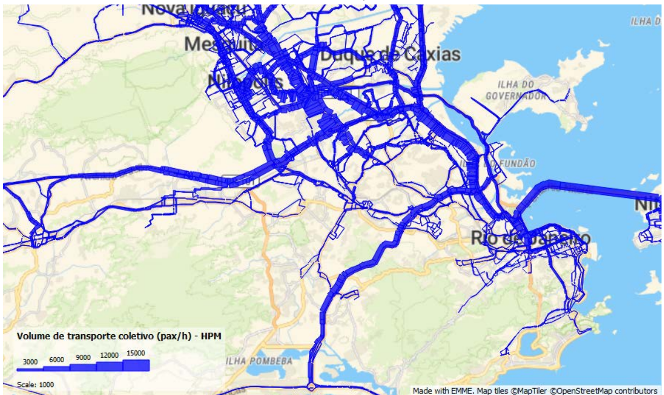
Figura 81: Destaque do carregamento de transporte coletivo - Linhas Metropolitanas
