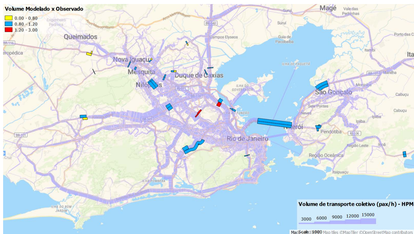
Figura 68: Volume de passageiros no Transporte Público – HPM
