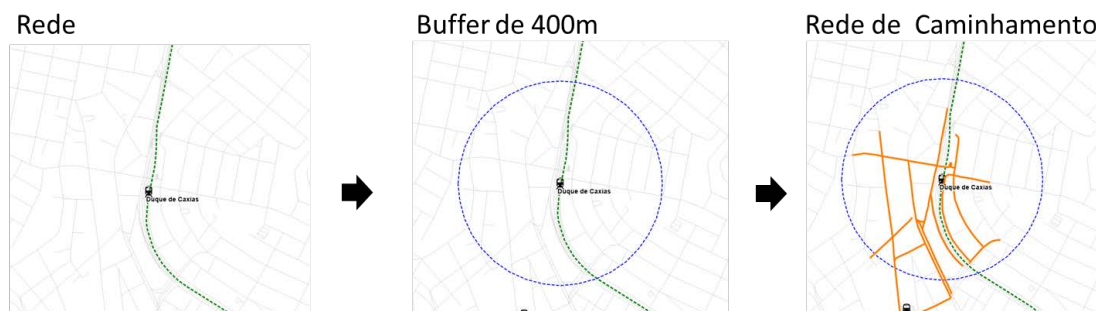
Figura 43: Metodologia de definição da rede de caminhada
