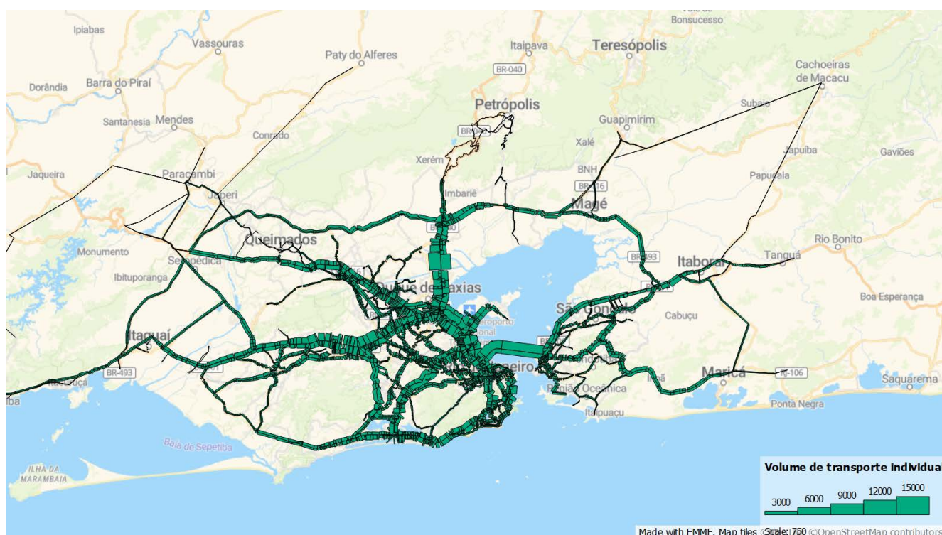
Figura 71: Carregamento de transporte individual nos principais eixos metropolitanos
