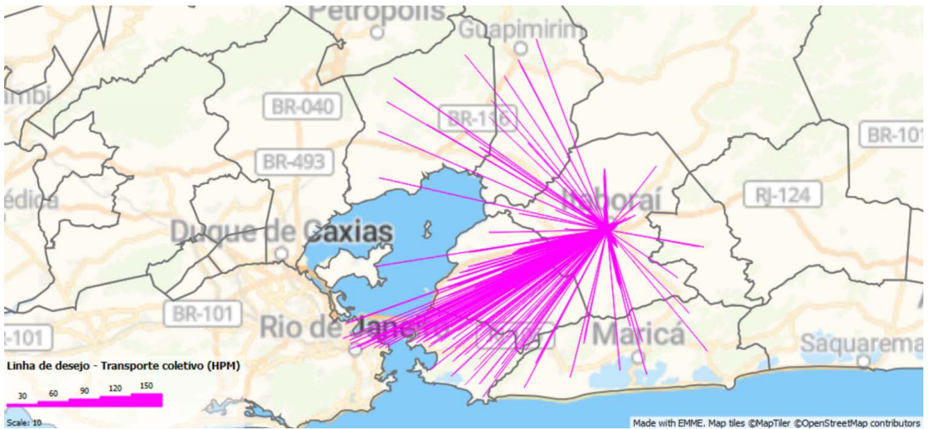
Figura 86: Linhas de desejo de origens no município de Itaboraí durante o pico da manhã
