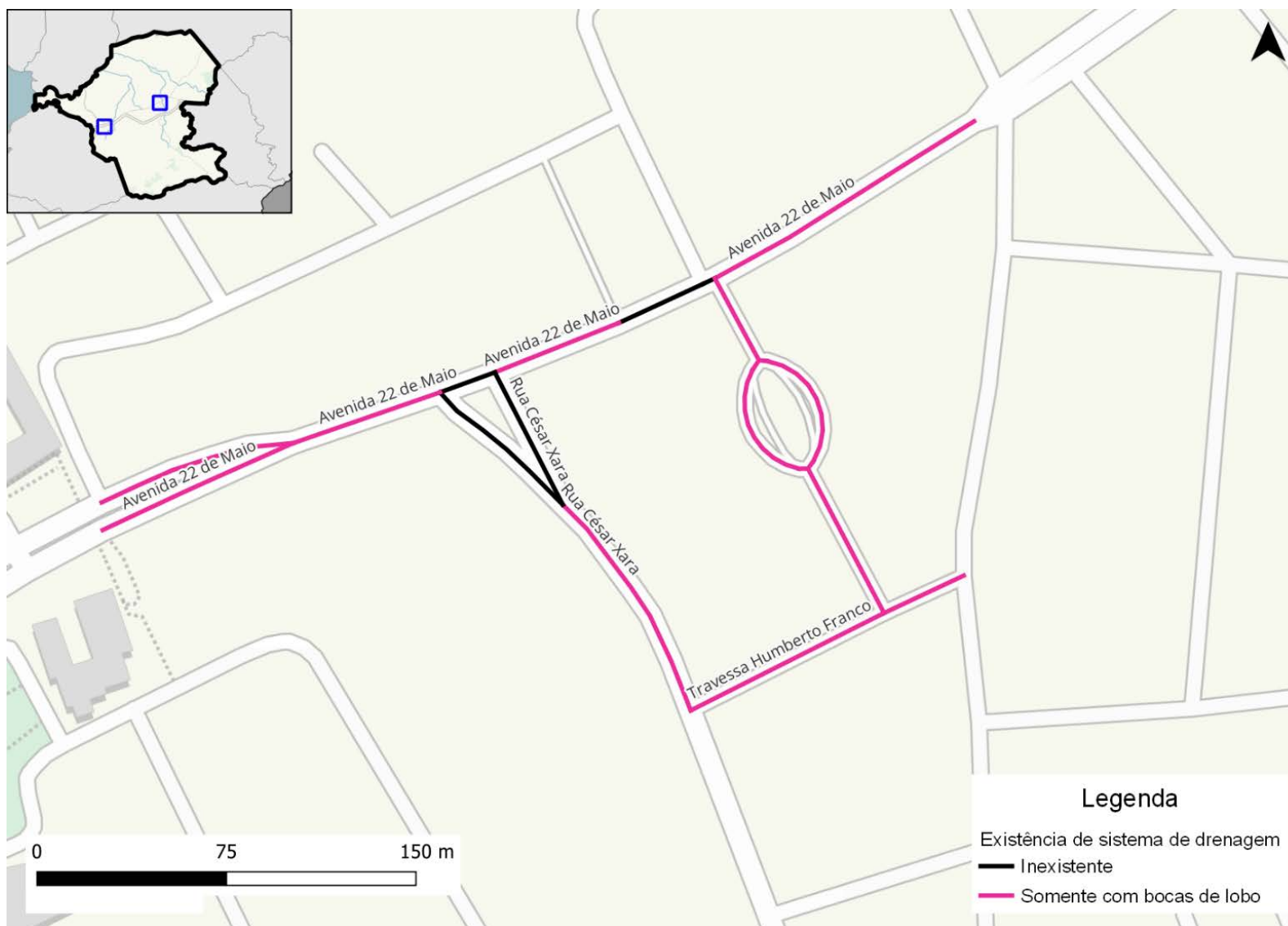
Figura 256: Equipamentos de drenagem na rede inventariada de Itaboraí (Venda das Pedras)
