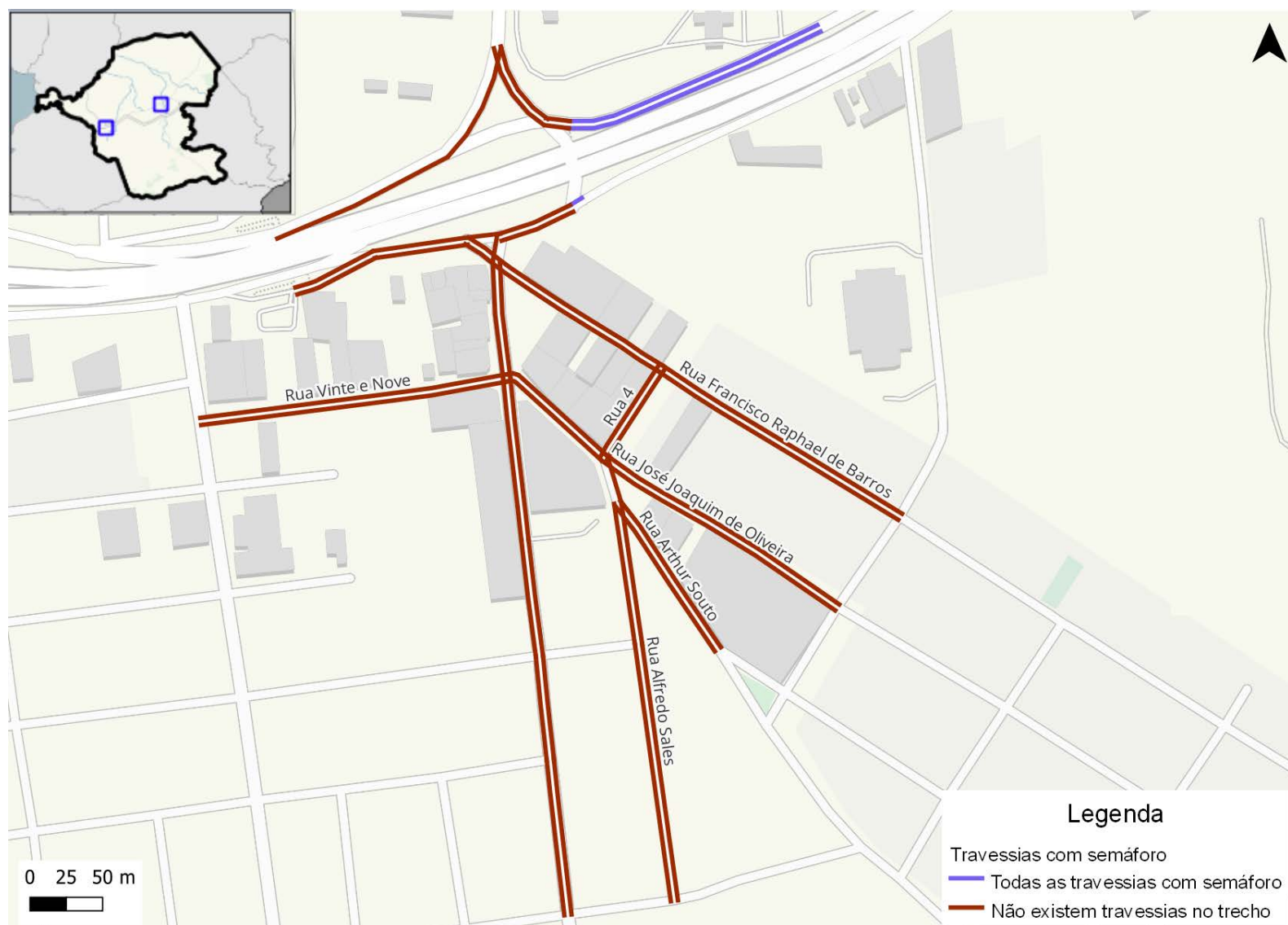
Figura 282: Travessias semaforizadas na rede inventariada de Itaboraí (Manilha)
