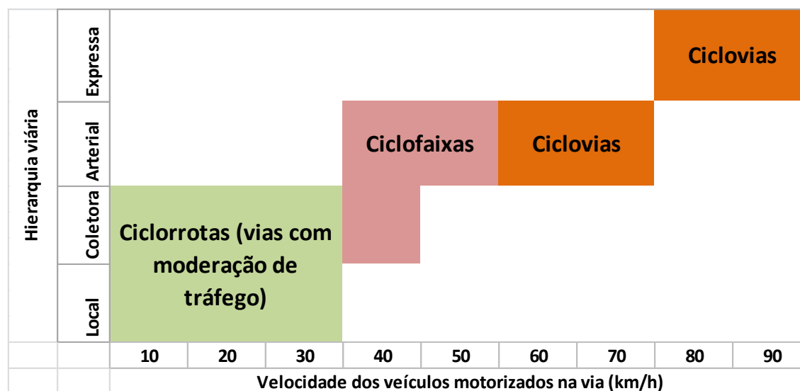
Figura 197: Tipologia de tratamento ciclovitário de acordo com hierarquia viária e velocidade da via
