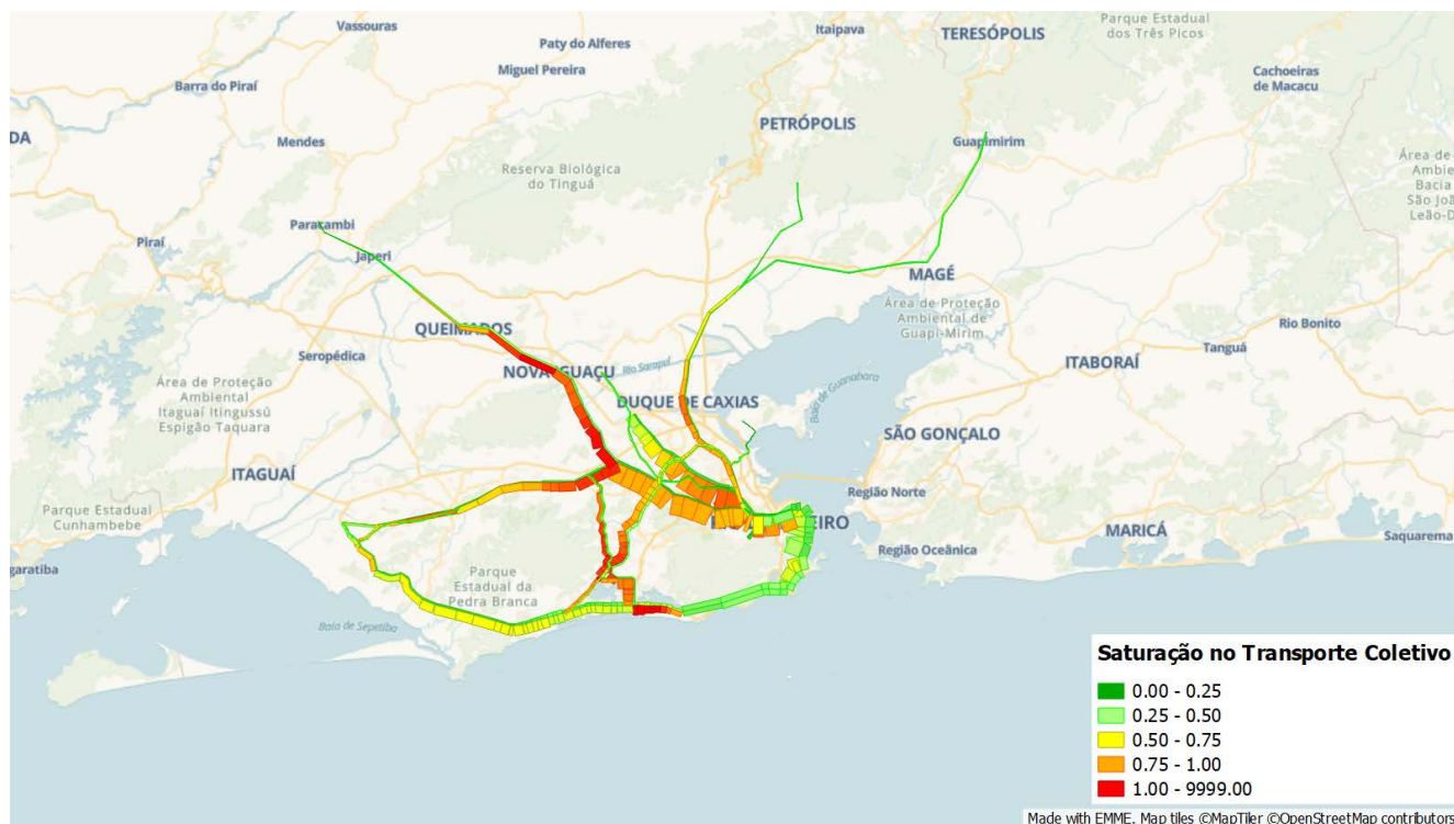
Figura 82: Nível de saturação no sistema de transporte estruturante de alta capacidade
