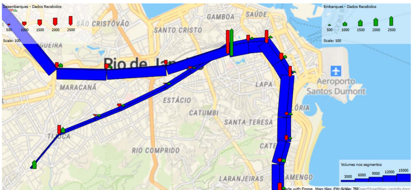
Figura 63: Volume de passageiros no metrô – zoom na região central
