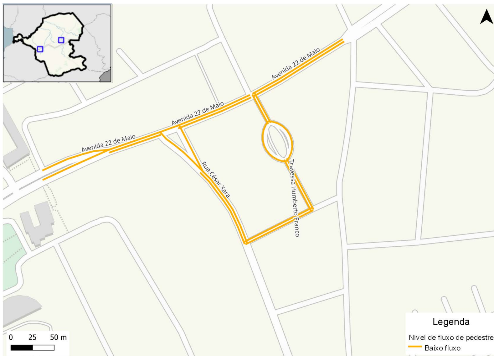
Figura 299: Fluxo de pedestres nas calçadas da rede inventariada de Itaboraí (Venda das Pedras)
