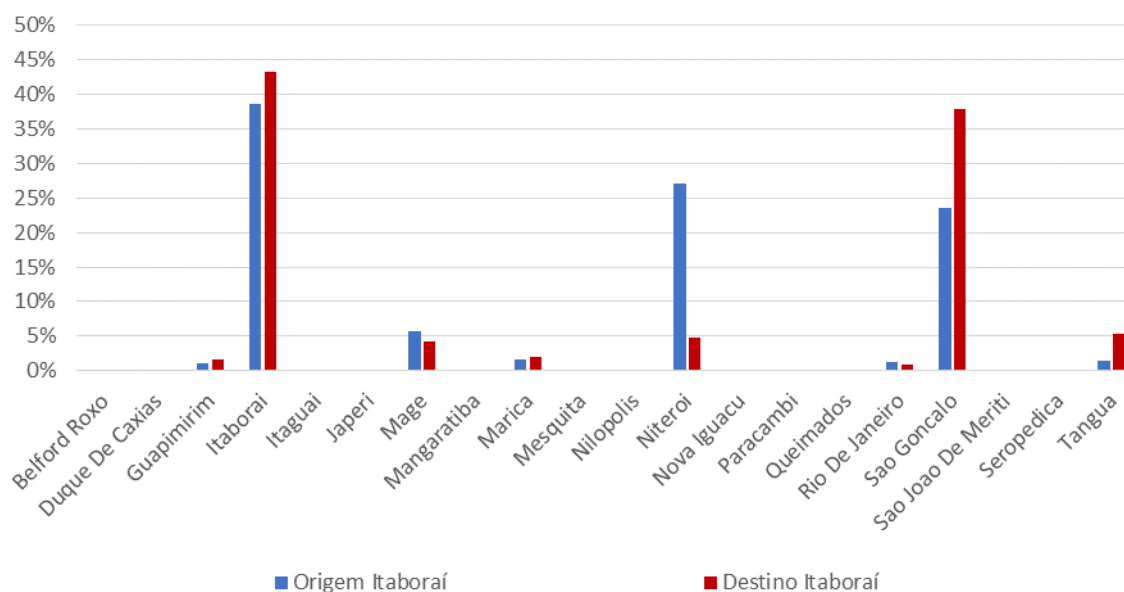
Figura 154: Origens e destinos das viagens em Itaboraí, por transporte coletivo – Pico da Manhã
