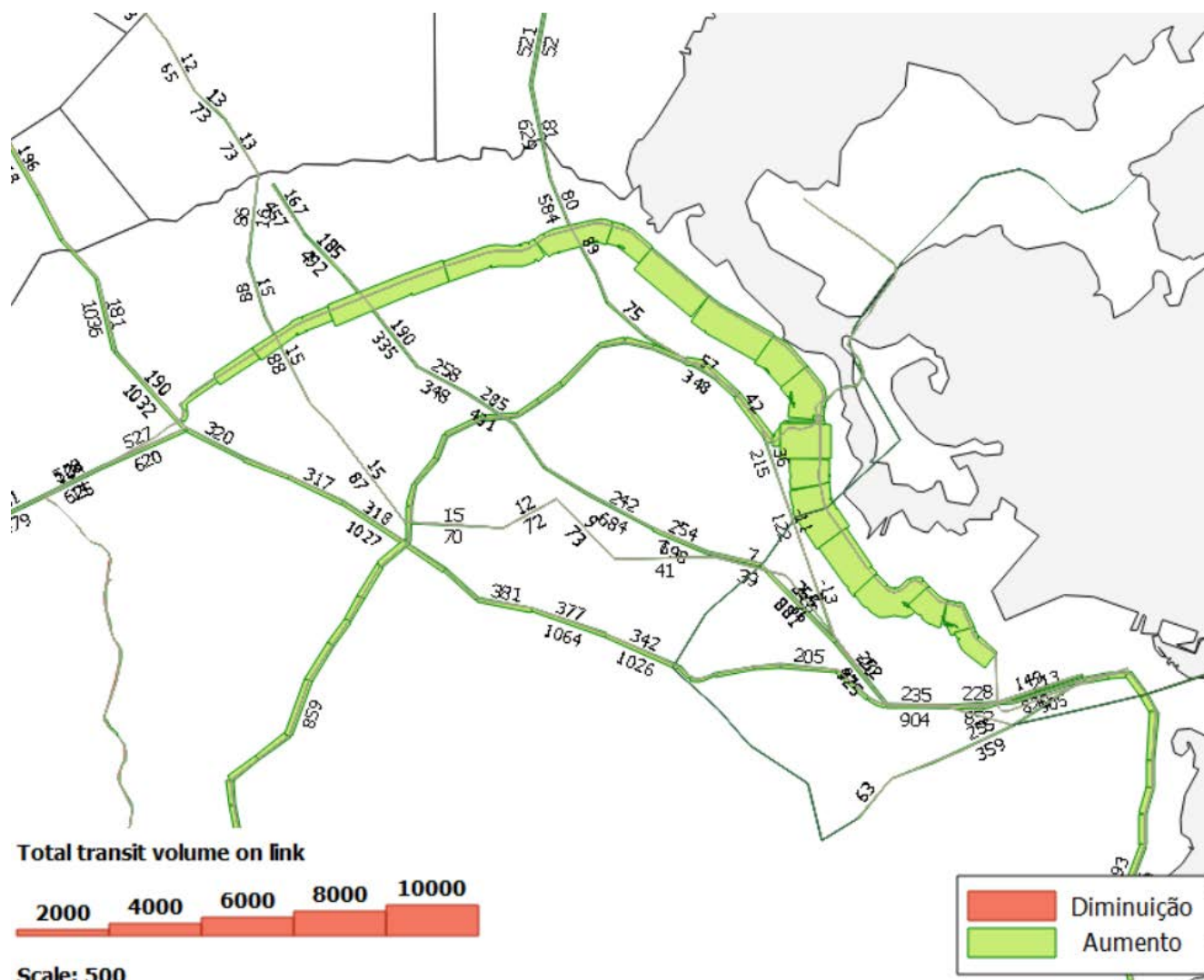
Figura 175: Comparação dos volumes de transporte coletivo no cenário base e no cenário de prognóstico
