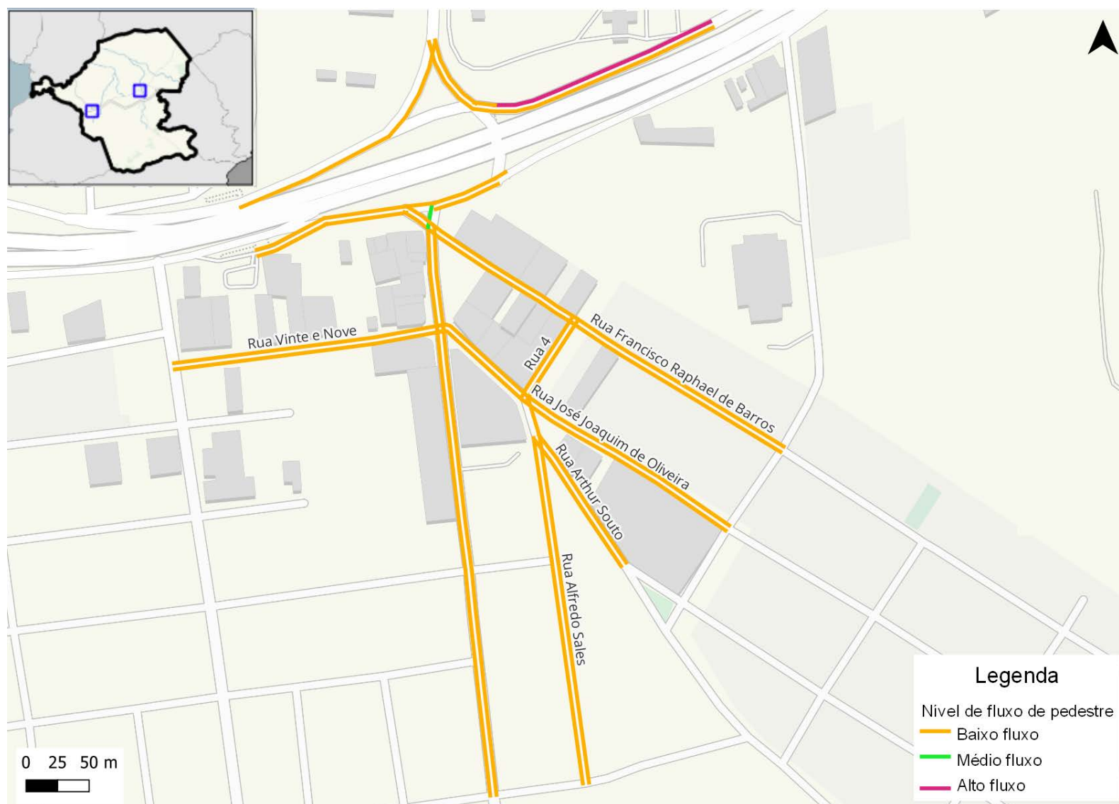
Figura 281: Fluxo de pedestres nas calçadas da rede inventariada de Itaboraí (Manilha)
