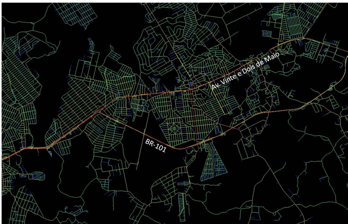
Figura 17: Exemplo do resultado da simulação no DepthmapX para Itaboraí
