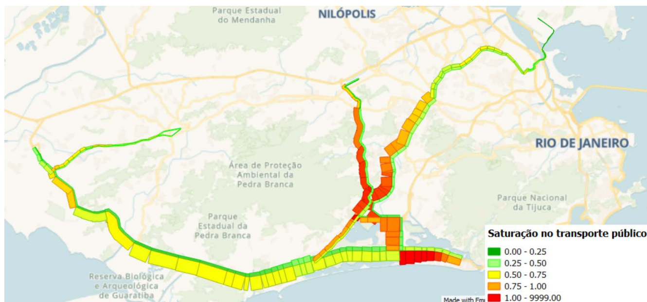
Figura 85: Nível de saturação no sistema de BRTs
