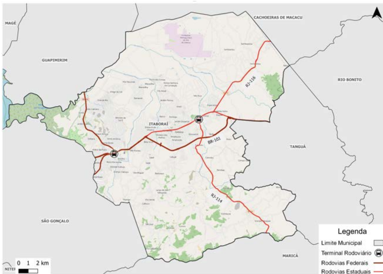
Figura 121: Localização dos terminais em Itaboraí
