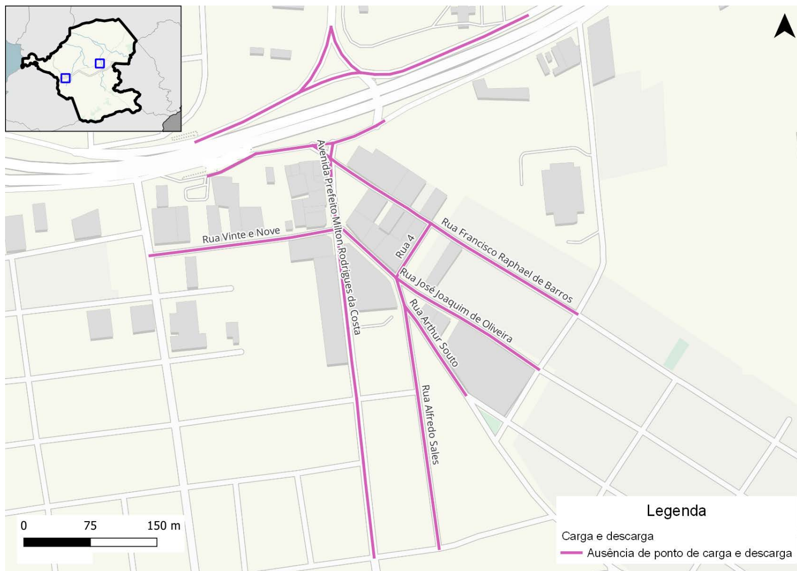
Figura 249: Vagas de carga e descarga na rede inventariada de Itaboraí (Manilha)
