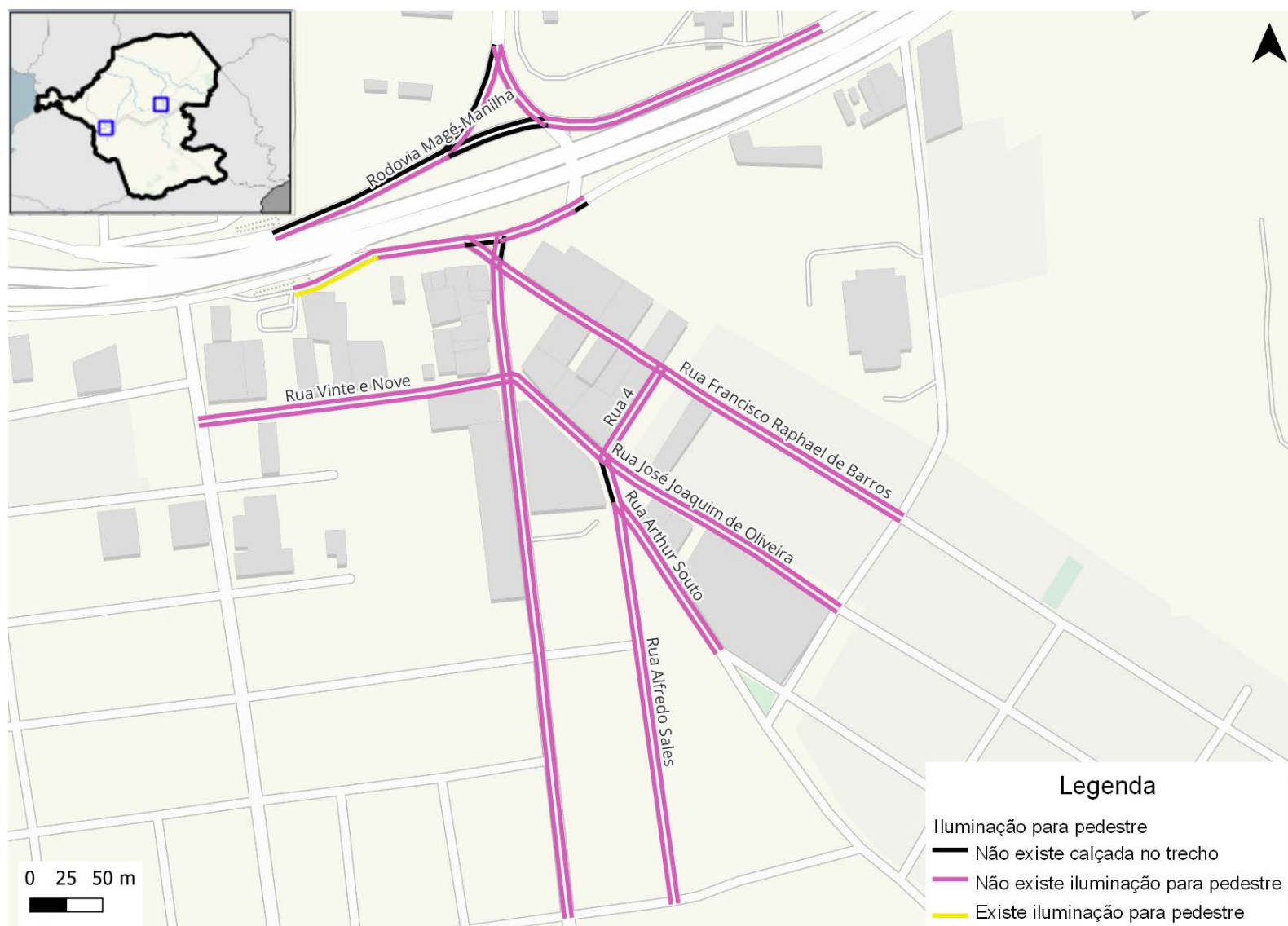
Figura 278: Iluminação para pedestre nas calçadas da rede inventariada de Itaboraí (Manilha)
