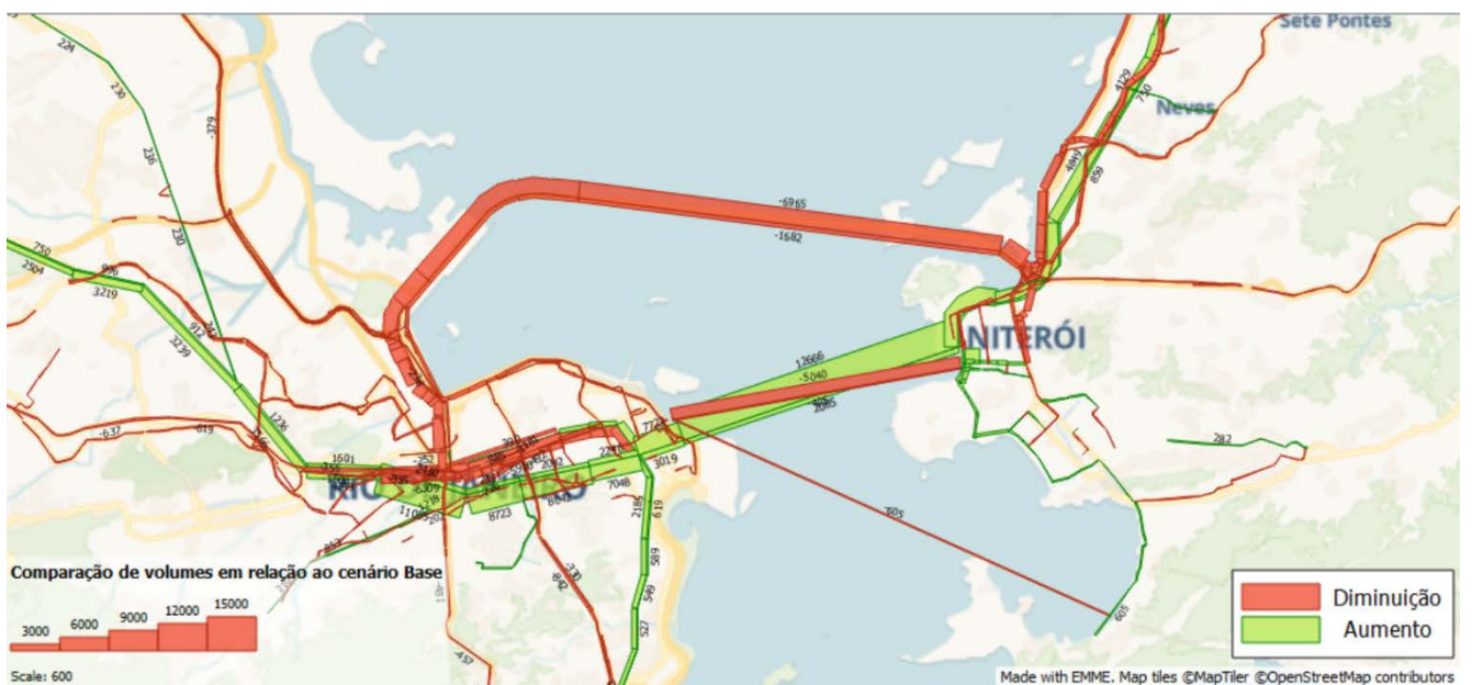
Figura 92: Comparação do carregamento entre cenário base e cenário com a Linha 3
