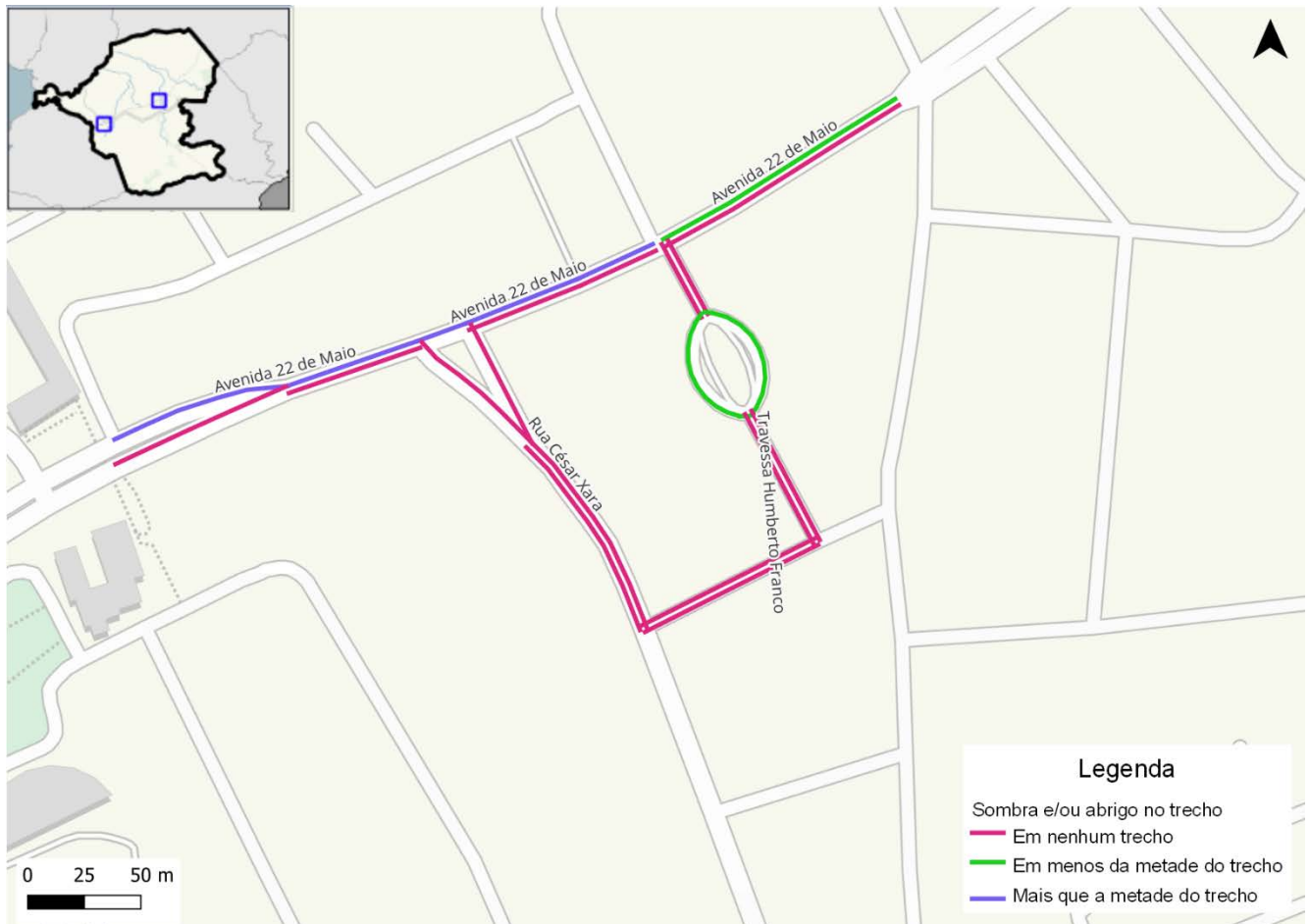
Figura 146: Presença de sombra e abrigo nas calçadas na região do entorno do terminal de Venda das Pedras
