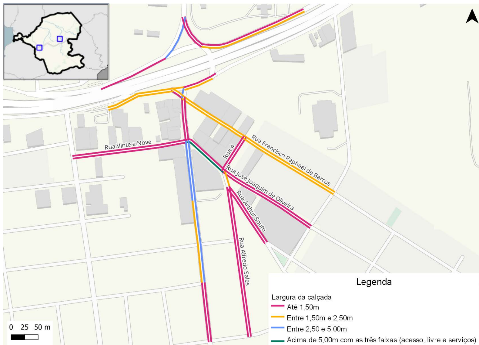
Figura 270: Largura das calçadas da rede inventariada de Itaboraí (Manilha)
