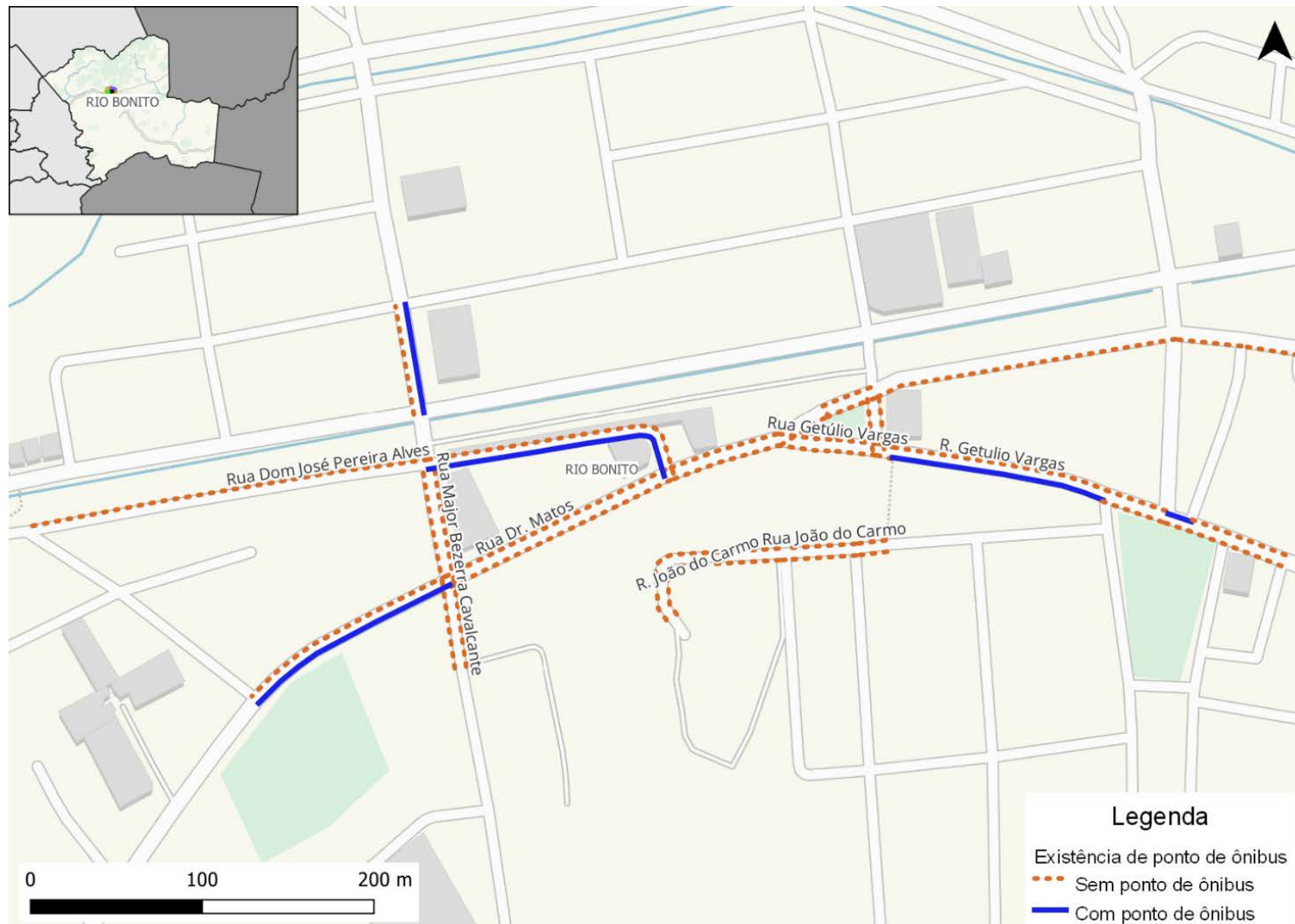
Figura 232: Existência de ponto de ônibus na rede inventariada de Rio Bonito
