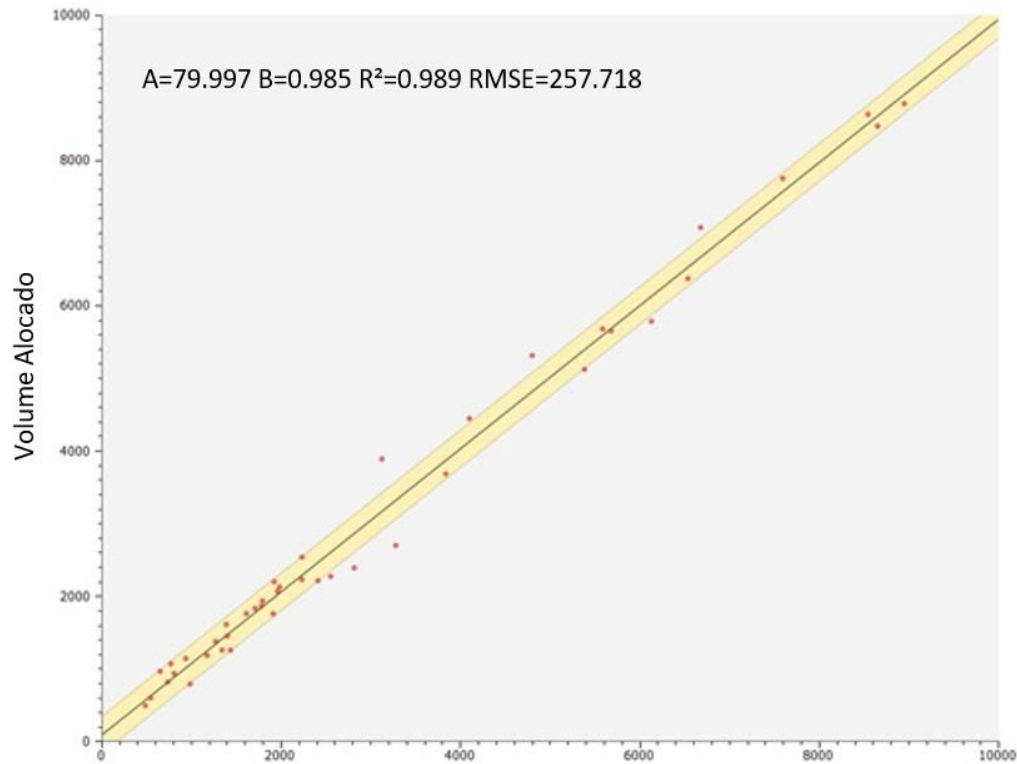
Figura 73: Gráfico do volume alocado x observado para transporte público
