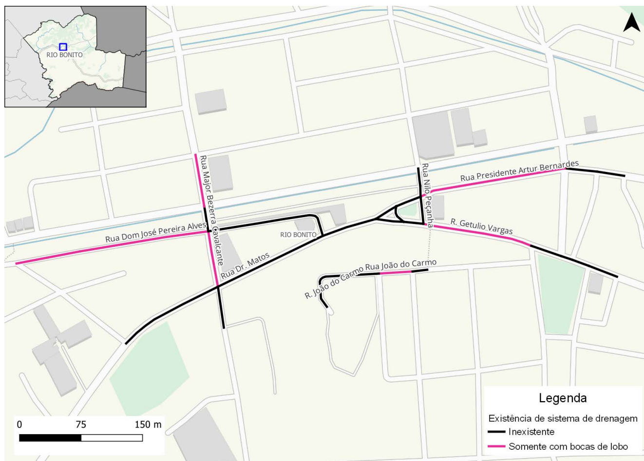
Figura 103: Sistema de drenagem no entorno da Rodoviária de Rio Bonito
