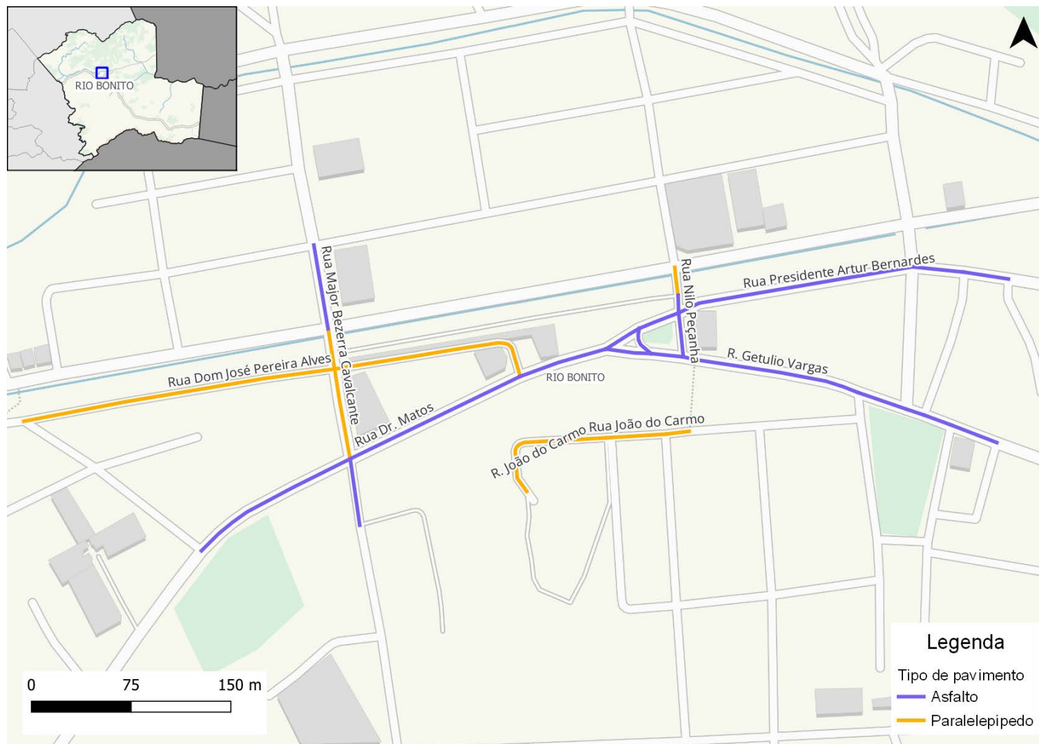
Figura 214: Tipo de pavimento na rede inventariada de Rio Bonito
