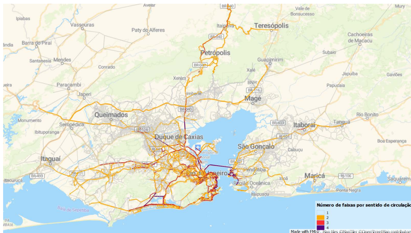
Figura 54: Número de faixas na rede de simulação RMRJ
