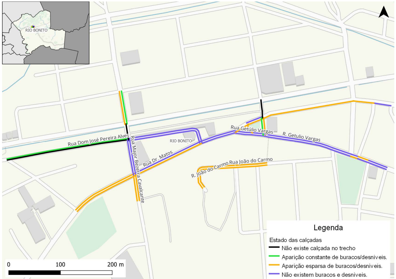
Figura 126: Estado das calçadas no entorno da Rodoviária de Rio Bonito
