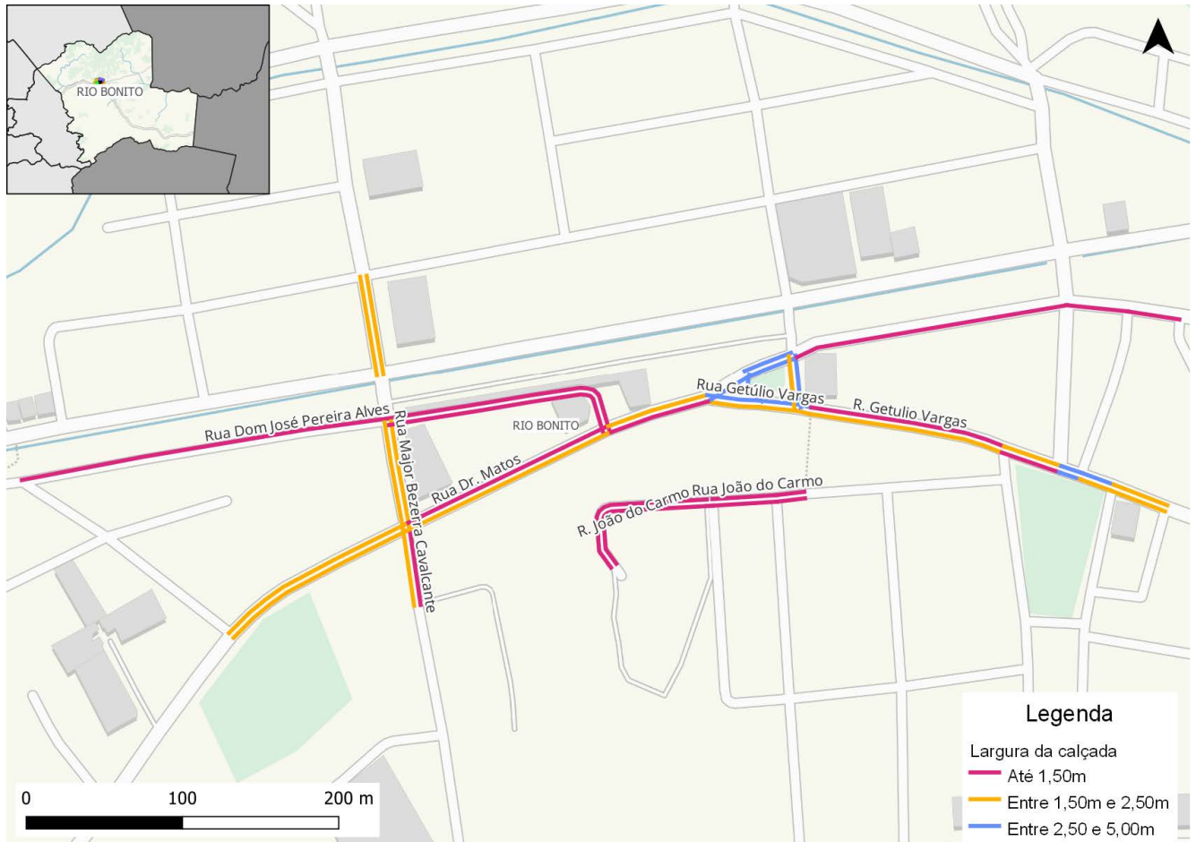
Figura 127: Largura das calçadas no entorno da Rodoviária de Rio Bonito
