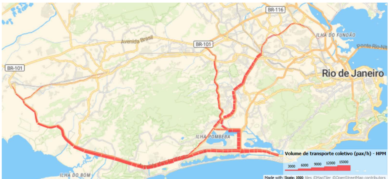
Figura 81: Carregamento dos BRTs TransOeste, TransOlímpica e TransCarioca na HPM
