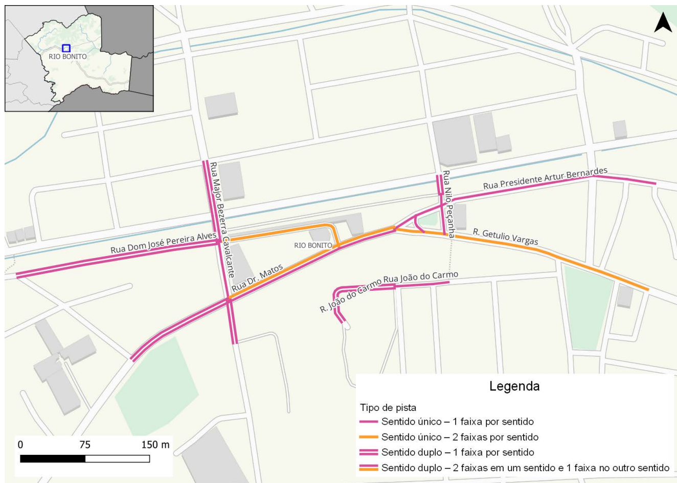
Figura 101: Tipo de pista no entorno da Rodoviária de Rio Bonito
