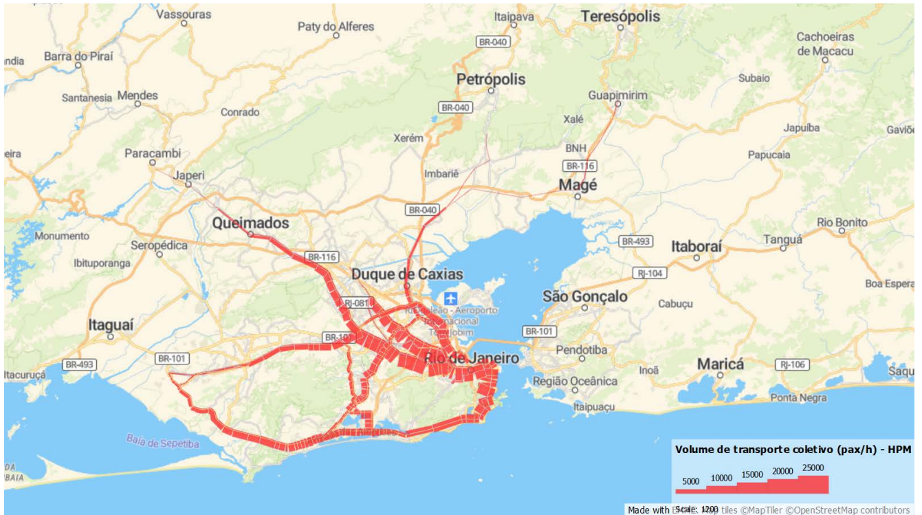
Figura 148: Volume de transporte coletivo na HPM, para o cenário de prognóstico no horizonte de 10 anos
