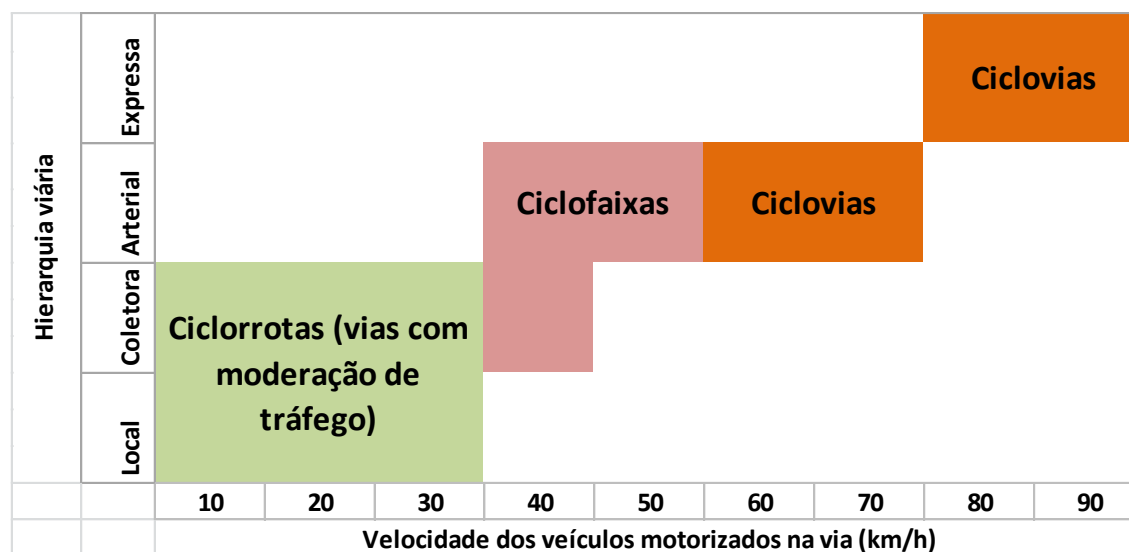
Figura 172: Tipologia de tratamento ciclovitário de acordo com hierarquia viária e velocidade da via
