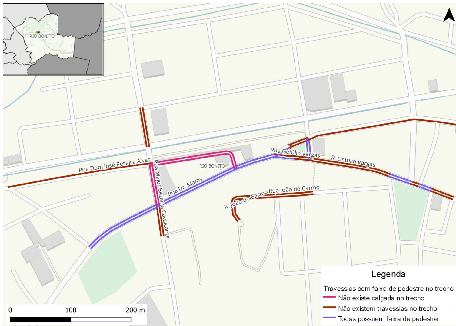
Figura 244: Travessias com faixas de pedestres na rede inventariada de Rio Bonito
