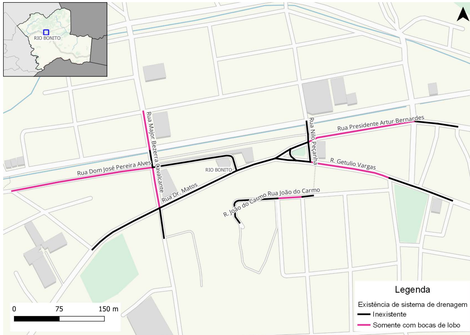
Figura 217: Equipamentos de drenagem na rede inventariada de Rio Bonito
