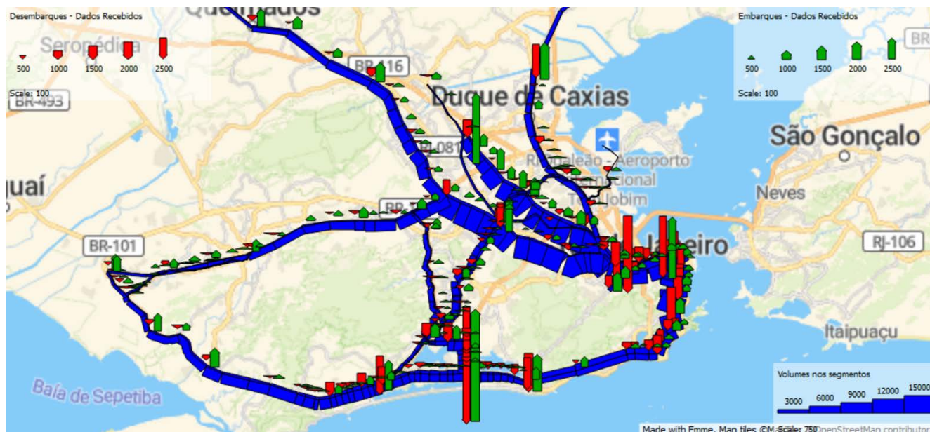
Figura 65: Volume de passageiros no sistema estruturante Supervia, Metro e BRTs – HPM
