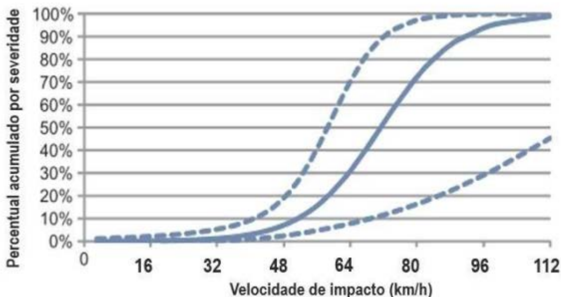
Figura 192: Probabilidade de fatalidades em atropelamentos em relação à velocidade do condutor no momento do acidente. 31
