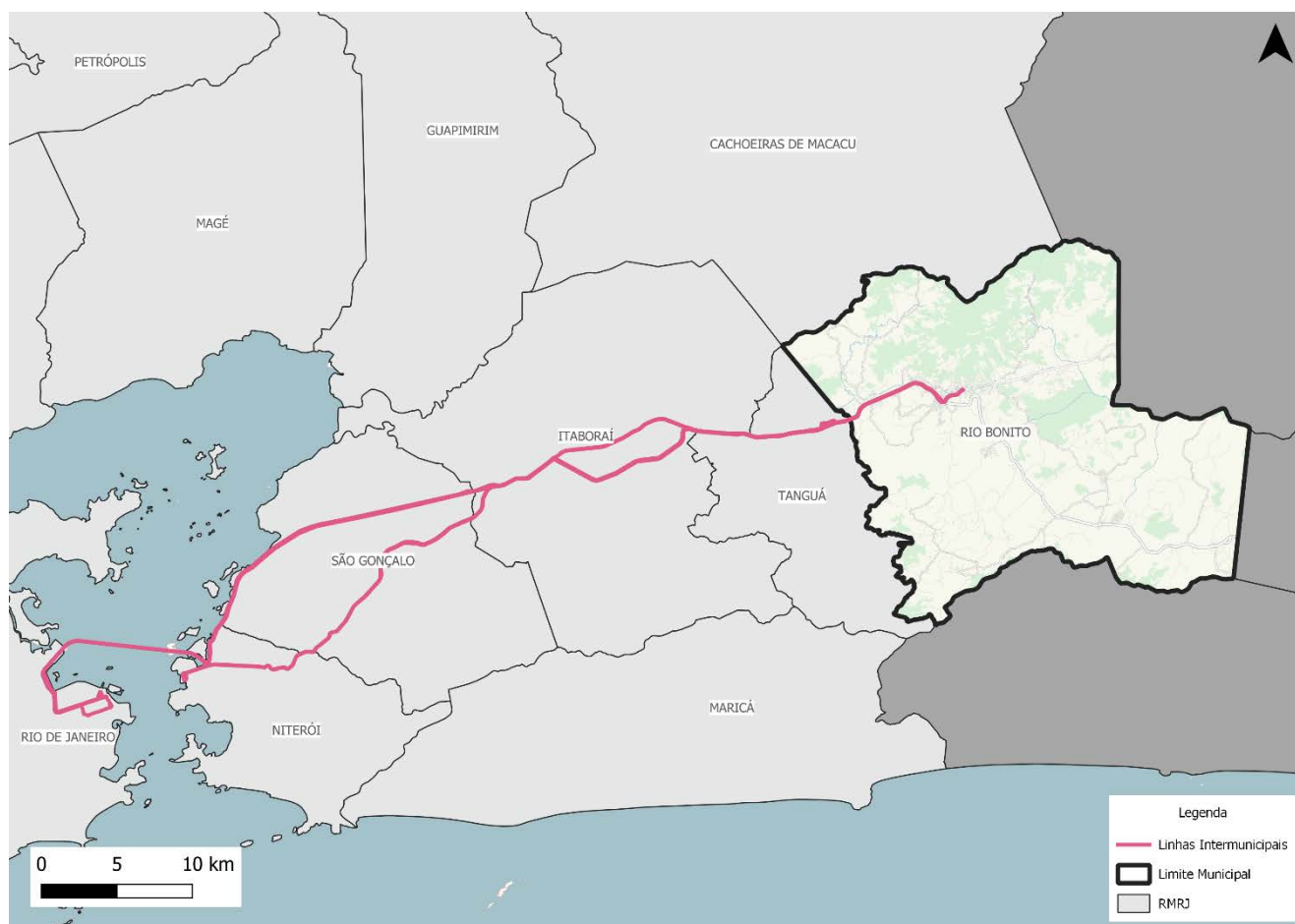
Figura 107: Linhas Intermunicipais que atendem ao município de Rio Bonito
