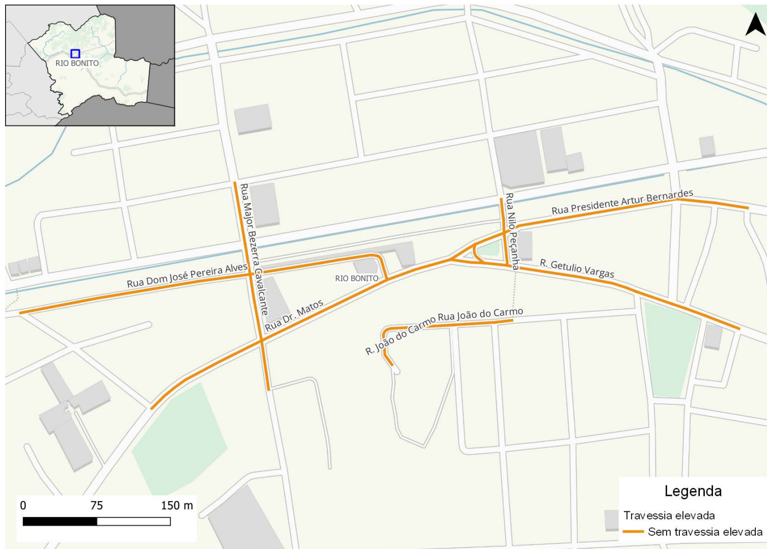
Figura 219: Travessia elevada de pedestre na rede inventariada de Rio Bonito
