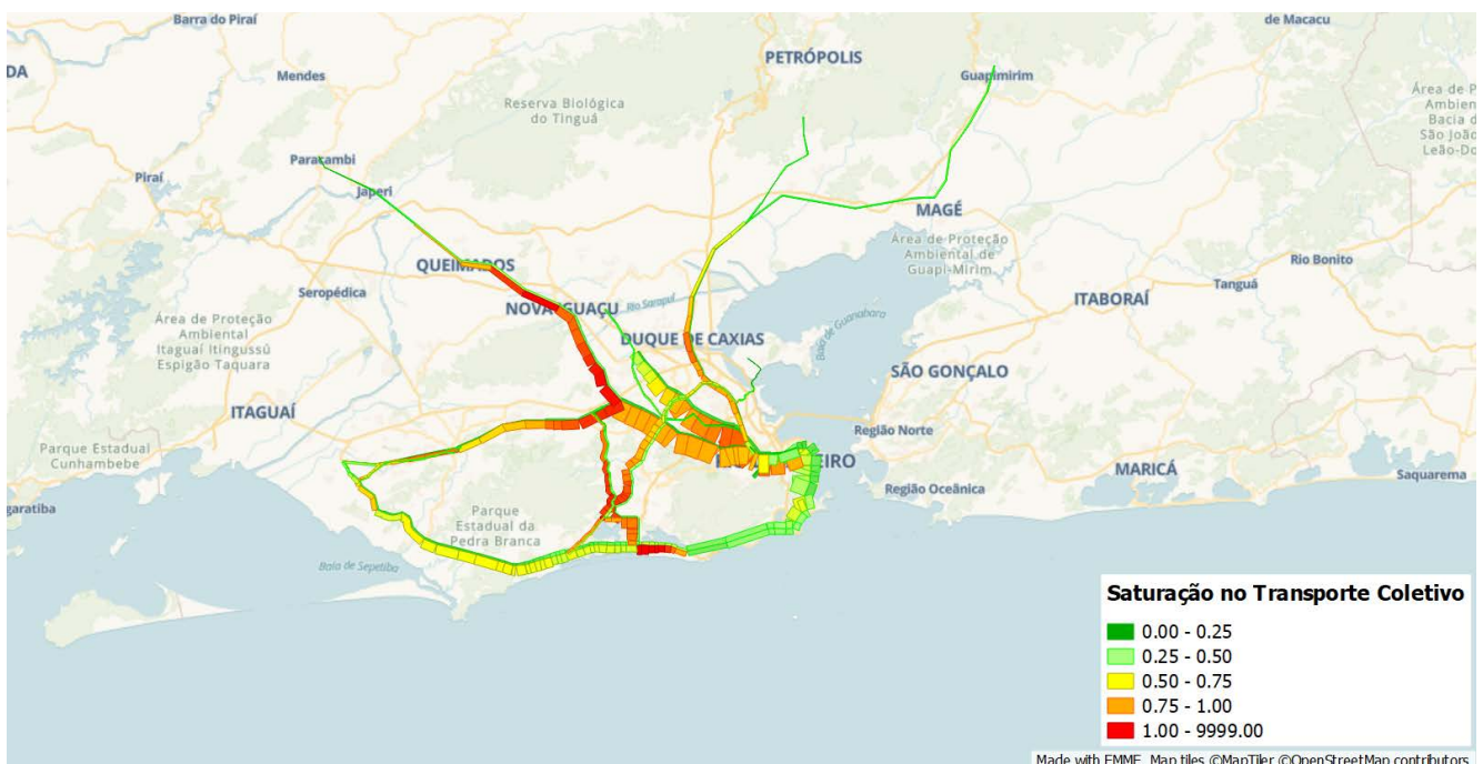
Figura 84: Nível de saturação no sistema de transporte estruturante de alta capacidade
