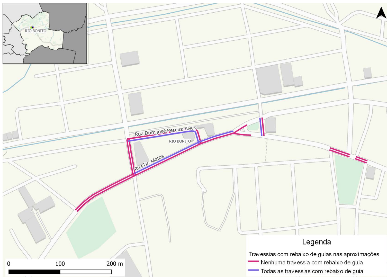
Figura 246: Travessias com rebaixo de guia nas aproximações na rede inventariada de Rio Bonito
