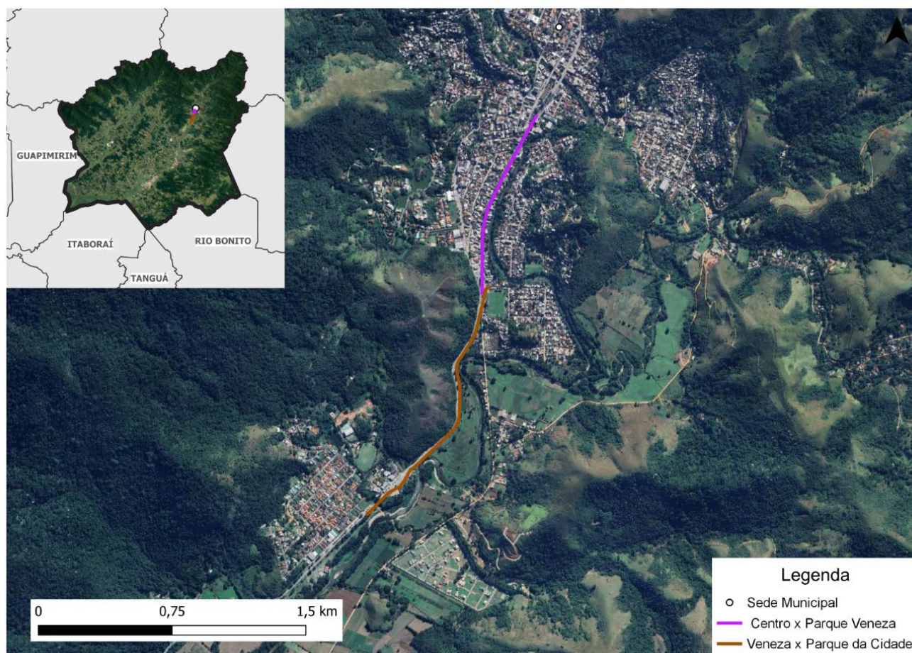
Figura 199: Ciclovia e ciclofaixa projetadas
