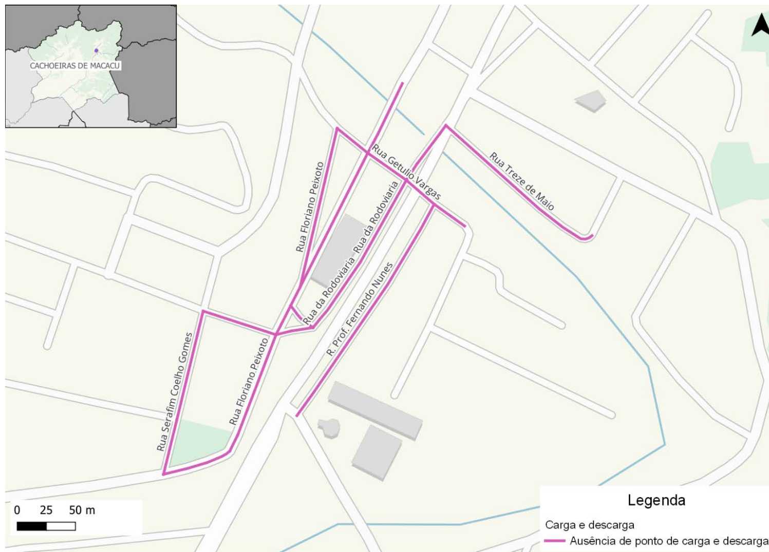
Figura 268: Vagas de carga e descarga na rede inventariada de Cachoeiras de Macacu
