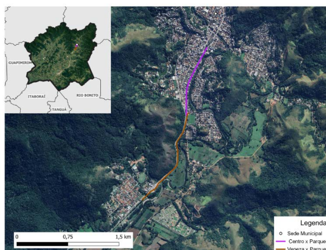
Figura 25: Ciclovía e ciclofaixa projetadas
