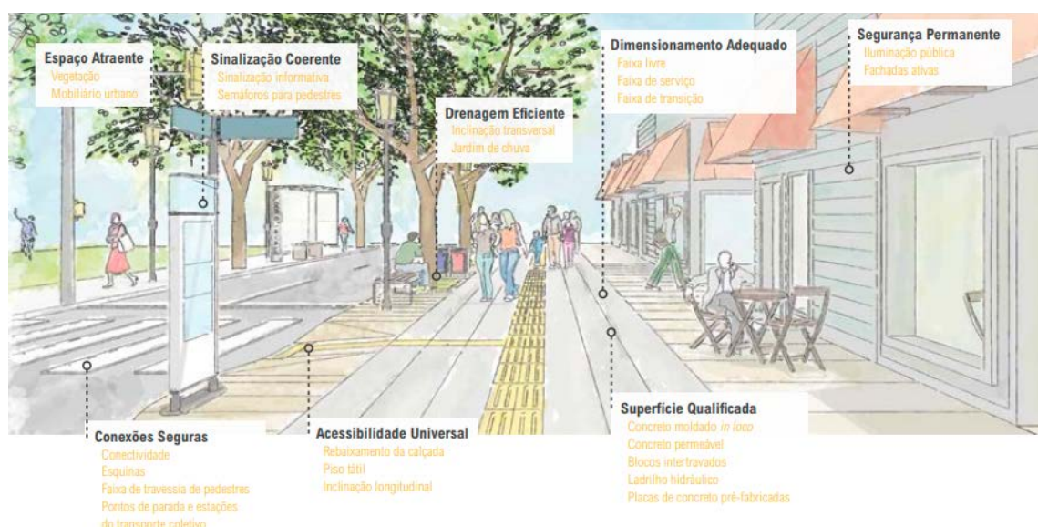
Figura 21: Esquema ilustrativo de calçada ideal
