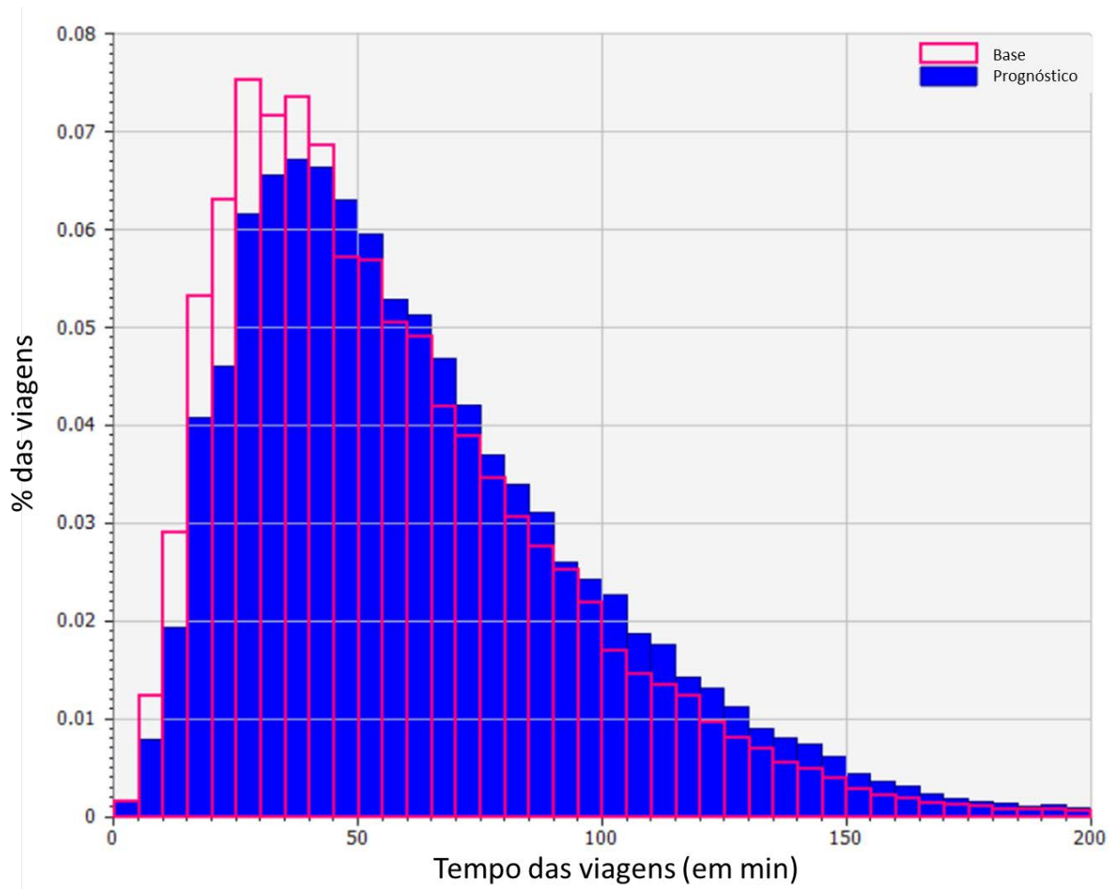
Figura 181: Histograma de comparação do tempo de viagem entre cenários base e prognóstico
