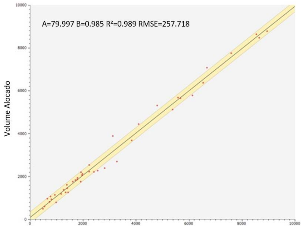
Figura 84: Gráfico do volume alocado x observado para transporte público
