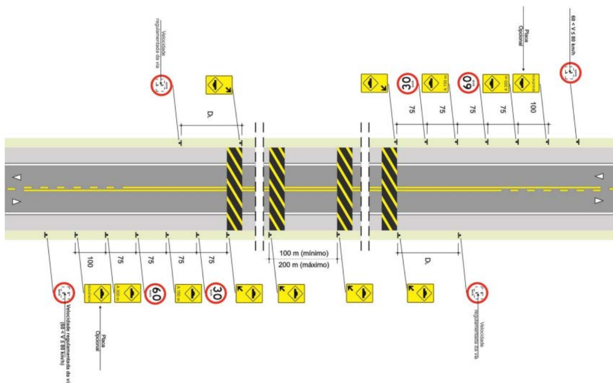
Figura 218: Exemplo de sinalização em rodovia com velocidade regulamentada maior que 60km/h e menor ou igual a 80km/h
