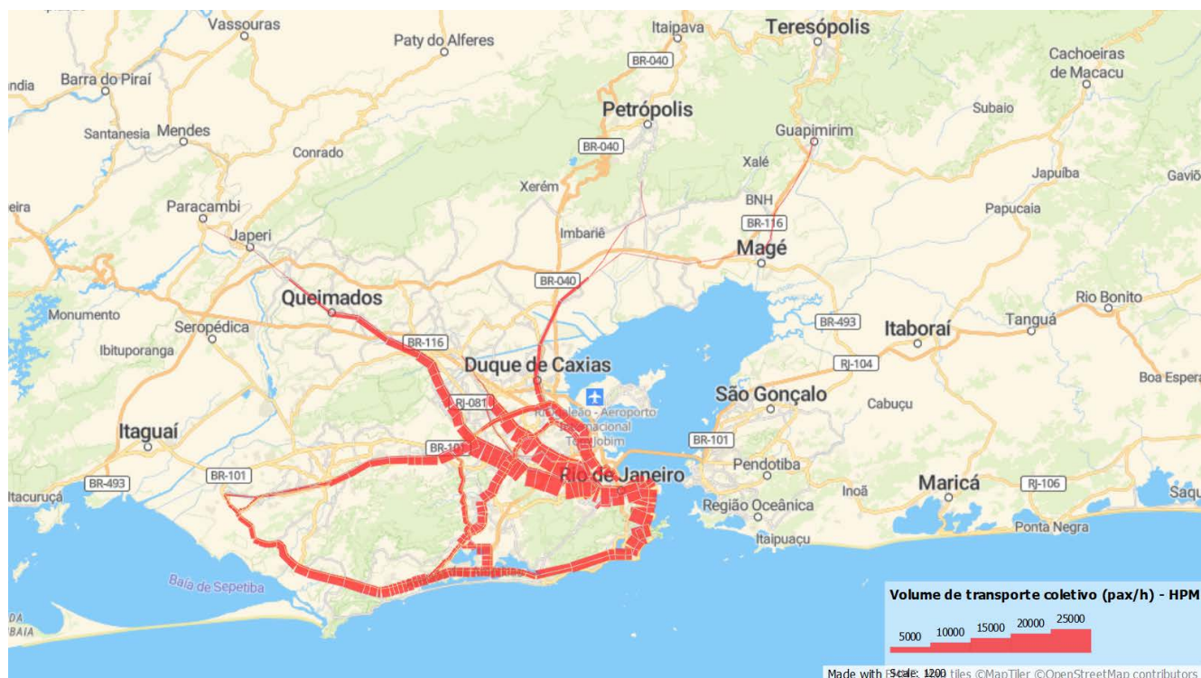
Figura 156: Volume de transporte coletivo na HPM, para o cenário de prognóstico no horizonte de 10 anos
