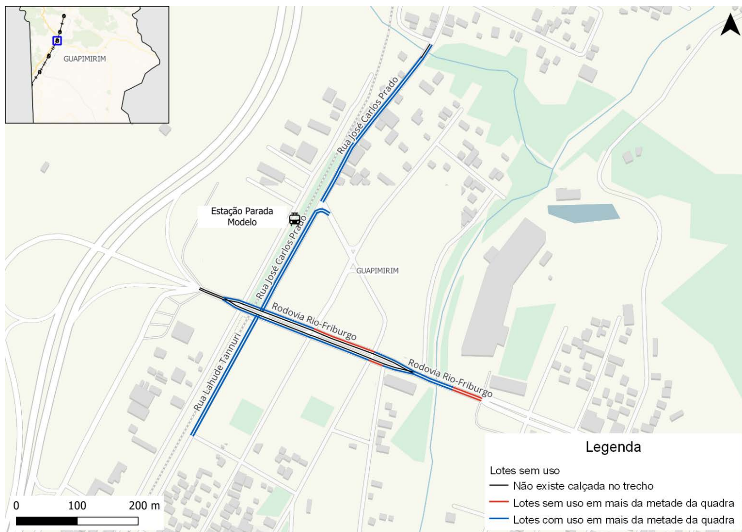
Figura 259: Lotes em uso para a rede inventariada de Parada Modelo
