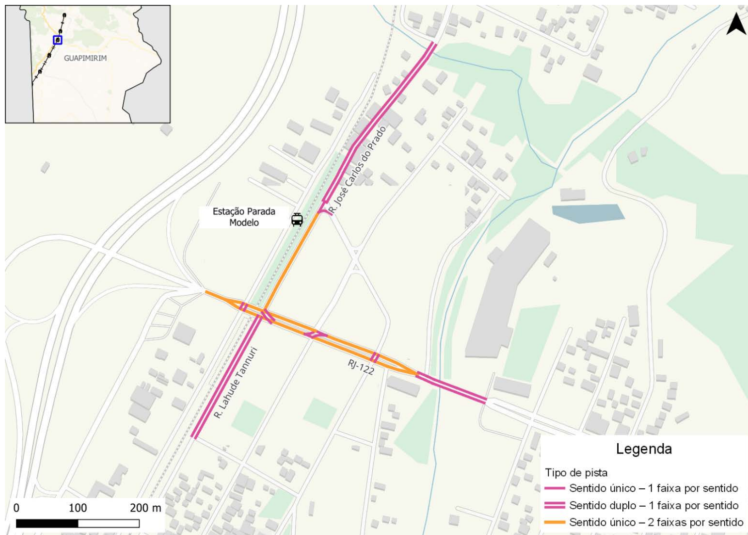
Figura 239: Tipo de pista e número de faixas por sentido na rede inventariada de Parada Modelo
