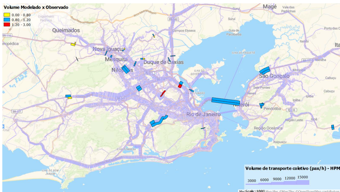
Figura 66: Volume de passageiros no Transporte Público – HPM
