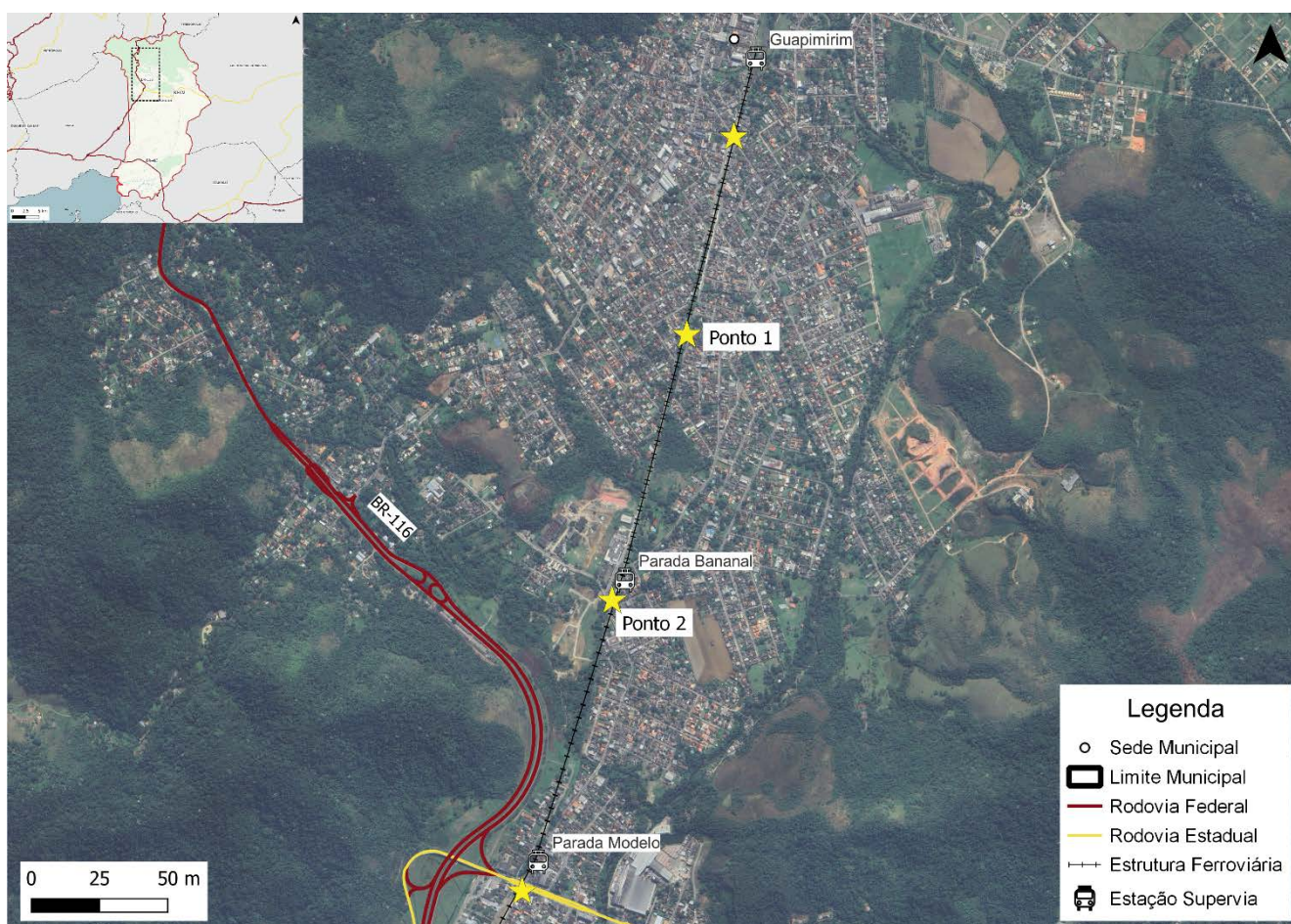
Figura 101: Interrupções viárias causadas pela linha ferroviária
