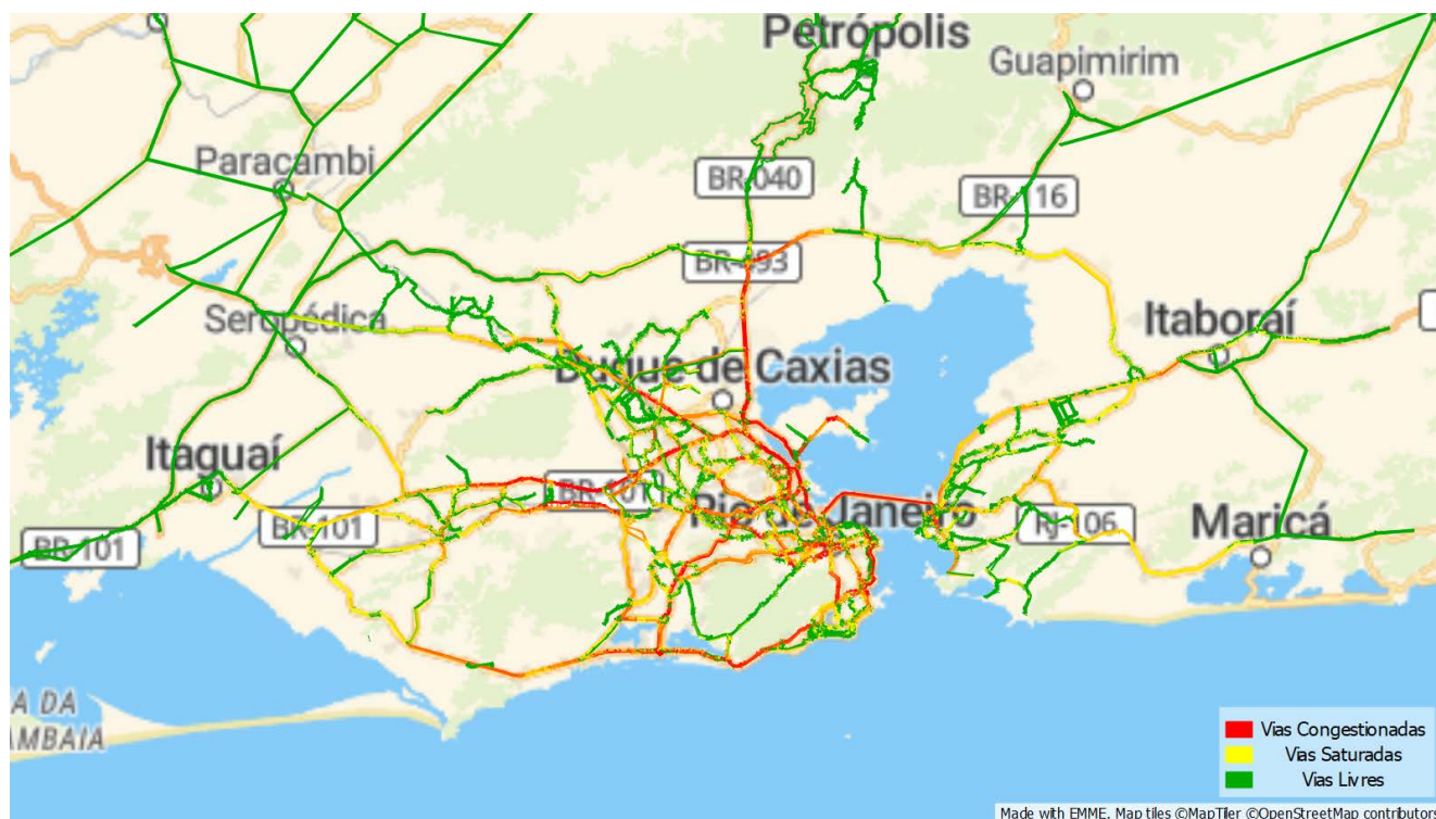
Figura 155: Nível de saturação do sistema viário metropolitano no cenário de prognóstico no horizonte de 10 anos
