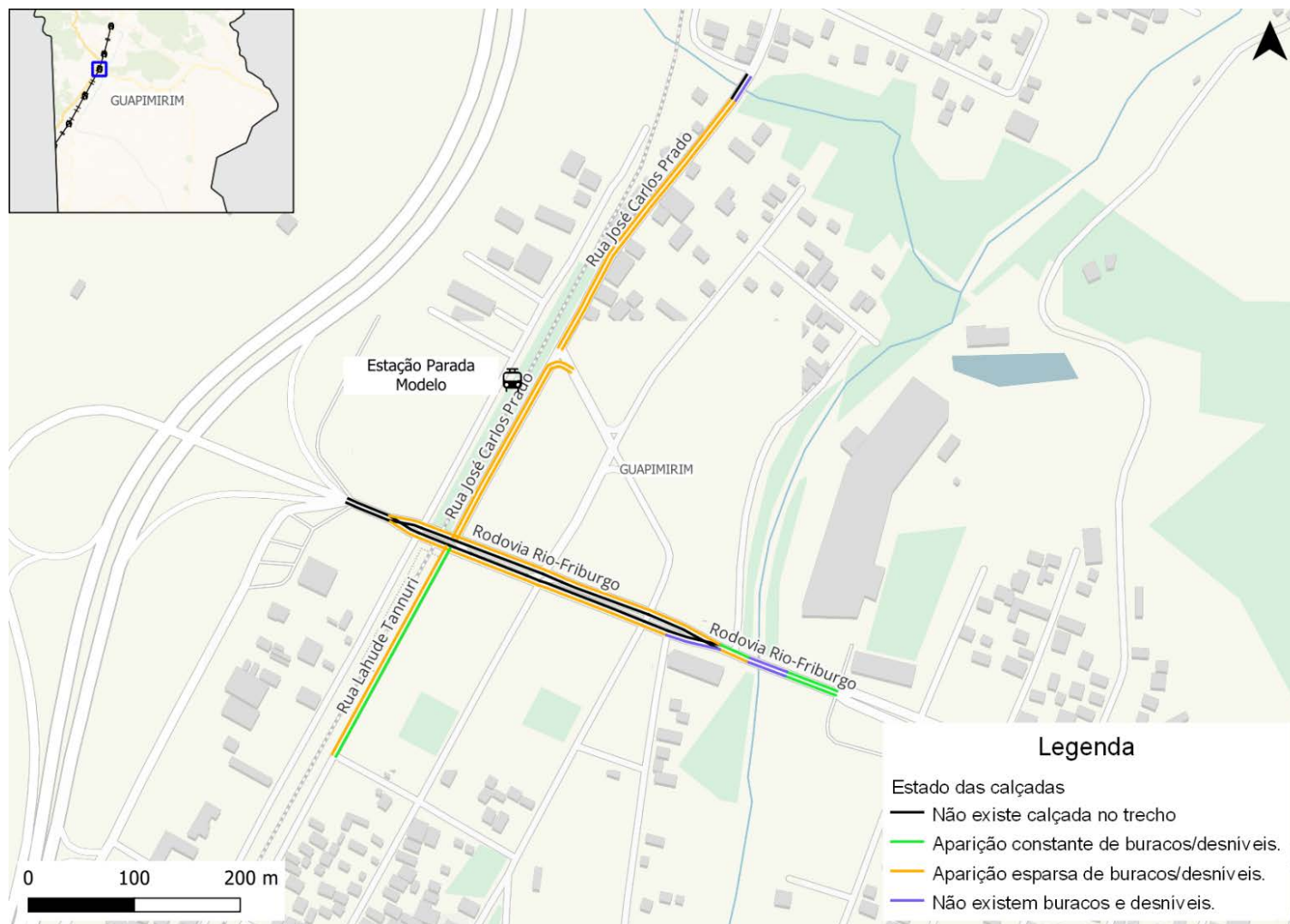
Figura 253: Existência de buracos e desníveis nas calçadas da rede inventariada de Parada Modelo
