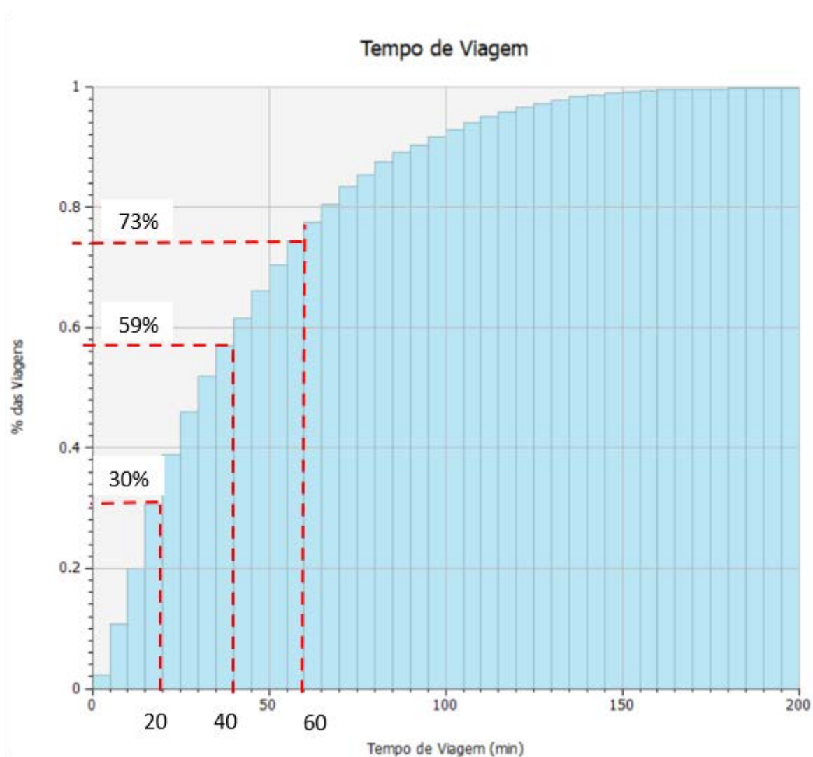
Figura 86: Histograma do tempo de viagem dos usuários do transporte privado na RMRJ
