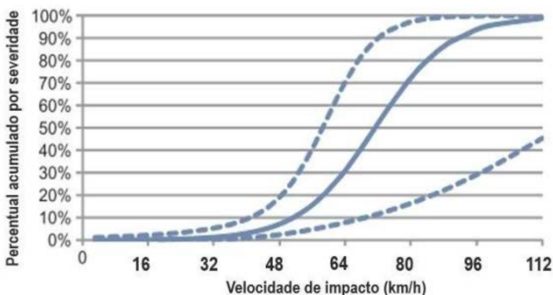
Figura 217: Probabilidade de fatalidades em atropelamentos em relação à velocidade do condutor no momento do acidente 41
