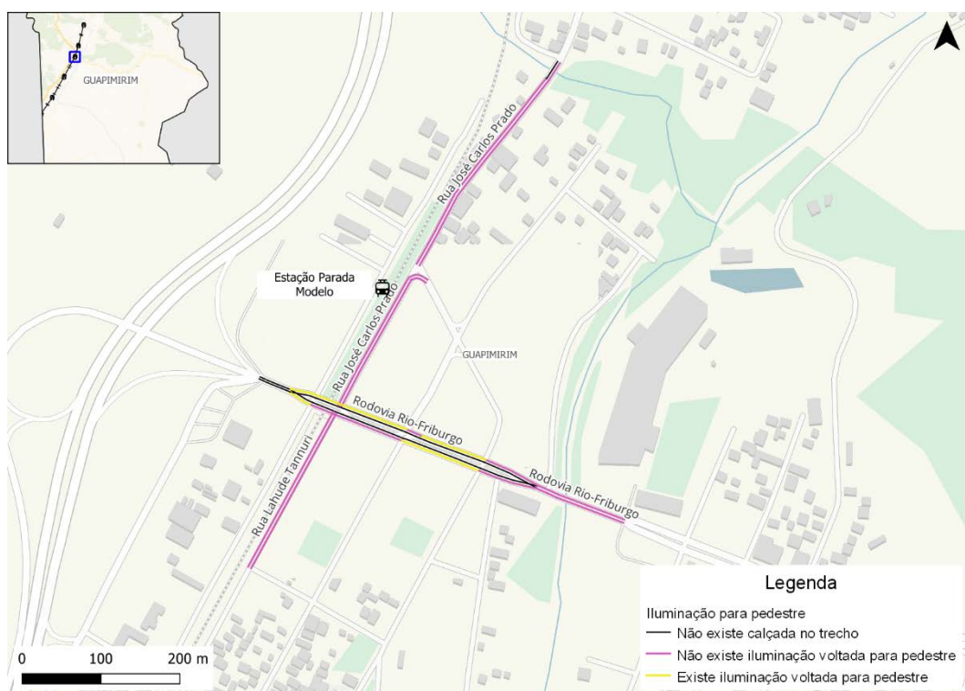
Figura 132: Iluminação pública exclusiva para pedestre
