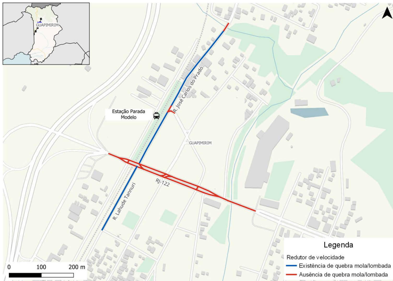
Figura 244: Elementos de redução de velocidade na rede inventariada de Parada Modelo
