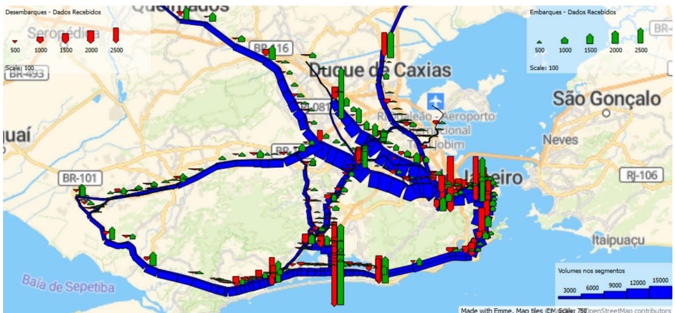
Figura 68: Volume de passageiros no sistema estruturante SuperVia, Metro e BRTs – HPM
