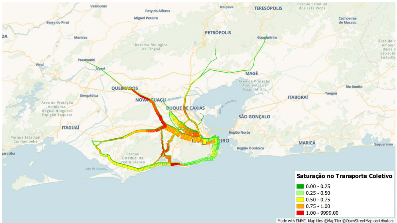
Figura 89: Nível de saturação no sistema de transporte estruturante de alta capacidade
