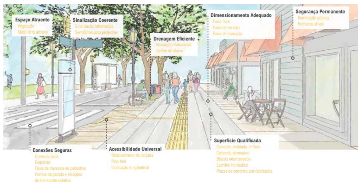
Figura 18: Esquema ilustrativo de calçada ideal
