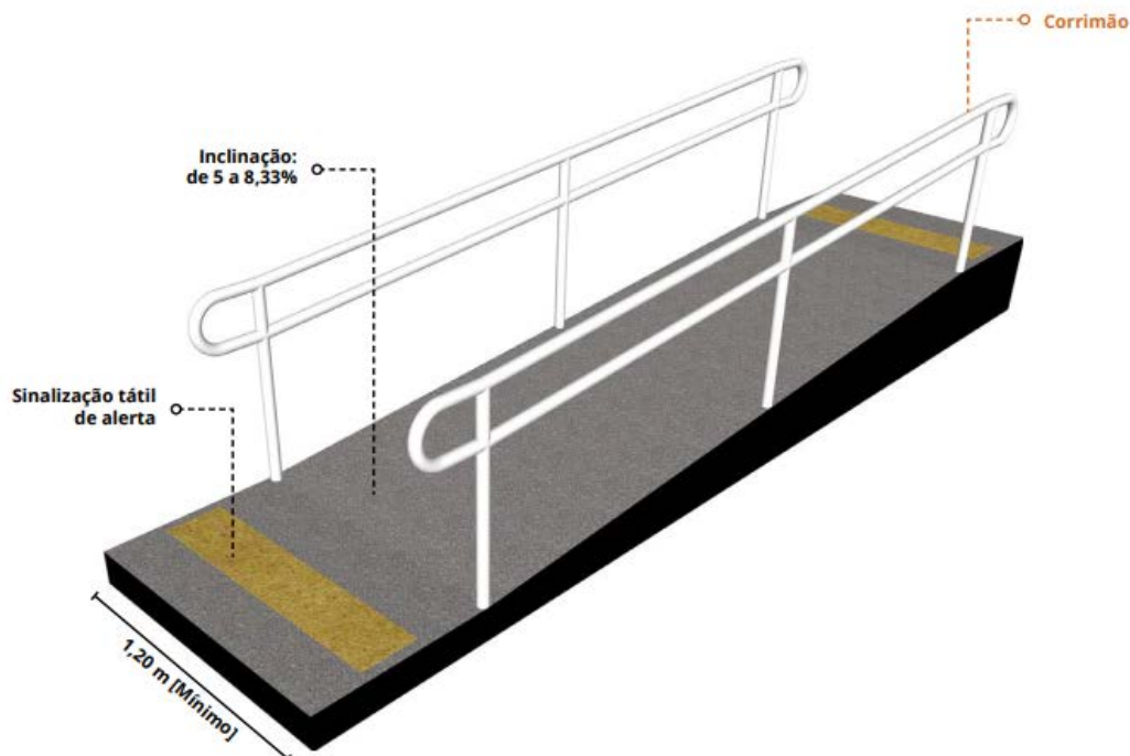
Figura 187: Exemplo de material encontrado no Caderno Técnico de Mobilidade Ativa
