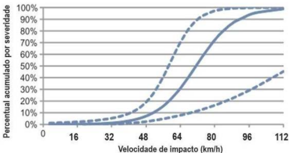
Figura 225: Probabilidade de fatalidades em atropelamentos em relação à velocidade do condutor no momento do acidente. 30
