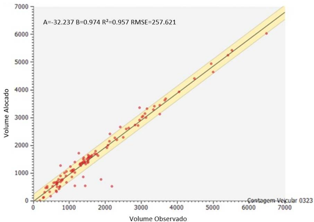
Figura 77: Gráfico do volume alocado x observado para transporte privado
