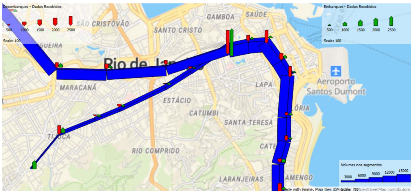
Figura 70: Volume de passageiros no metrô – zoom na região central
