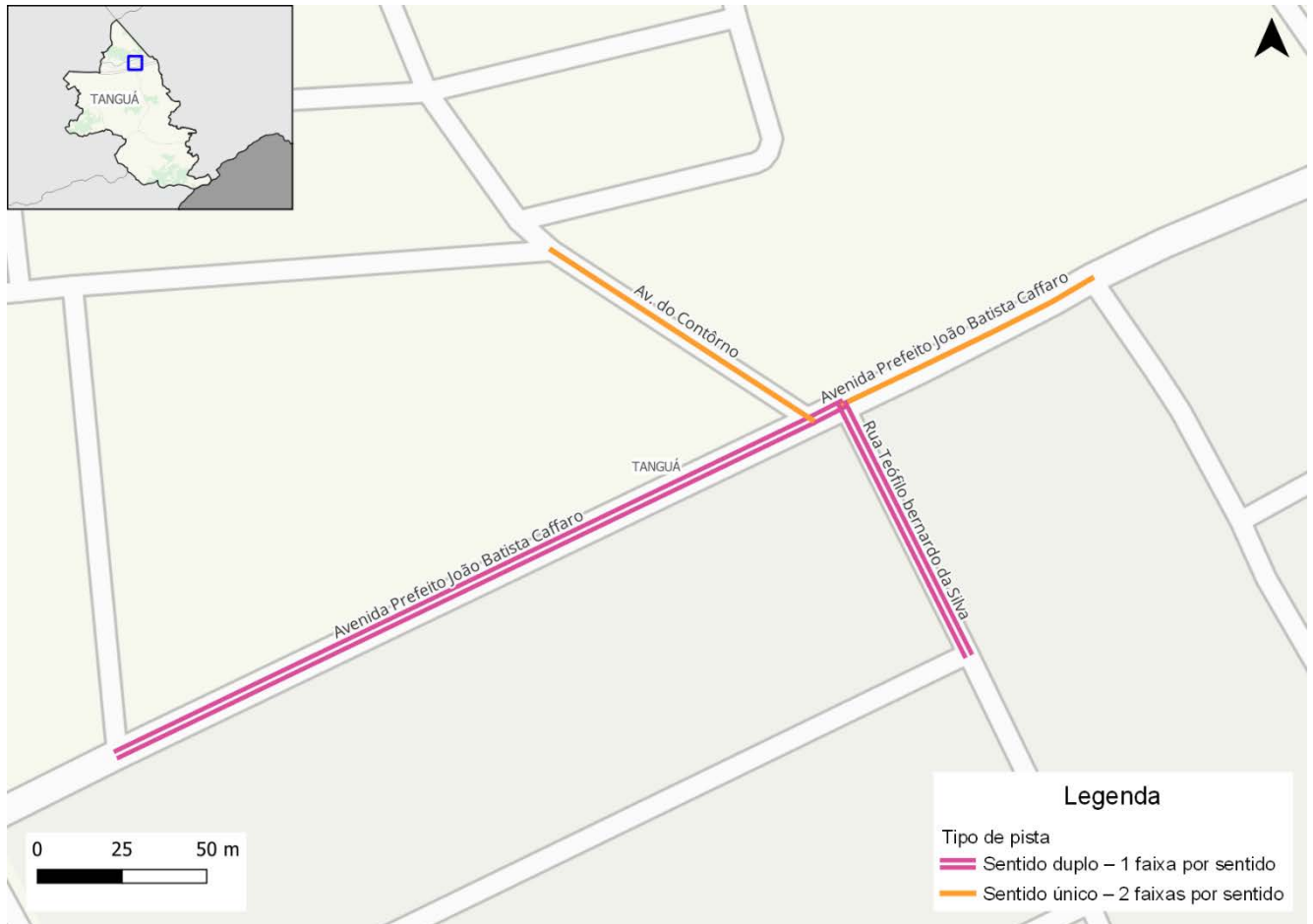
Figura 113: Tipo de pista na região central de Tanguá
