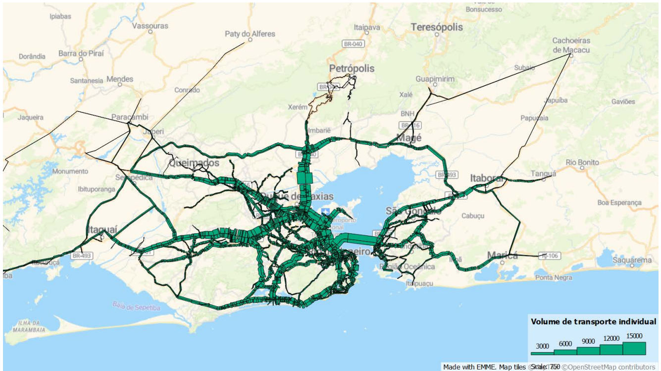
Figura 175: Carregamento de transporte individual nos principais eixos metropolitanos, no cenário de prognóstico
