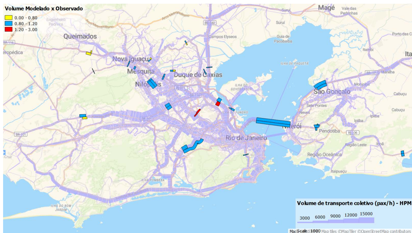
Figura 75: Volume de passageiros no Transporte Público – HPM
