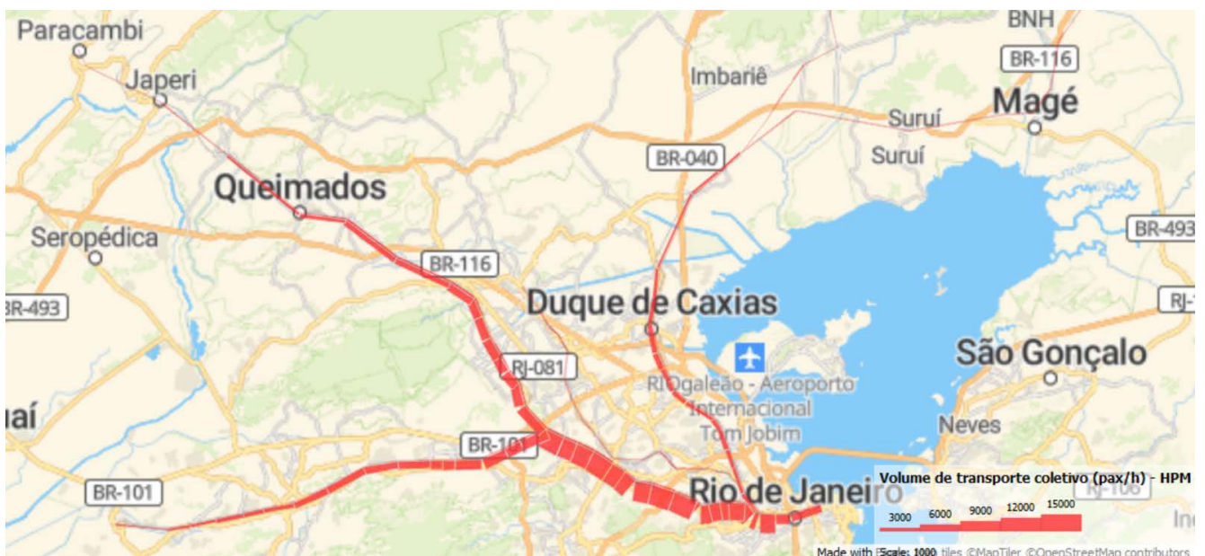
Figura 85: Carregamento da SuperVia na HPM
