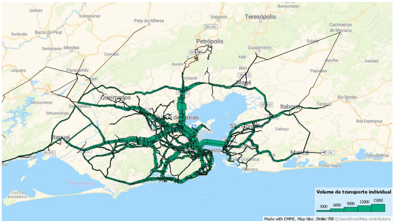
Figura 78: Carregamento de transporte individual nos principais eixos metropolitanos
