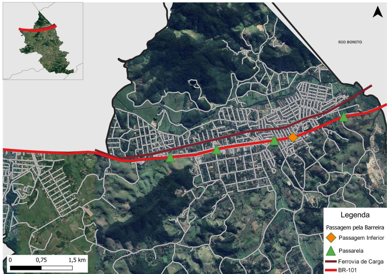
Figura 109: Traçado da ferrovia e da BR-101 com a localização de passarelas
