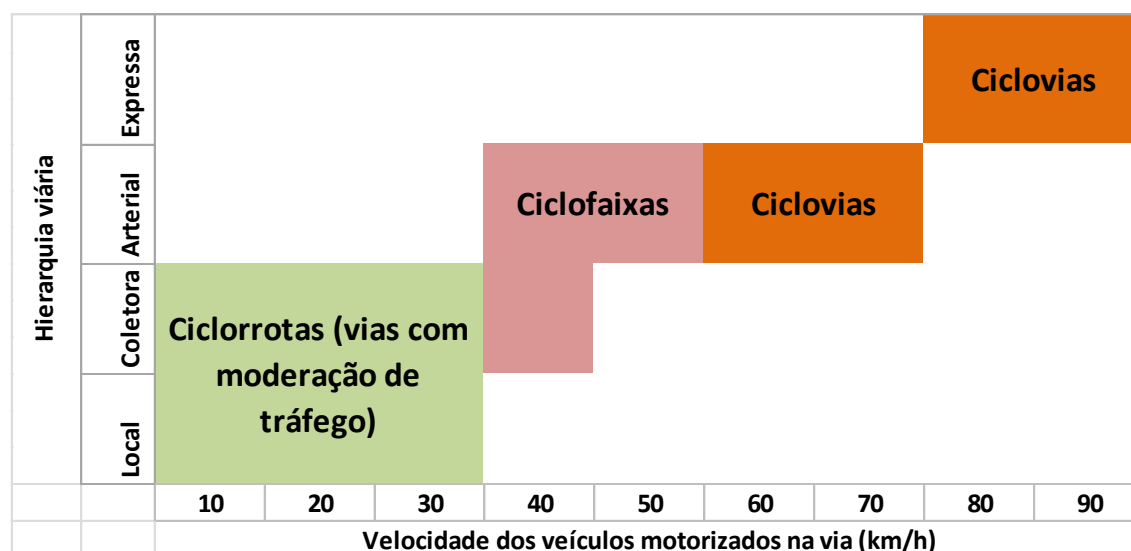
Figura 203: Tipologia de tratamento ciclovitário de acordo com hierarquia viária e velocidade da via
