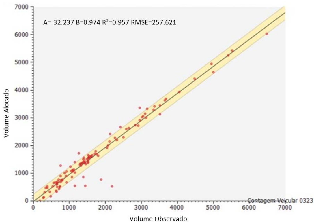
Figura 75: Gráfico do volume alocado x observado para transporte privado
