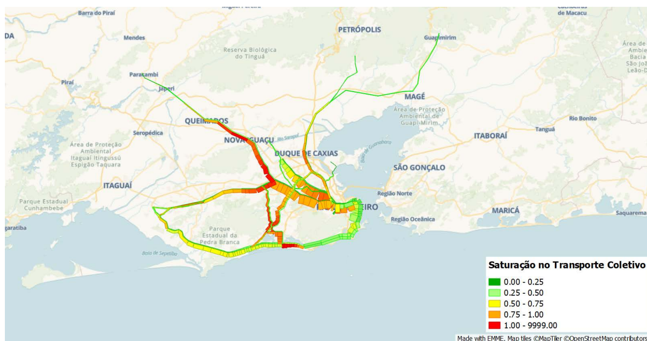
Figura 87: Nível de saturação no sistema de transporte estruturante de alta capacidade
