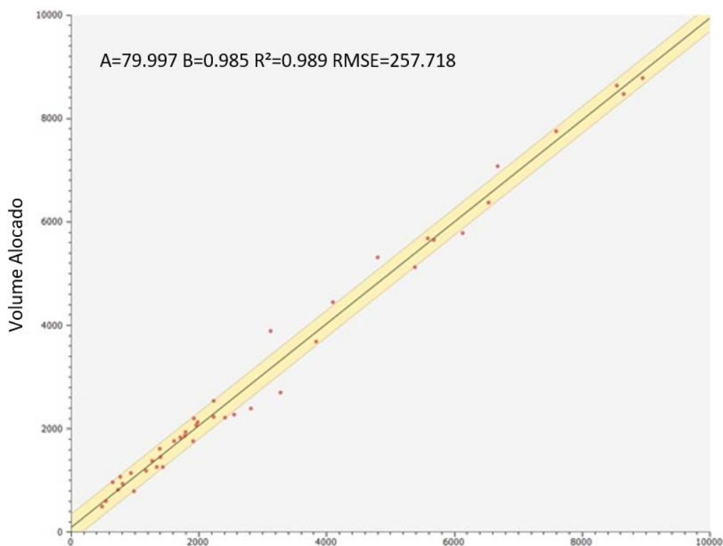
Figura 74: Gráfico do volume alocado x observado para transporte público
