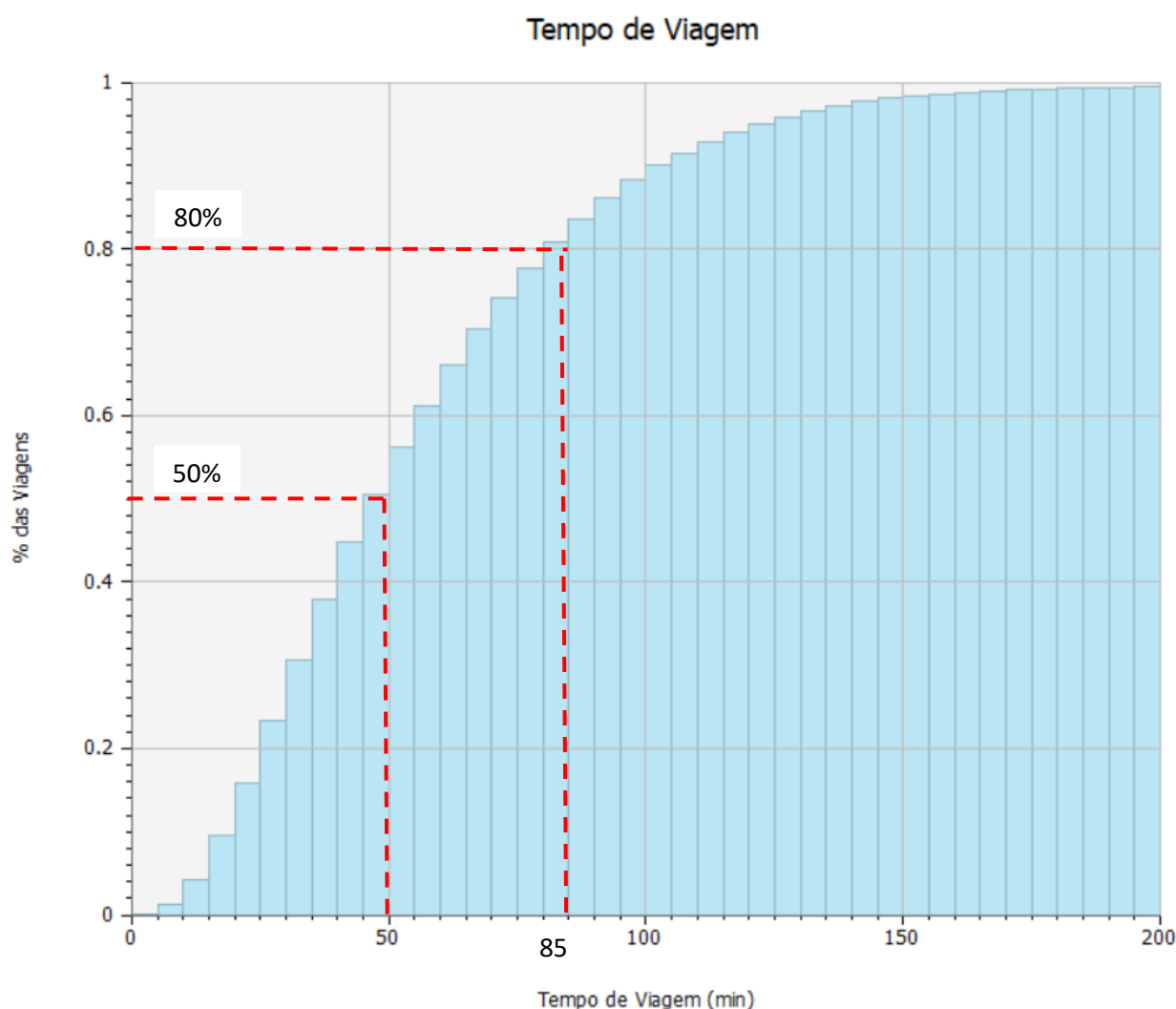
Figura 94: Histograma do tempo de viagem do transporte coletivo na RMRJ
