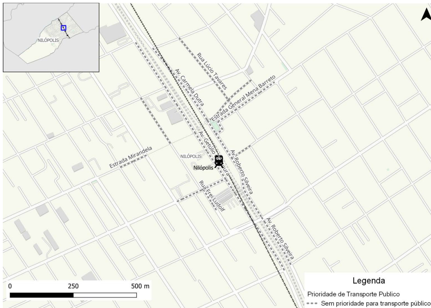
Figura 238: Tipo de preferência ao transporte coletivo na rede inventariada de Nilópolis
