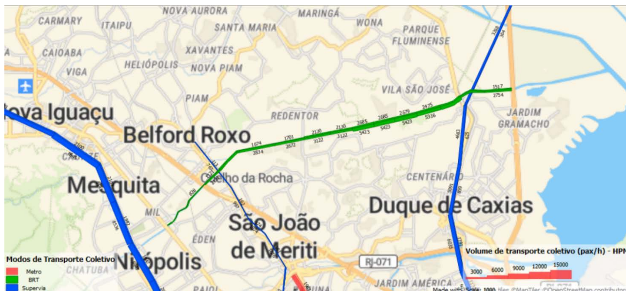
Figura 96: Carregamento TransBaixada, no horizonte de 2034
