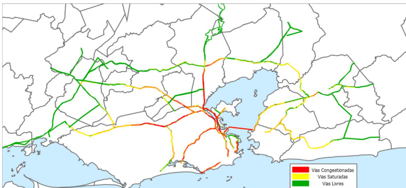
Figura 78: Nível de saturação do sistema viário metropolitano
