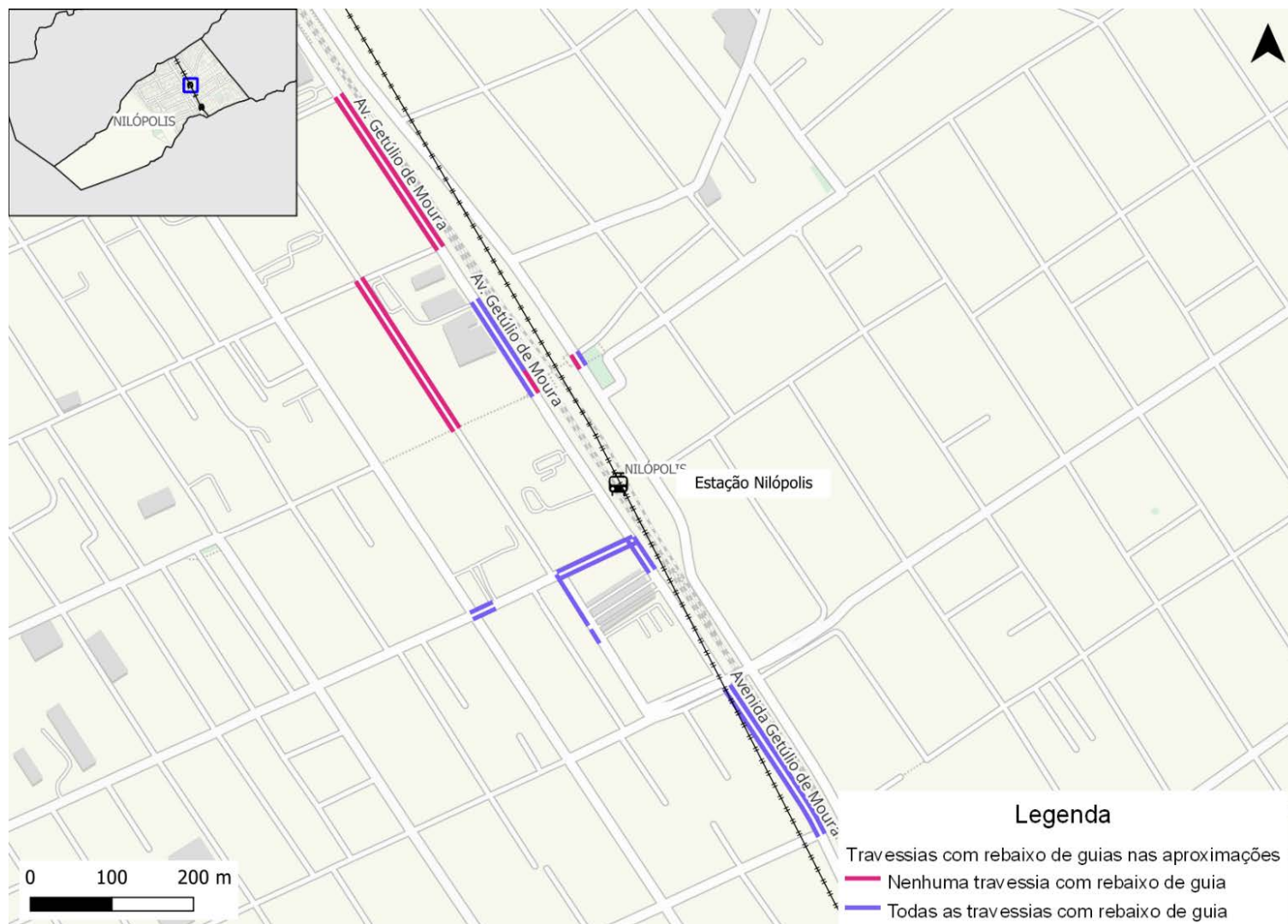
Figura 262: Travessias com rebaixo de guia nas aproximações na rede inventariada de Nilópolis
