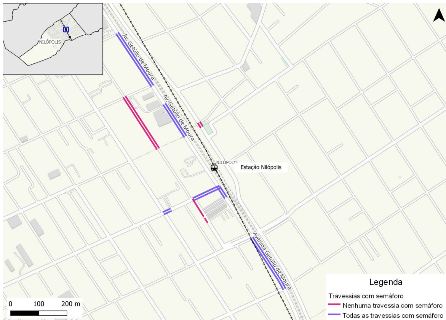
Figura 259: Travessias semaforizadas na rede inventariada de Nilópolis
