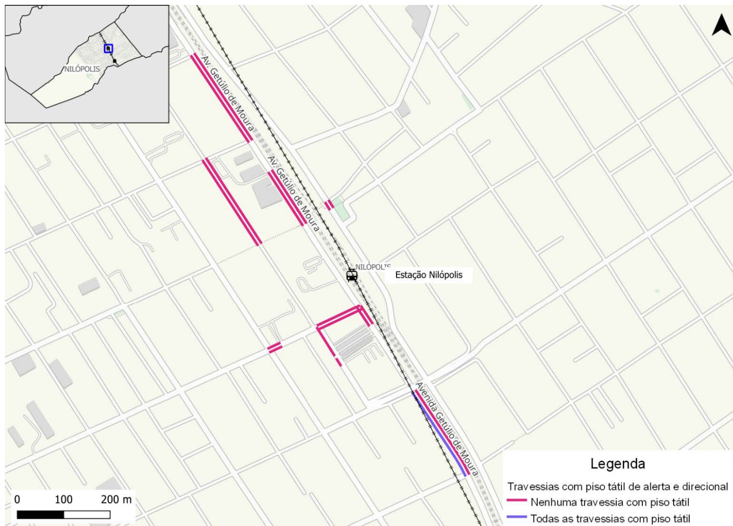
Figura 261: Travessias com piso tátil na rede inventariada de Nilópolis
