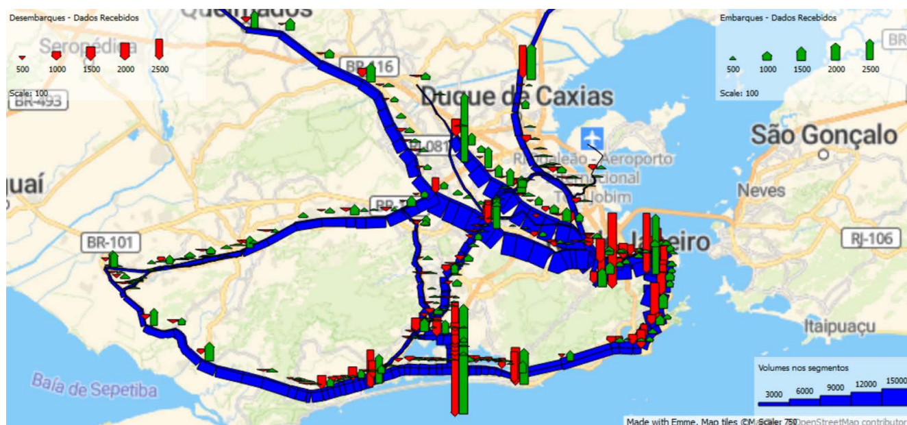
Figura 66: Volume de passageiros no sistema estruturante SuperVia, Metro e BRTs – HPM
