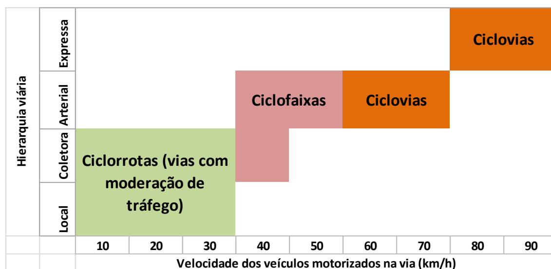
Figura 188: Tipologia de tratamento ciclovitário de acordo com hierarquia viária e velocidade da via
