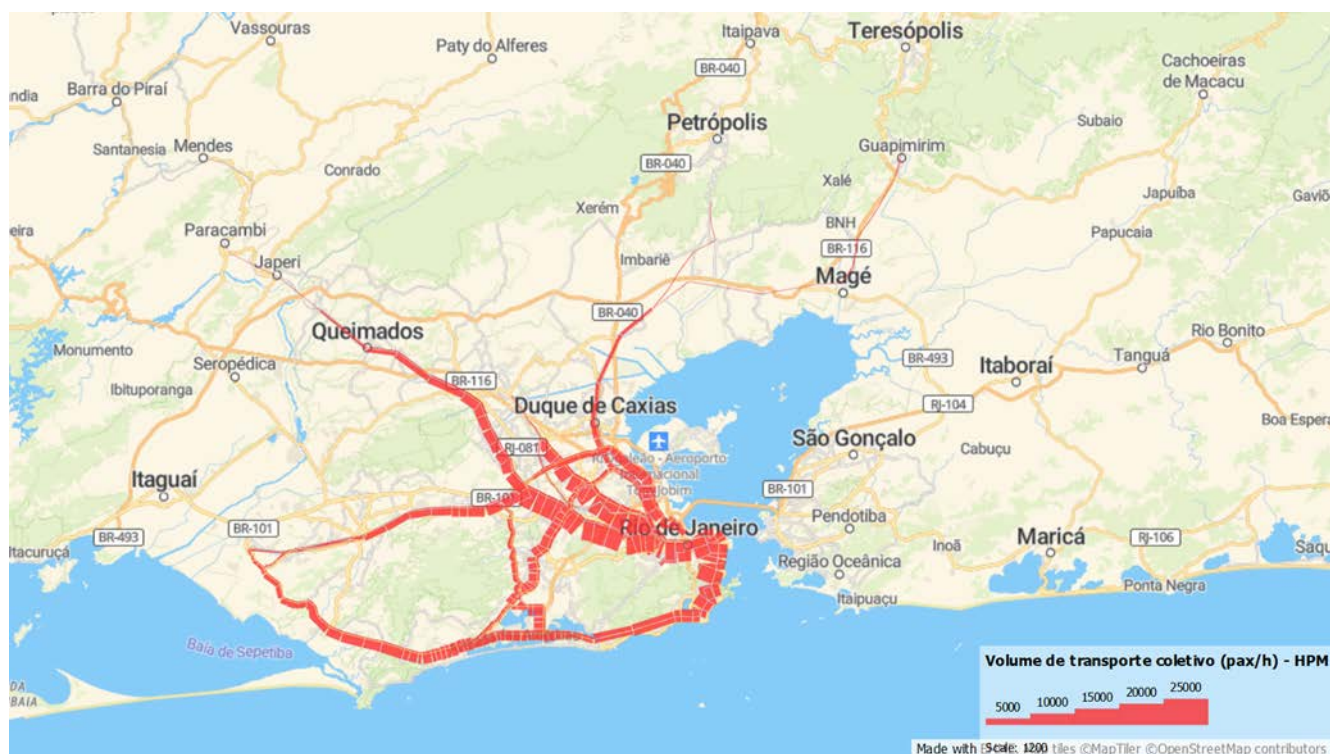
Figura 163: Volume de transporte coletivo na HPM, para o cenário de prognóstico no horizonte de 10 anos
