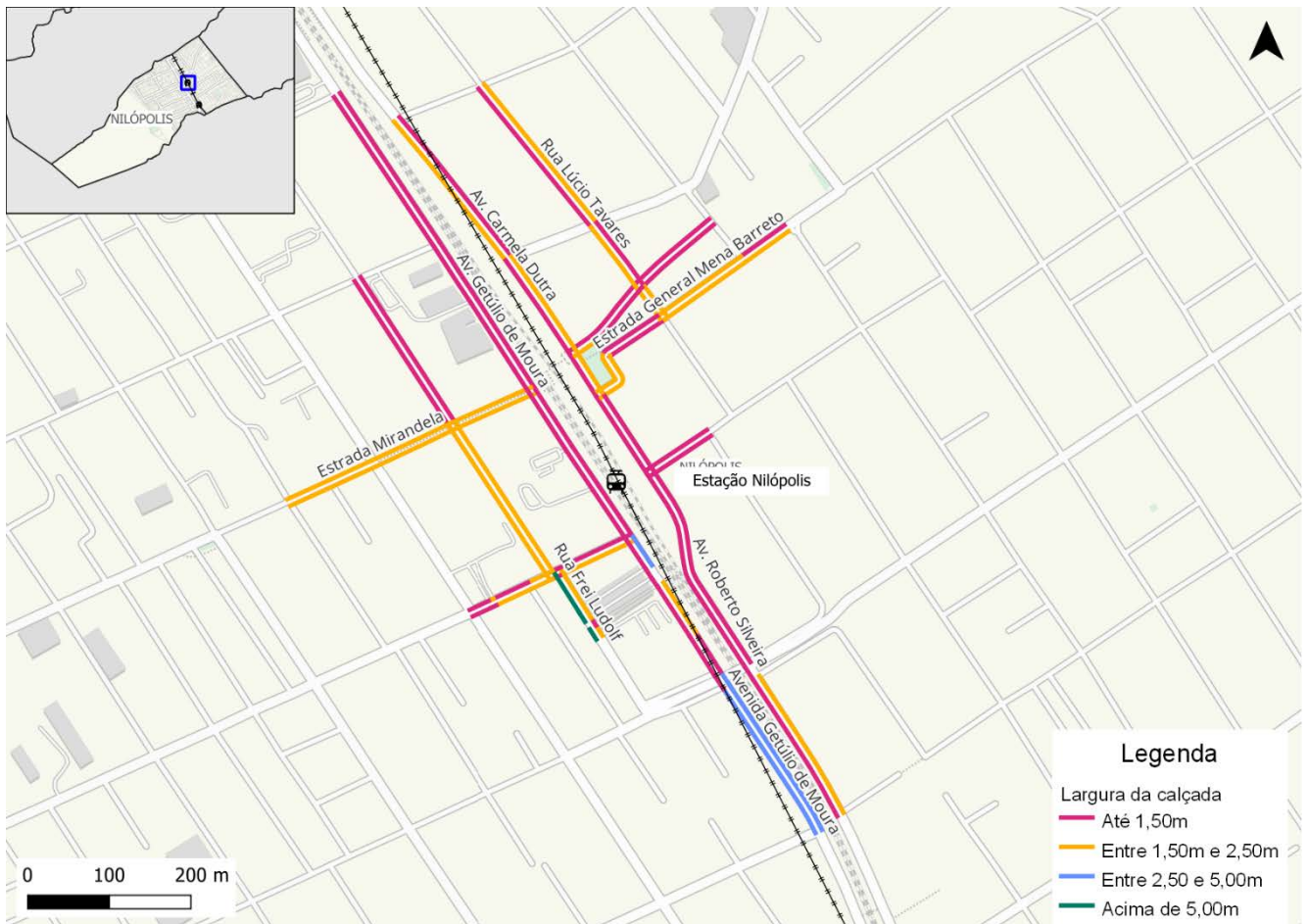
Figura 137: Largura das calçadas no entorno da estação de trem Nilópolis e Rodoviária
