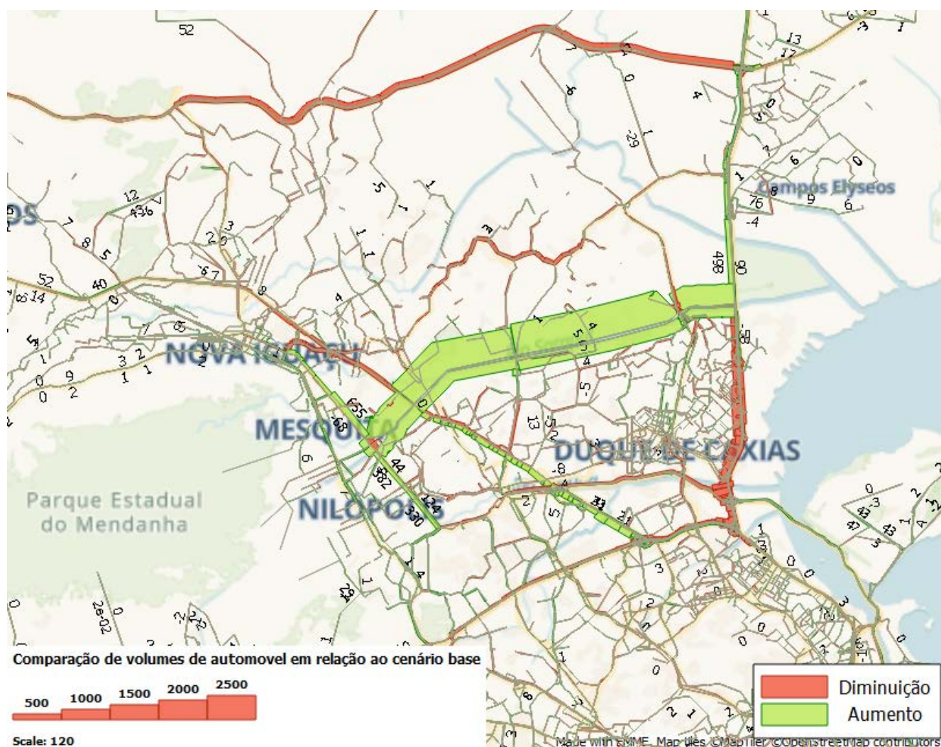
Figura 100: Comparação de volumes de automóvel no cenário base e no cenário da TransBaixada, no horizonte de 2034.
