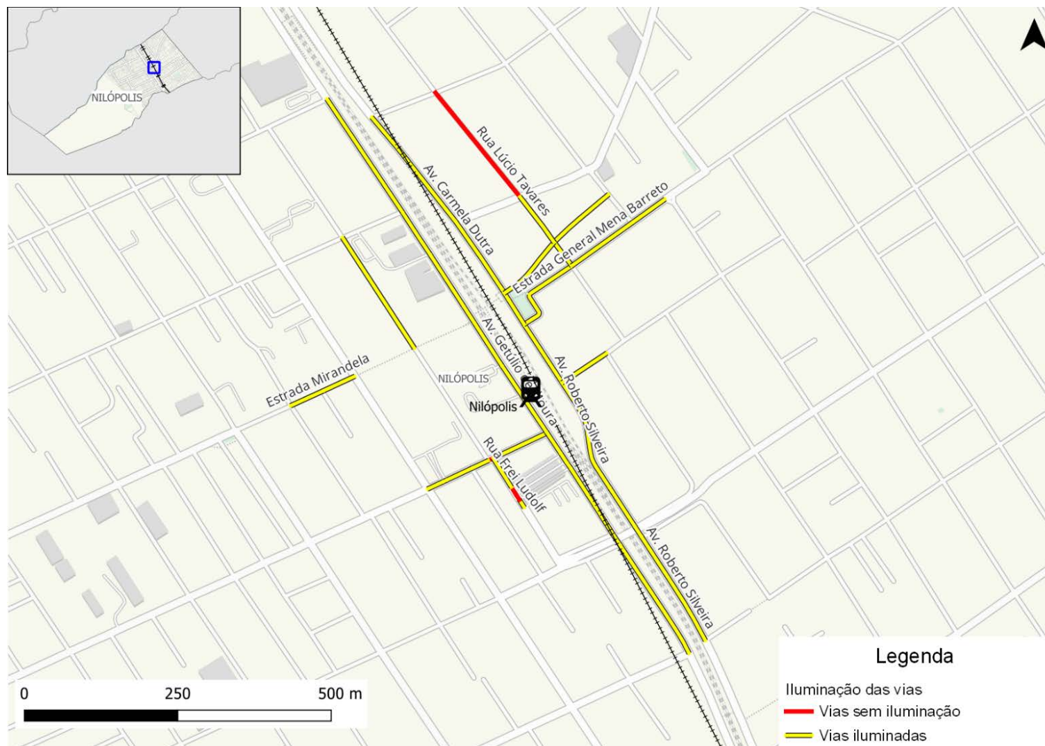
Figura 232: Iluminação viária na rede inventariada de Nilópolis
