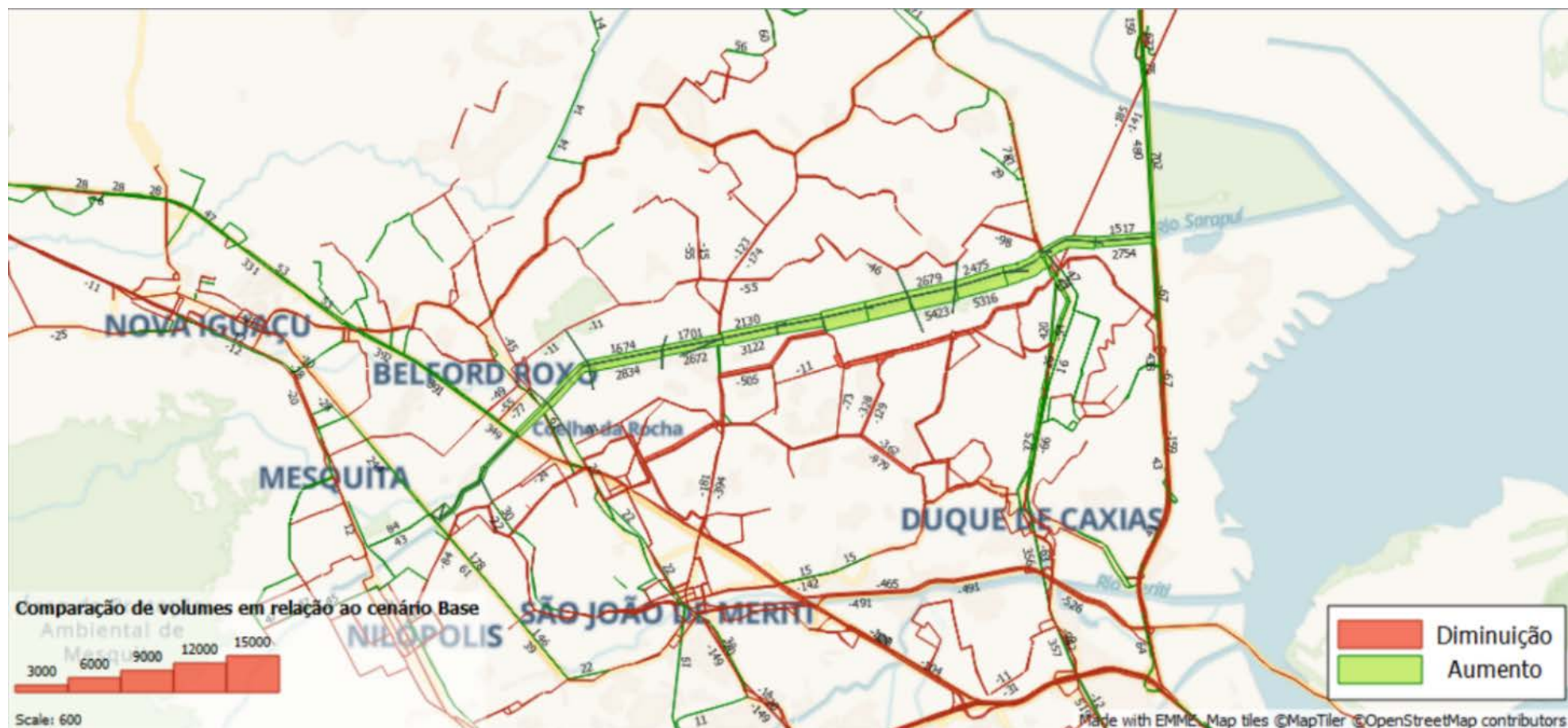
Figura 97: Comparação de volumes entre cenário Base e cenário com o BRT TransBaixada, no horizonte 2034
