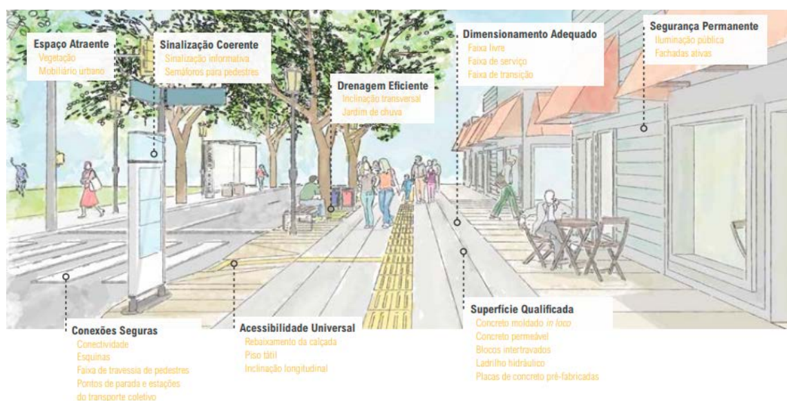
Figura 170: Esquema ilustrativo de calçada ideal
