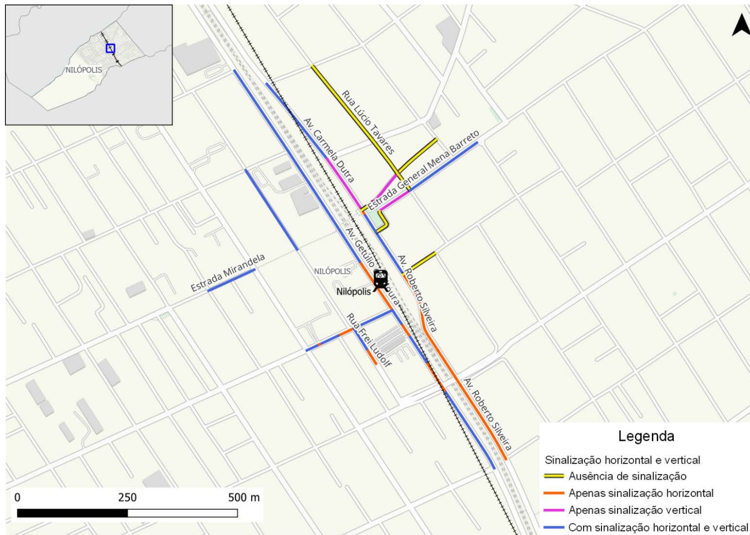
Figura 231: Existência de sinalização na rede inventariada de Nilópolis
