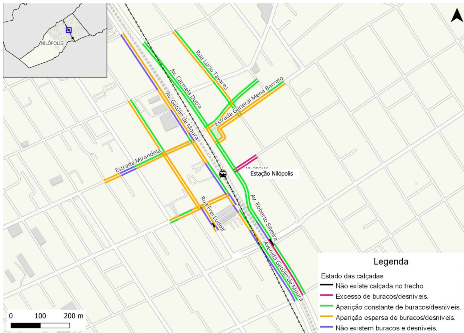
Figura 245: Existência de buracos e desníveis nas calçadas da rede inventariada de Nilópolis
