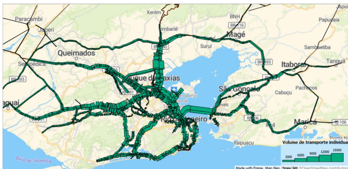
Figura 160: Carregamento de transporte individual nos principais eixos metropolitanos, no cenário de prognóstico
