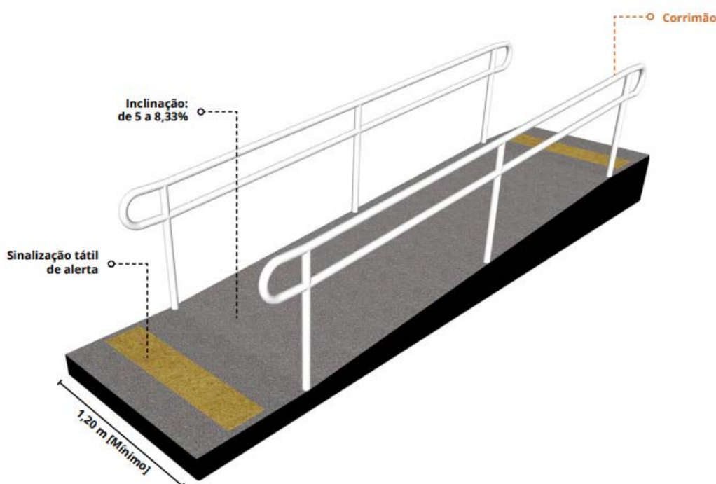
Figura 172: Exemplo de material encontrado no Caderno Técnico de Mobilidade Ativa
