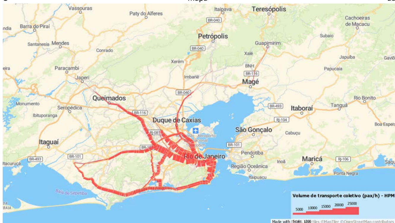
Figura 163 apresenta o carregamento dos sistemas estruturantes na RMRJ no cenário de prognóstico.
