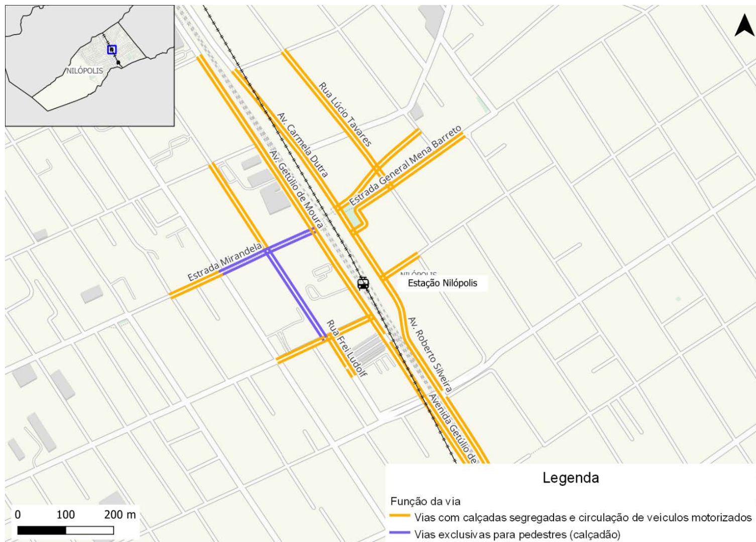
Figura 252: Função da via na rede inventariada de Nilópolis
