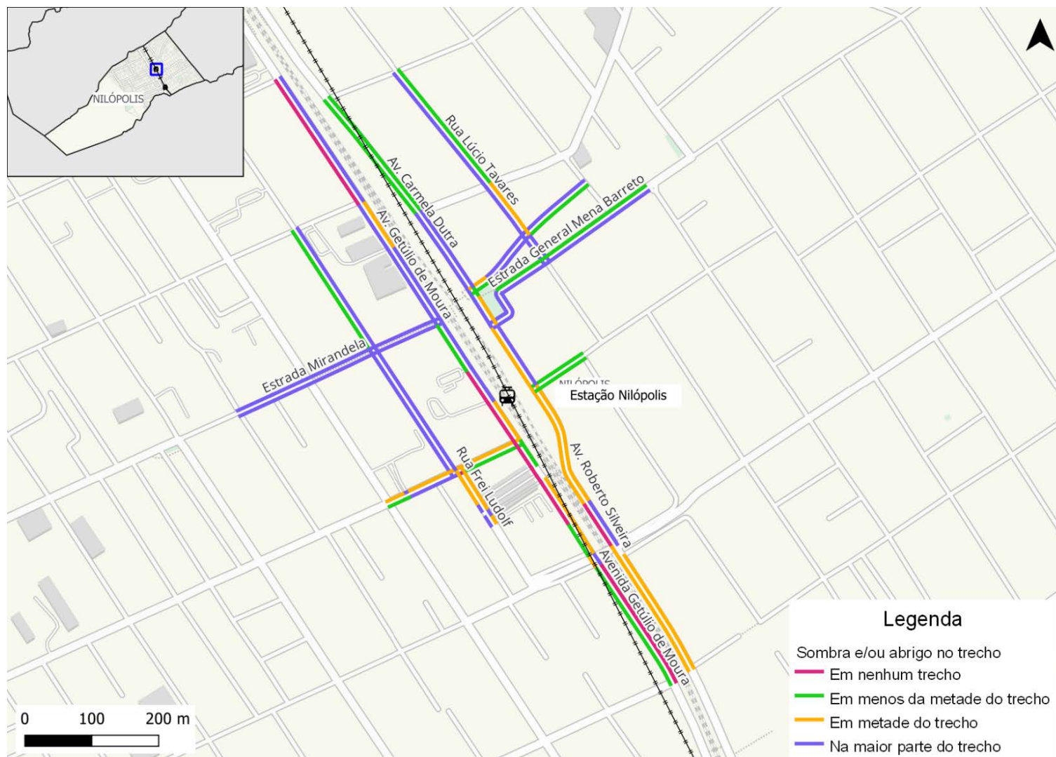
Figura 257: Presença de sombra e abrigo nas calçadas da rede inventariada de Nilópolis
