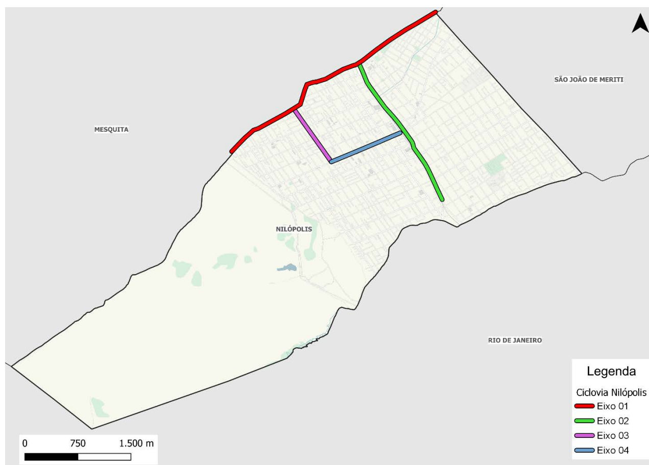
Figura 189: Recomendação de eixos cicloviários em Nilópolis
