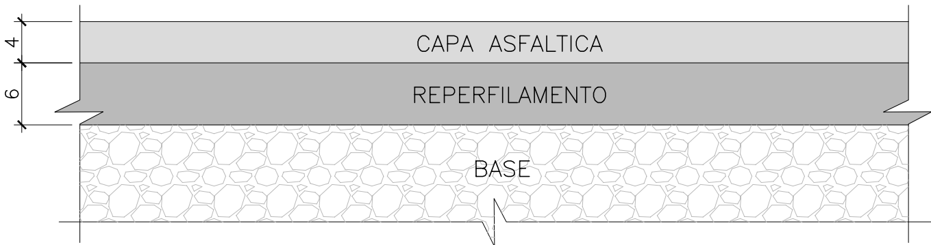
SEÇÃO TIPO DO PAVIMENTO
