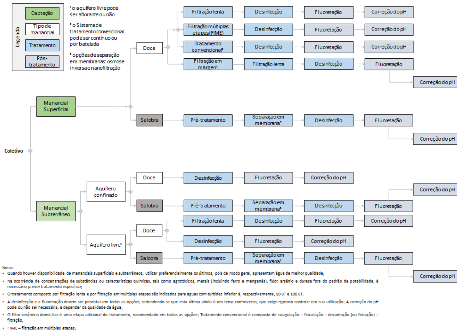
Figura 7-2 – Matriz tecnológica das soluções coletivas de abastecimento de água
