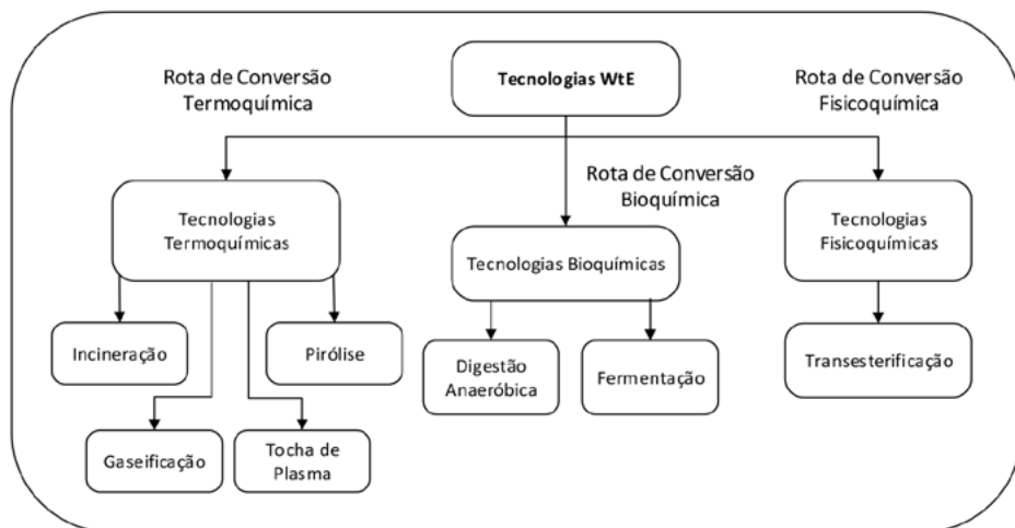
Figura 58: Classificação das Tecnologias WtE em Relação aos Caminhos de Conversão
