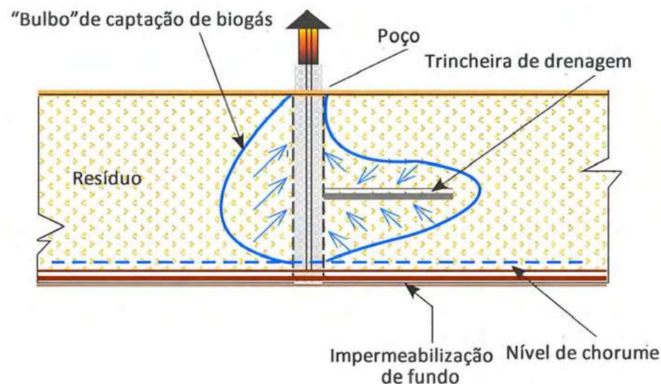
Figura 59: Esquema de Produção de Gás do Lixo e Chorume
