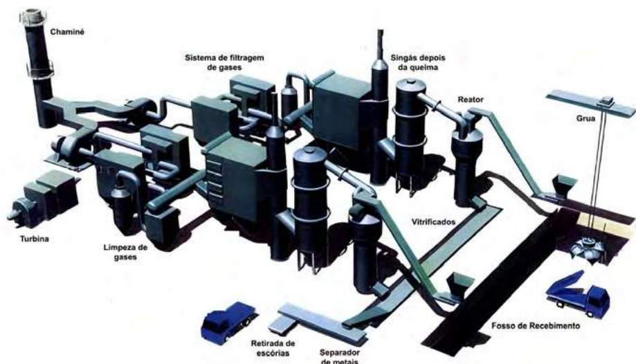
Figura 64: Esquema de uma Planta de Tocha de Plasma
