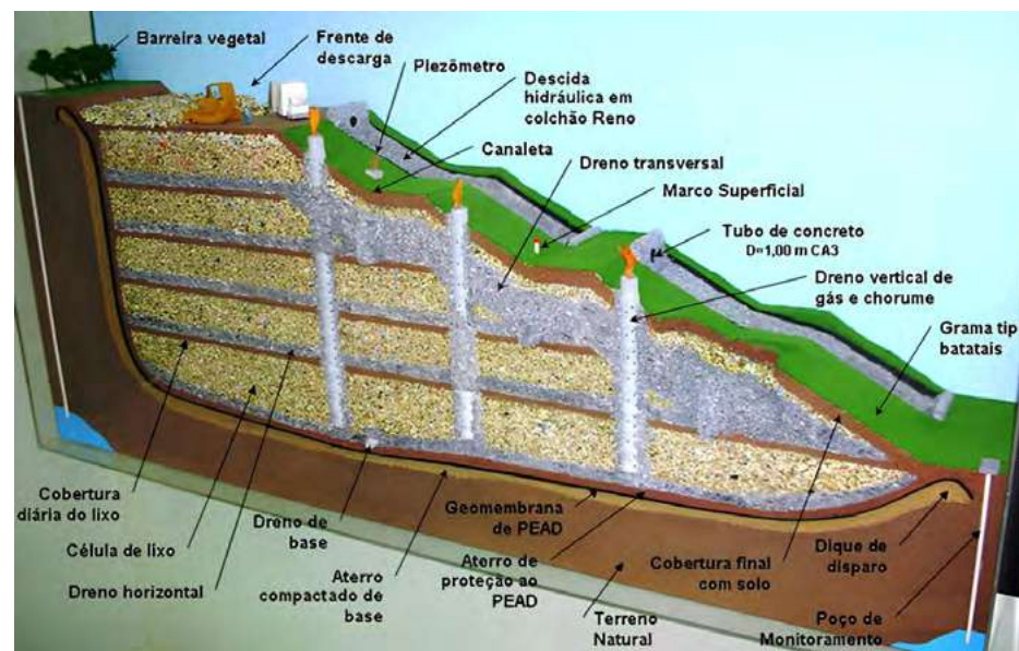
Figura 20: Principais Sistemas de Infraestrutura do Aterro Sanitário
