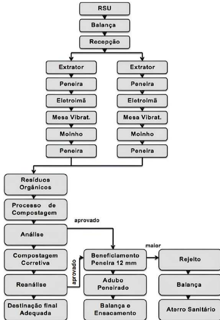
Figura 28: Fluxo dos Resíduos no Sistema de Compostagem
