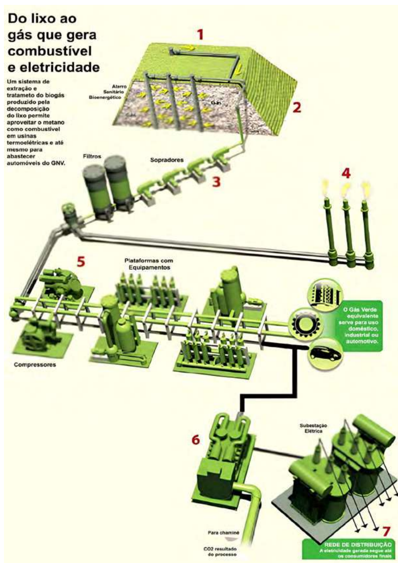
Figura 60: Planta de Produção, Tratamento e Conversão de Biogás do RSU
