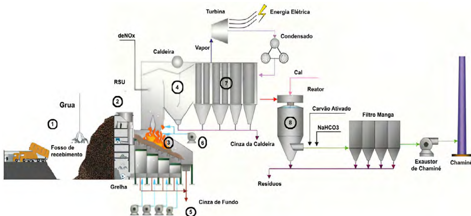
Figura 62: Fluxograma do Processo de Incineração
