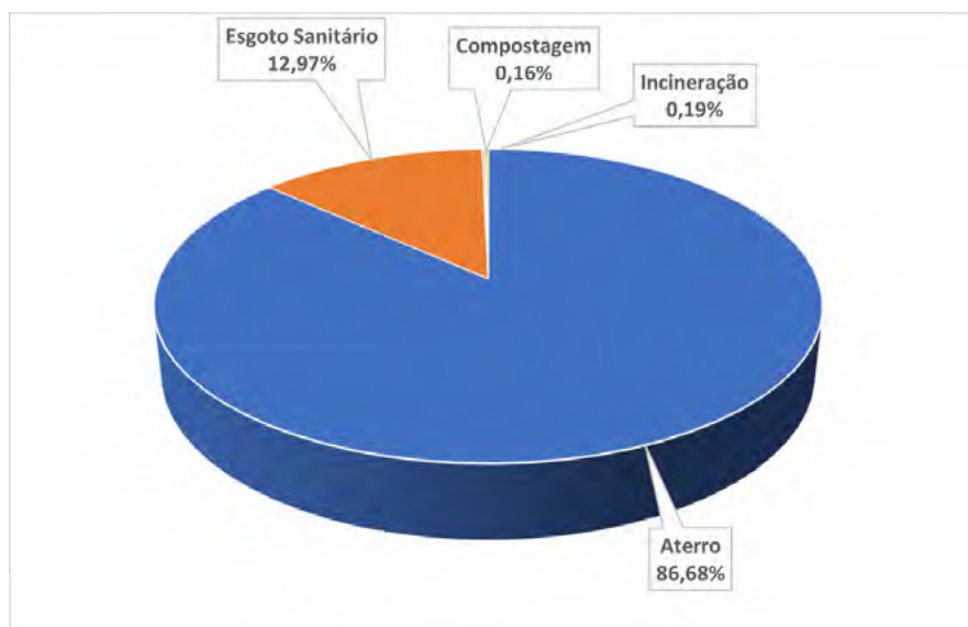
Figura 57: Setores Geradores de Gases de Efeito (GEE) – RSU
