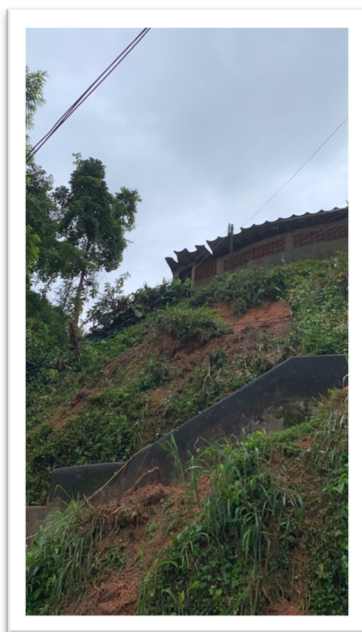
Figura 1 – Vista frontal do talude comprometido com sinais de carreamento de material granular e escorregamento parcial de massa
