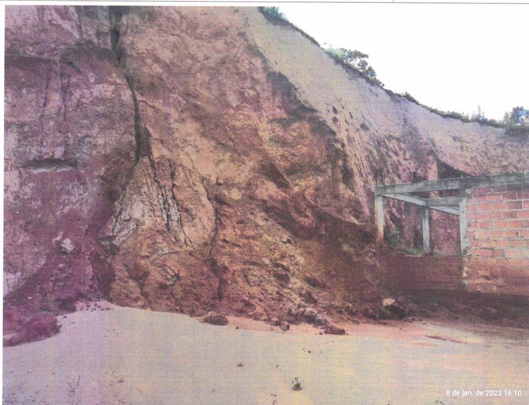
Foto 4 - Escorregamento atingindo parte da construção e do lote vizinho.
