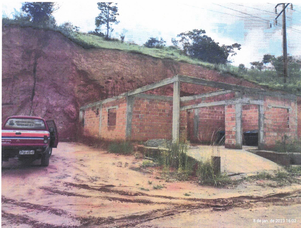
Foto 3 – “Esqueleto” de uma obra residencial, localizada um lote após o número 70 da Rua Orcina Medeiros Jorge, construção feita distando aproximadamente, 3m do talude.
