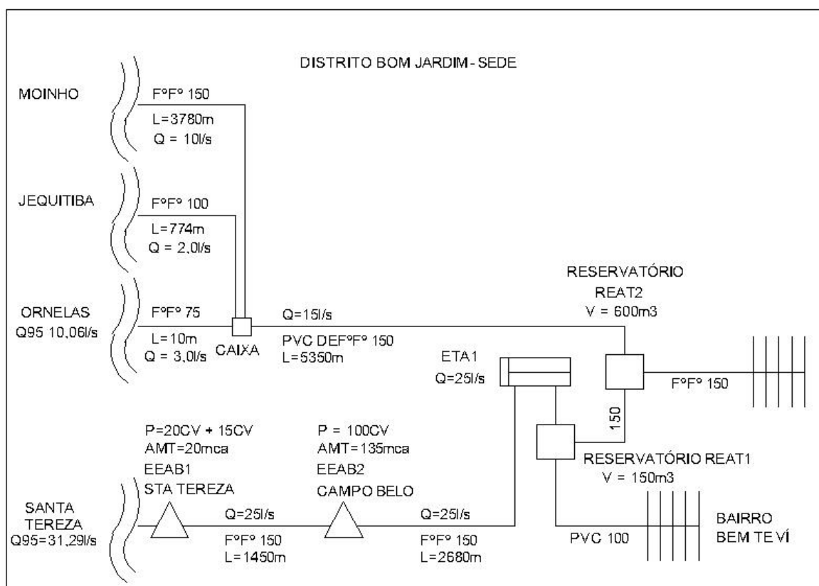
Figura 9: Diagrama simplificado SAA da Sede - Bom Jardim
