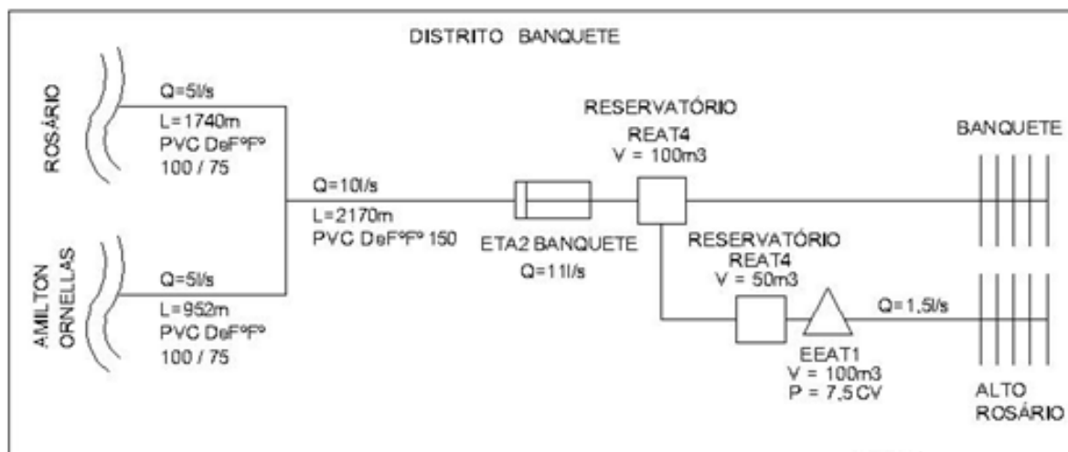
Figura 10: Diagrama simplificado do Sistema Banquete
