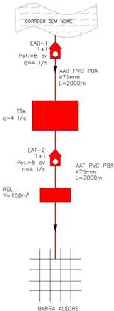
Figura 15 - Diagrama simplificado do Sistema Barra Alegre.
