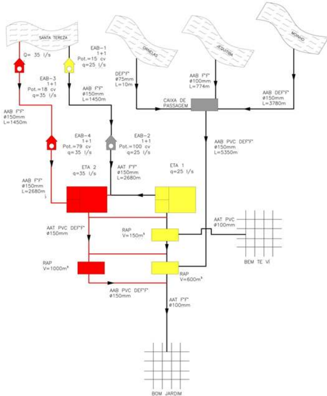
Figura 12 - Diagrama simplificado do Sistema Sede
