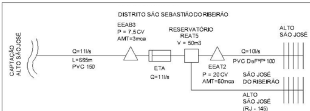
Figura 11: Diagrama simplificado do Sistema São José do Ribeirão
