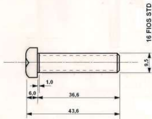
PARAFUSO COM ROSCA TOTAL
