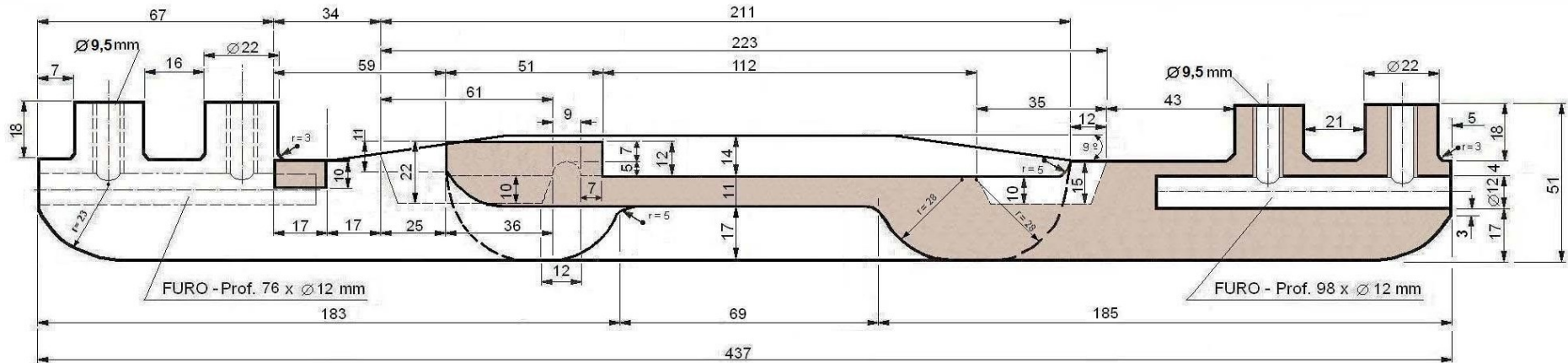
CORTE A - A' LONGITUDINAL
