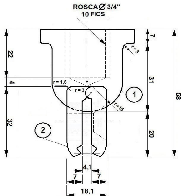
VISTA FRONTAL - PEÇAS 1 e 2 LADO DIREITO E ESQUERDO COMPONENTES UNIDOS PARA PARAFUSOS ALLEN MODELO 4
