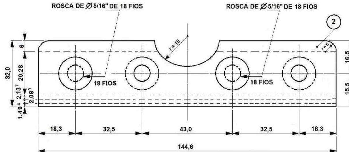
VISTA LATERAL - PEÇA 2 COMPONENTE DO LADO ESQUERDO PARA PARAFUSOS ALLEN MODELO 4
