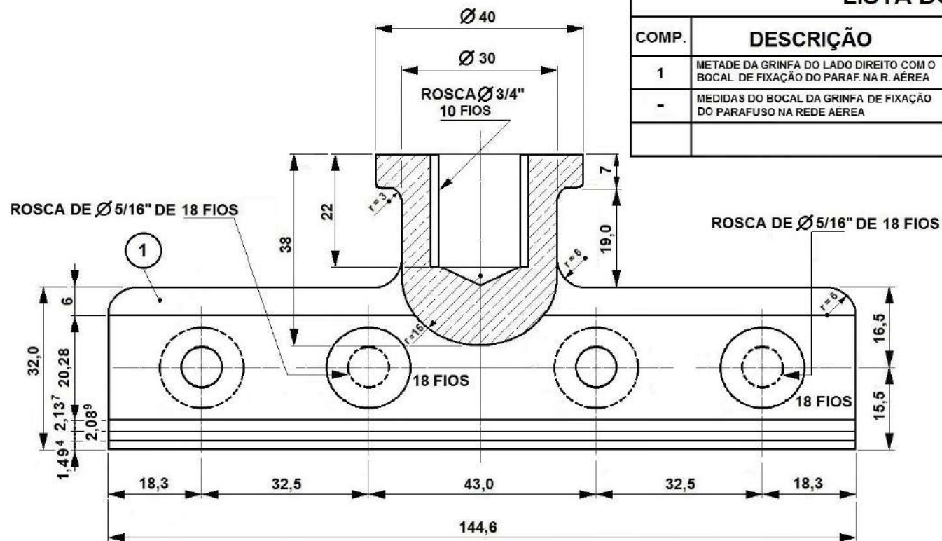
VISTA LATERAL - PEÇA 1 COMPONENTE DO LADO DIREITO PARA PARAFUSOS ALLEN MODELO 4 E CORTE PARCIAL A - A
