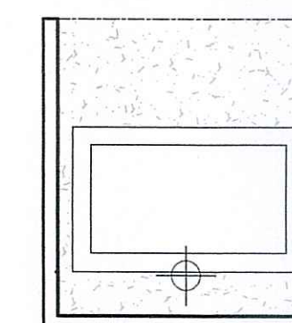
DETALHE REATERRO DE VALA PARA IMPLANTAÇÃO DE TUBULAÇÃO
