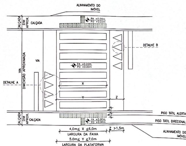
01 FAIXA ELEVADA PARA TRAVESSIA ESC.: 1:100
