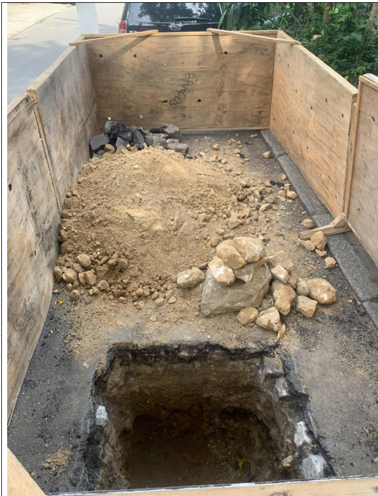
Foto 10: Sondagem realizada para identificação do tipo de solo antes do assentamento da tubulação de gás.
