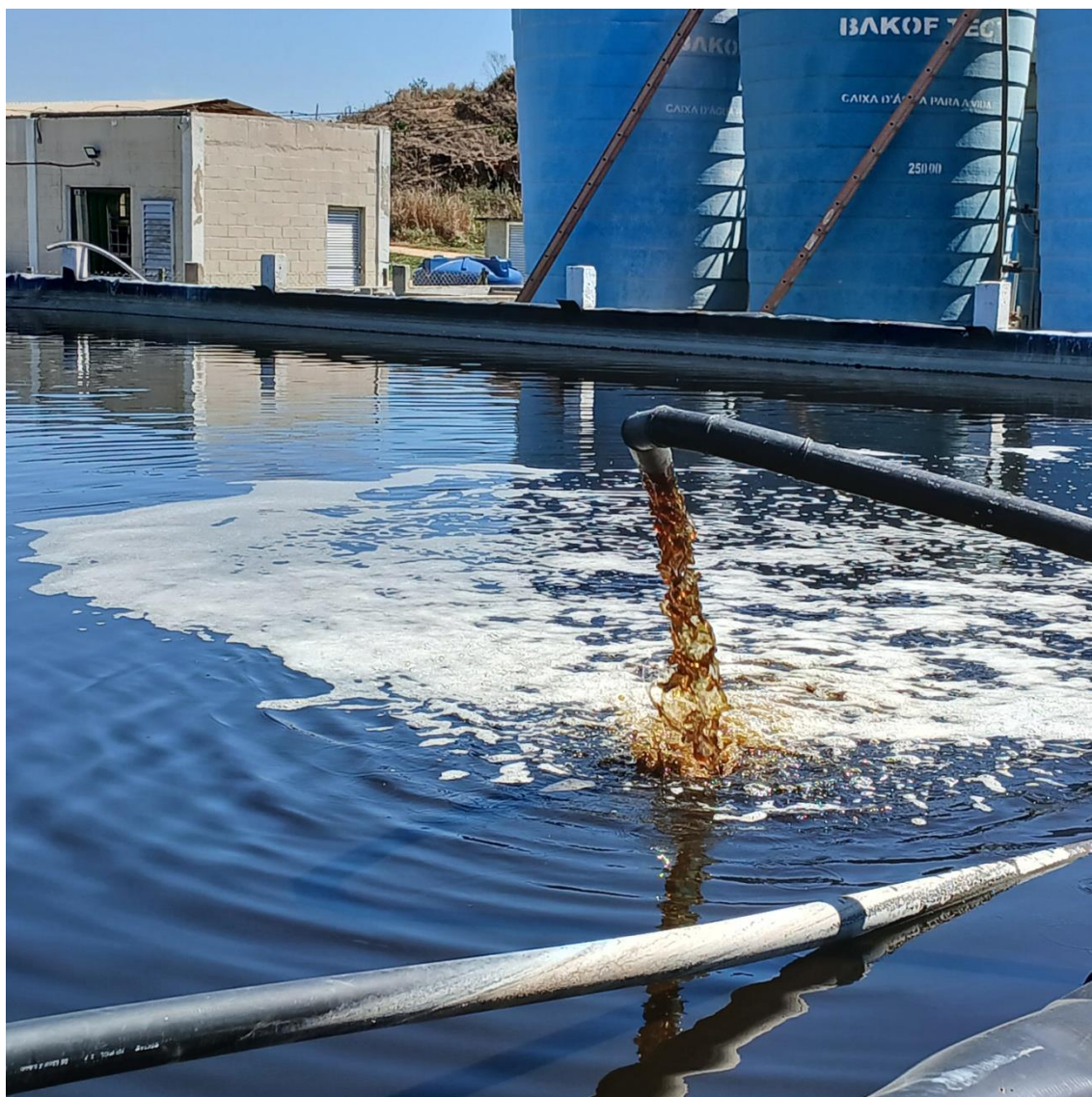
Figura 14: Lagoa secundária de recebimento de chorume
