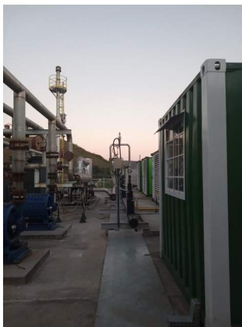
Figura 24: Estação de biogás
