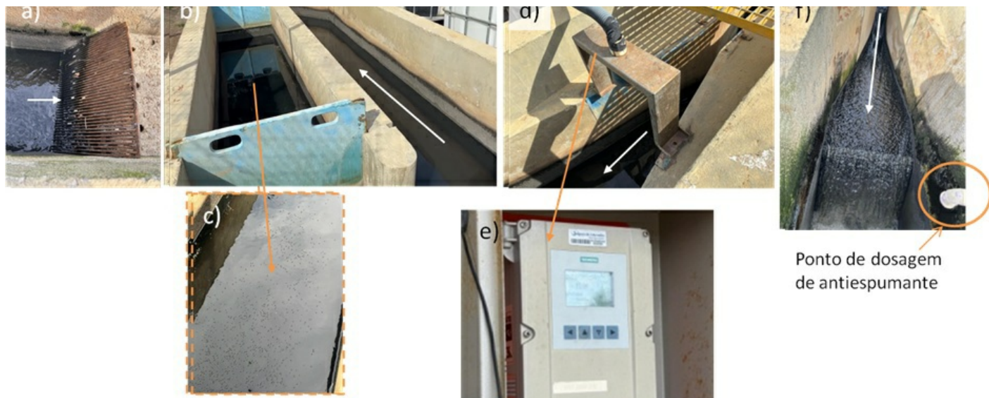
Foto 7 – Estruturas do tratamento preliminar (a- gradeamento, b - dois canais desarenadores, estando um - c - estagnado, com proliferação de insetos, d- calha Parshall com sensor de vazão, e - vazão instantânea: 19,84 l/s/ totalizador: 79432094, e f - saída com ponto para adição de antiespumante
