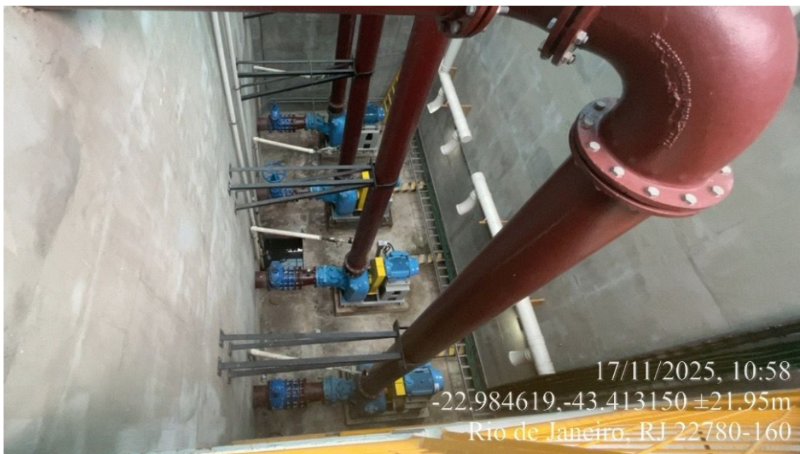
Foto 9 – Conjuntos motobombas
