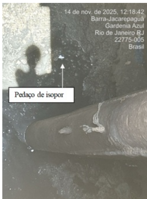
Foto 27 – Interior da caixa de chegada do esgoto
