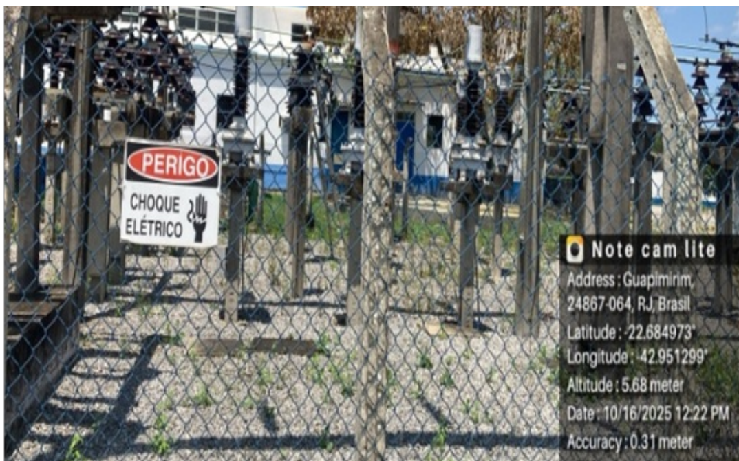
Foto 7 - Desligamento da subestação de Imunana para reaperto geral dos conectores e substituição de parafusos
