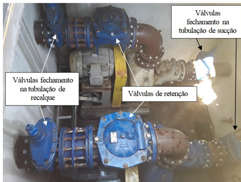
Foto 19 – Poço das motobombas com dois dos três grupos
