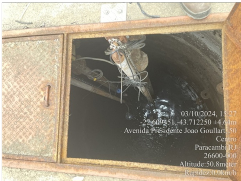
Foto 03 – Poço de sucção das bombas submersas e gradeamento
