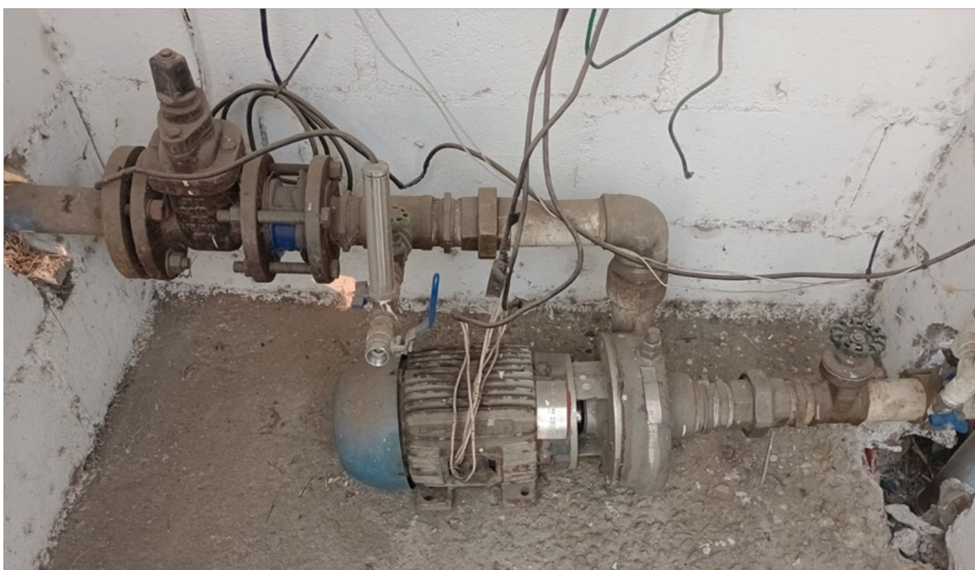
Foto 4 – Tubulação de retaguarda e recalque
