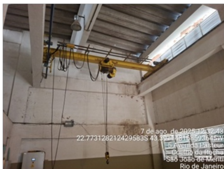
Foto 8 – Ponte rolante
