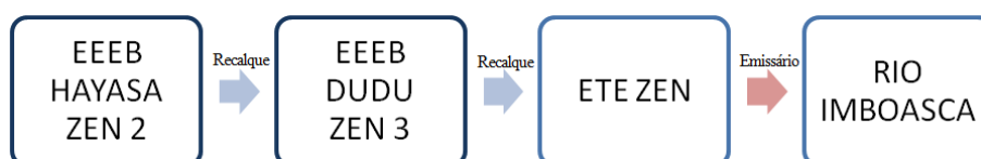
Foto 06 - Fluxograma das Estações Elevatórias do Distrito ZEN
