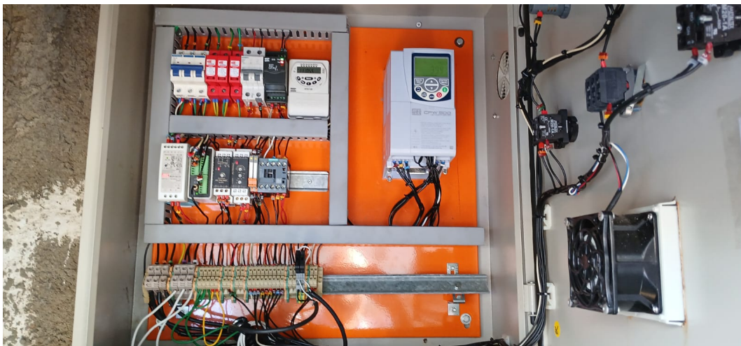
Foto 3 – Interior do painel de automação com inversor de frequência
