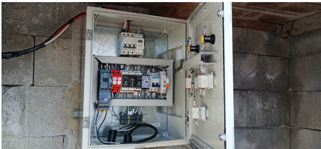
Foto 3 – Interior do painel de automação
