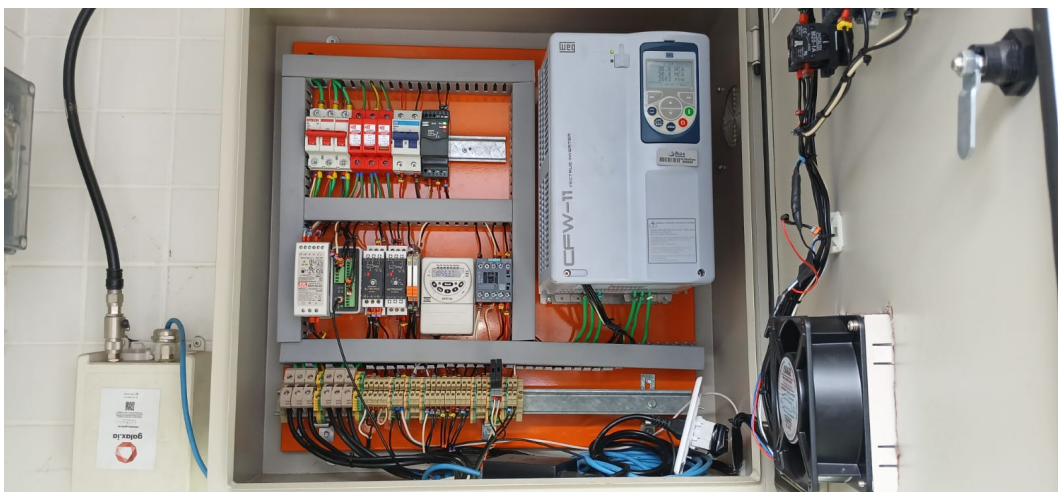
Foto 4 – Visualização do interior do painel de automação
