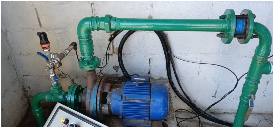
Foto 2 - Visualização dos equipamentos do conjunto motobomba
