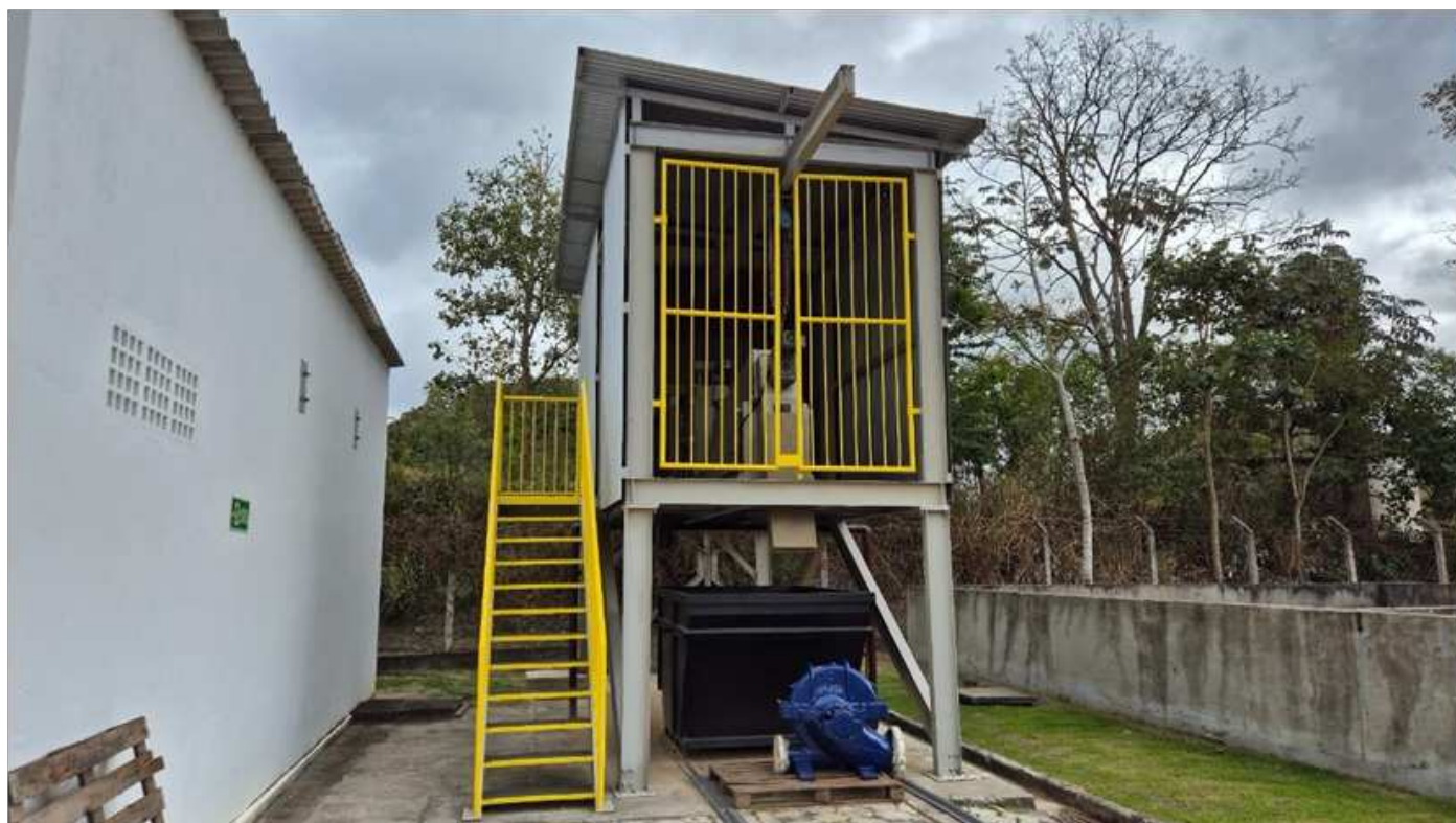
Foto 19 Local onde se encontra o preparador de polímeros e a centrífuga para desidratação do lodo
