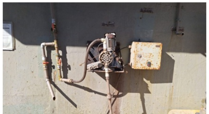
Fotos 12 e 13 – Reservatórios de PAC com baía de contenção ; Dosador de PAC necessitando de manutenção.
